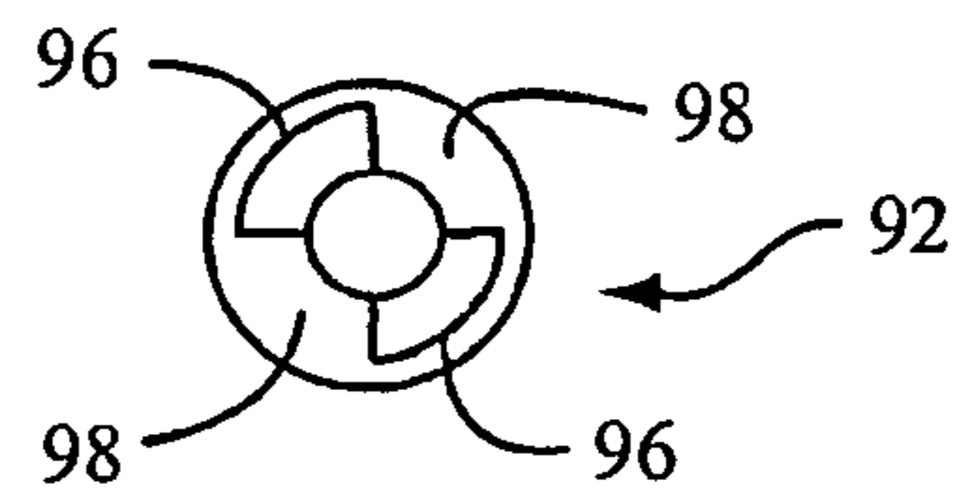
FIG. 11C
