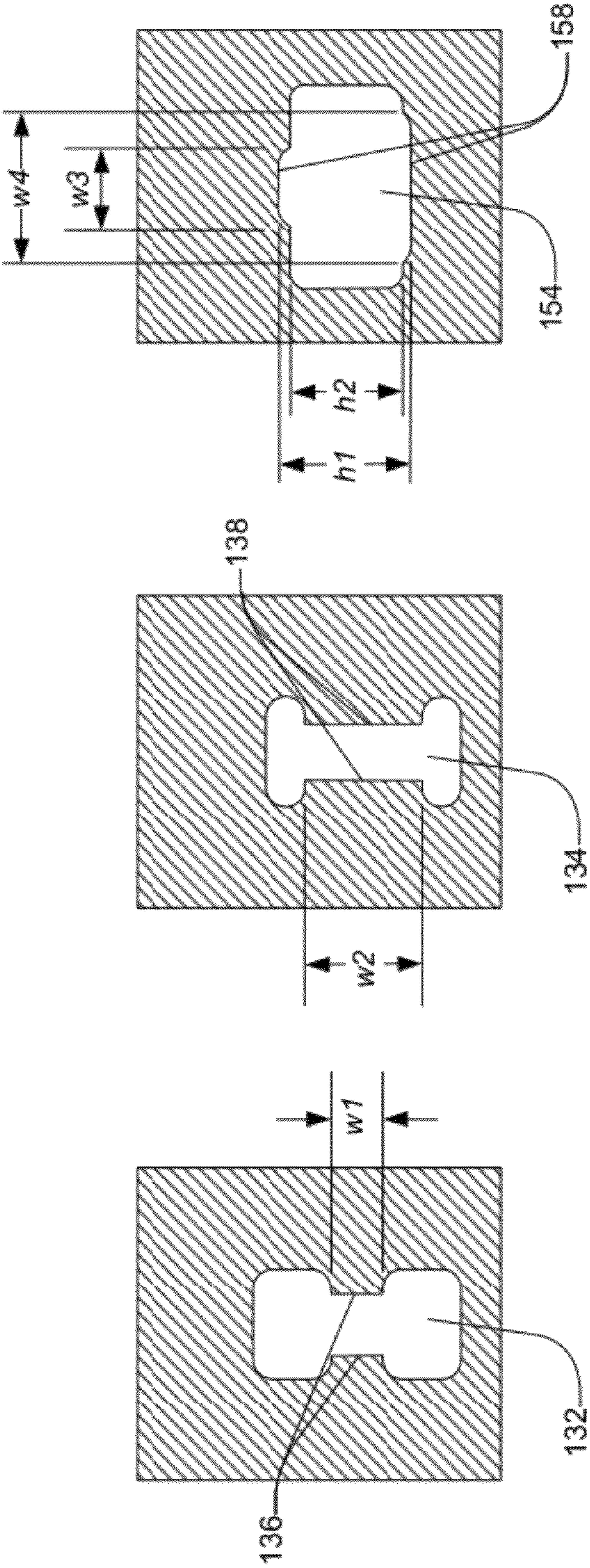
Section D-D
