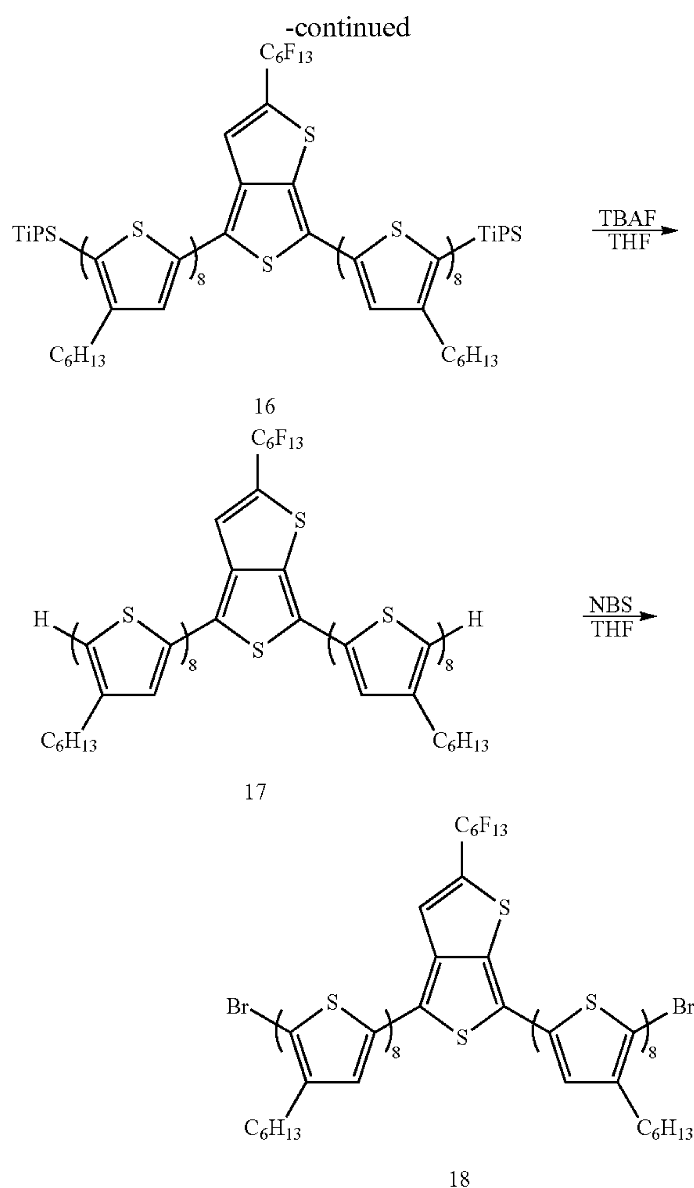
Oligomer (18)
