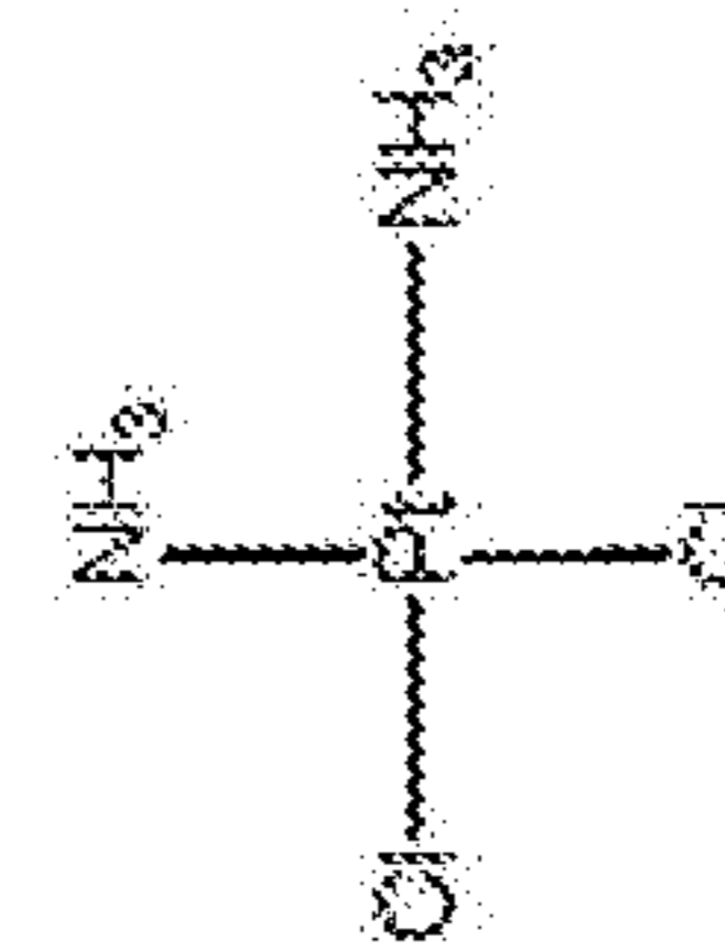
cisplatin cis-DDP
