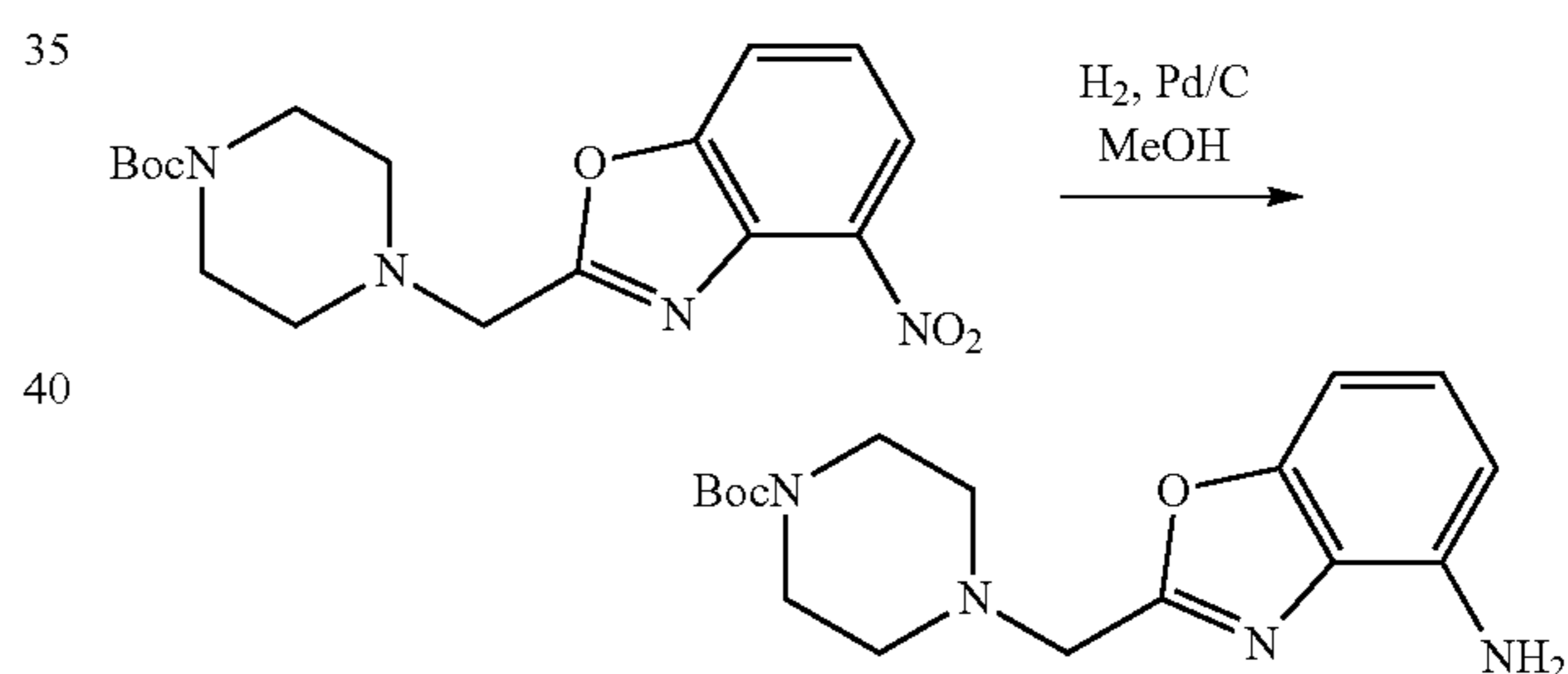
tert-Butyl 4-((4-aminobenzo[d]oxazol-2-yl)methyl)piperazine-1-carboxylate
