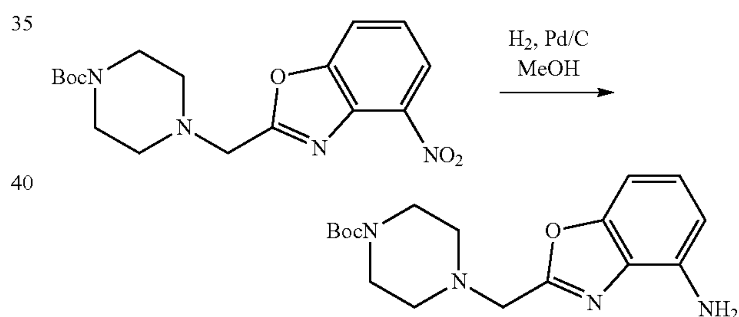
tert-Butyl 4-((4-aminobenzo[d]oxazol-2-yl)methyl)piperazine-1-carboxylate
