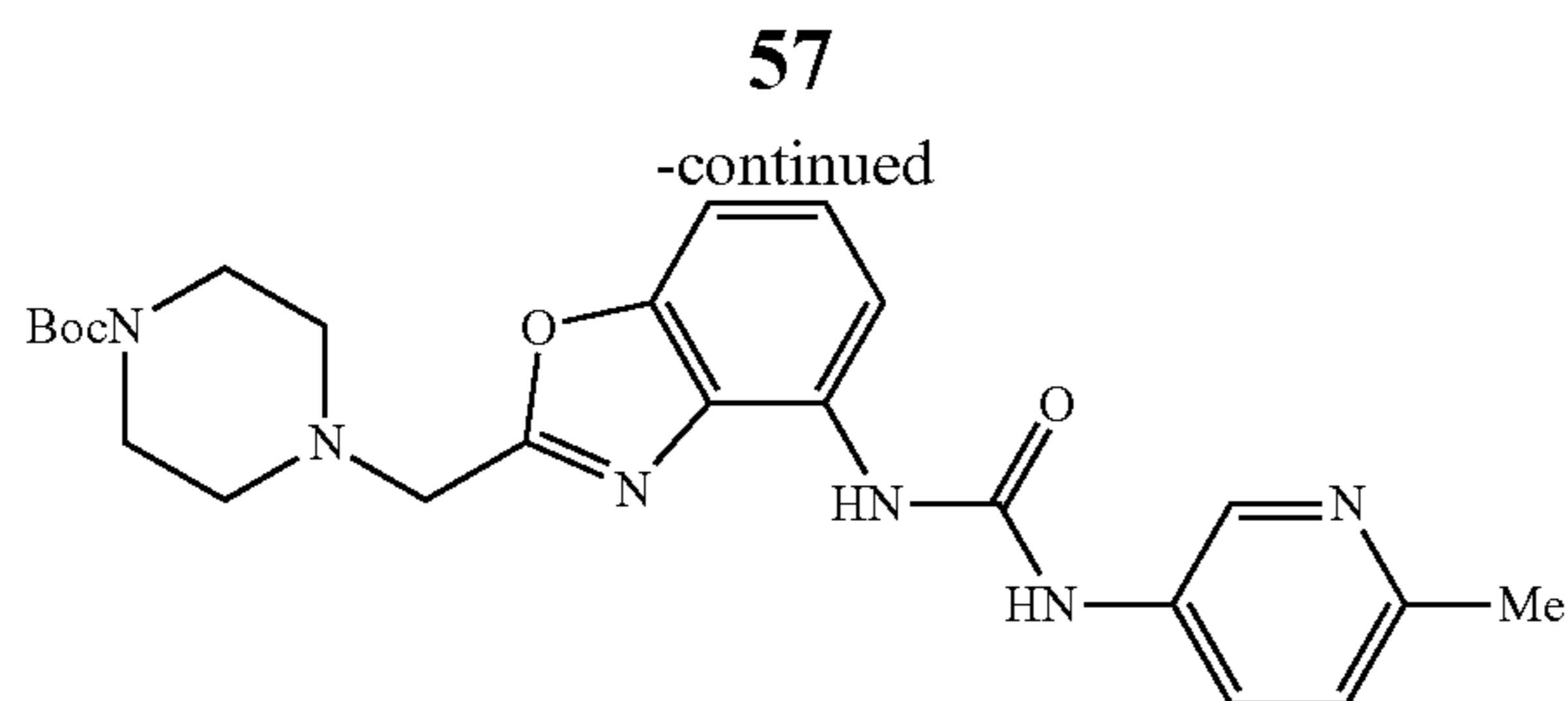
tert-Butyl 4-((4-(3-(6-methylpyridin-3-yl)ureido)benzo[d]oxazol-2-yl)methyl)piperazine-1-carboxylate
