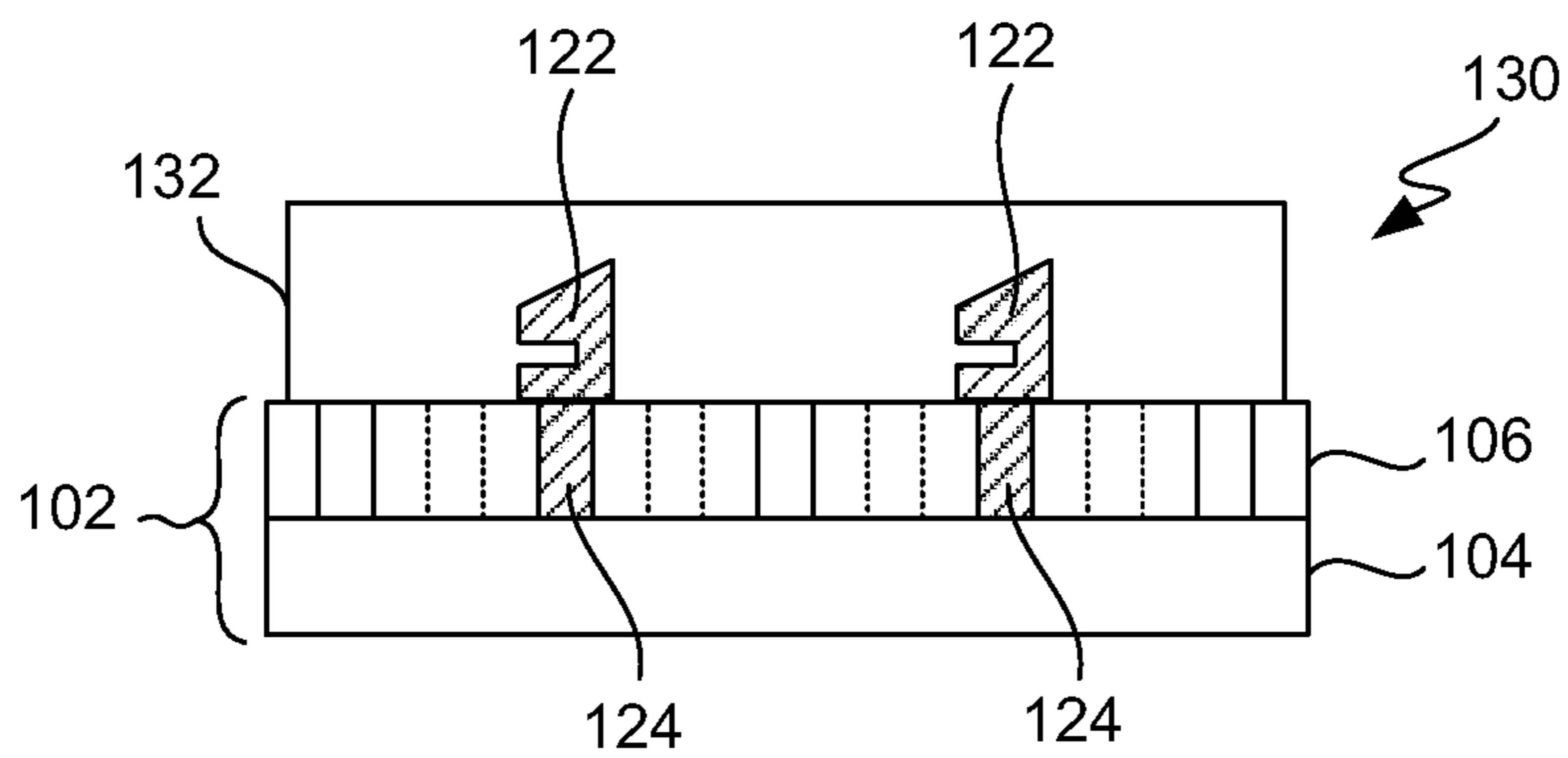
FIG. 1C
