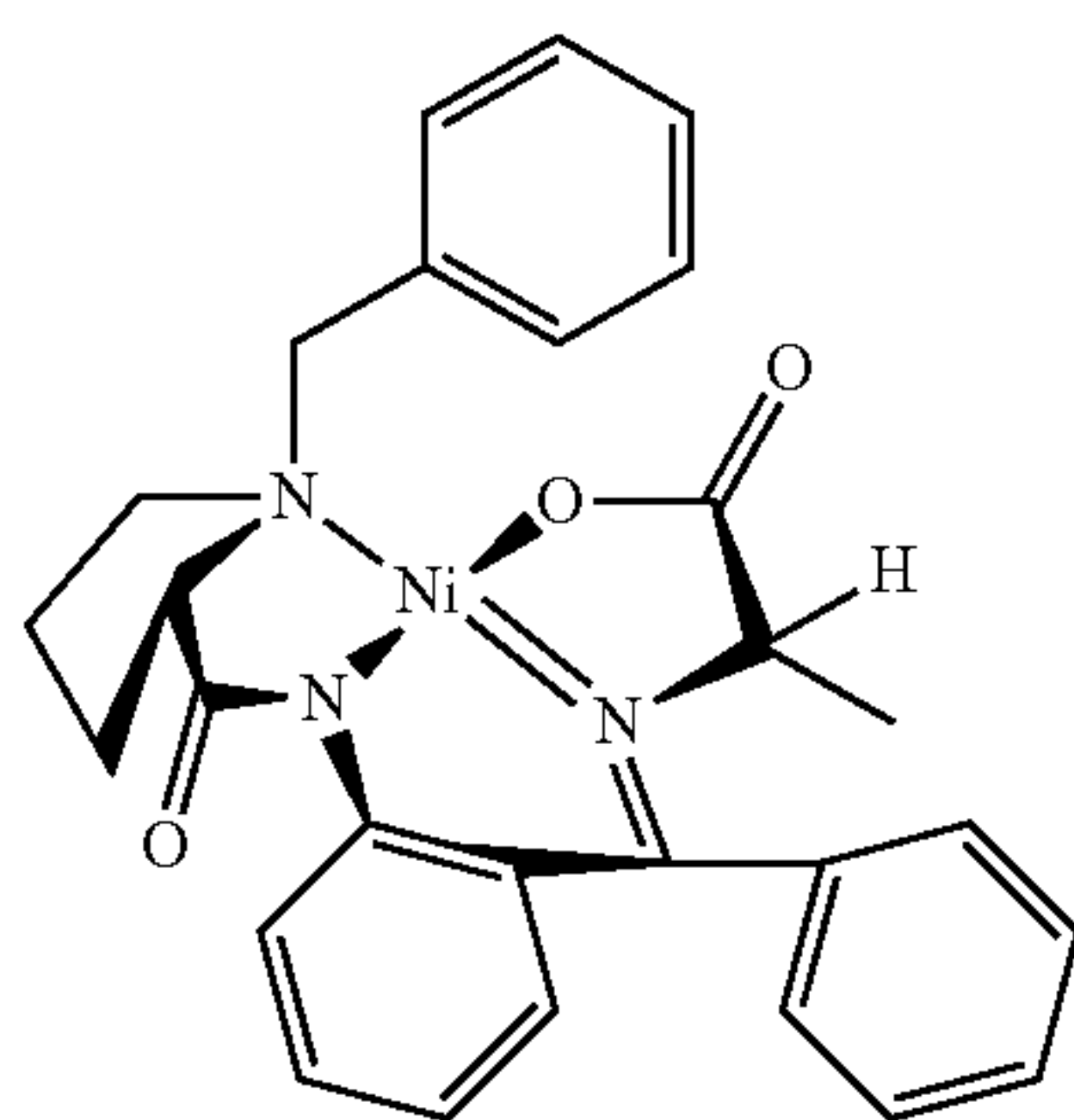
S-Ala-Ni-BPB
