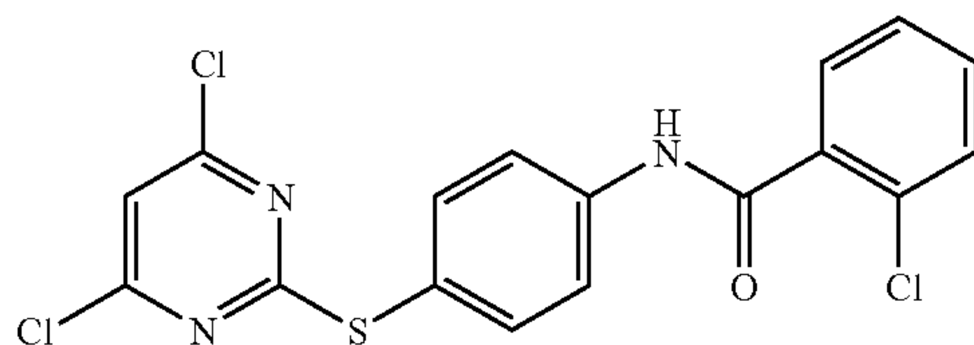
2-Chloro-N-[4-(4,6-dichloro-pyrimidin-2-ylsulfanyl)-phenyl]-benzamide
