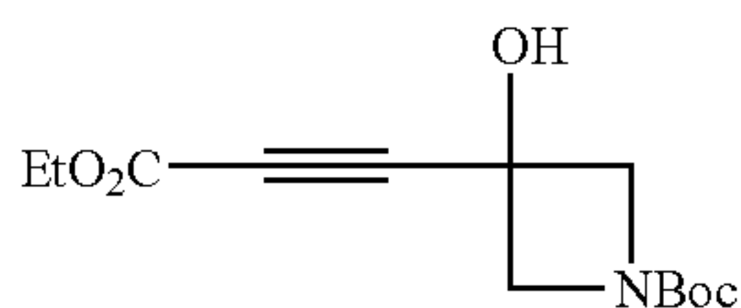
tert-butyl 3-(2-(ethoxycarbonyl)ethynyl)-3-hydroxyazetidine-1-carboxylate
