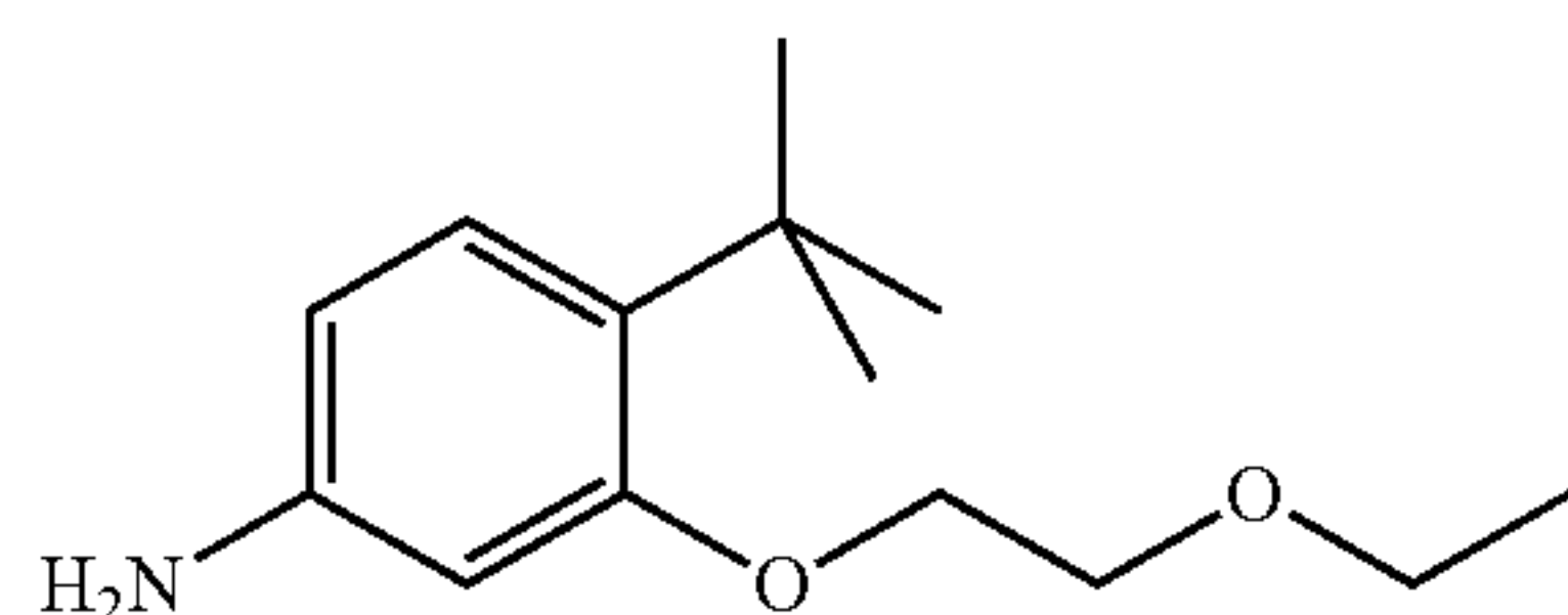
C-3; 3-(2-Ethoxyethoxy)-4-tert-butylbenzenamine
