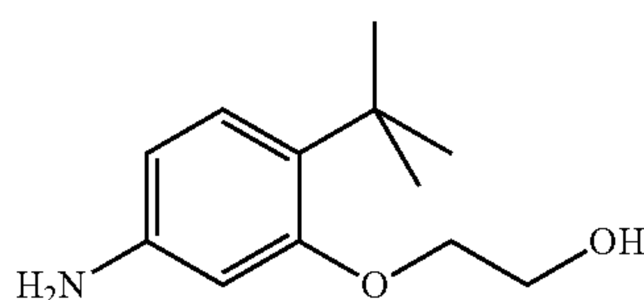
C-4; 2-(2-tert-Butyl-5-aminophenoxy)ethanol
