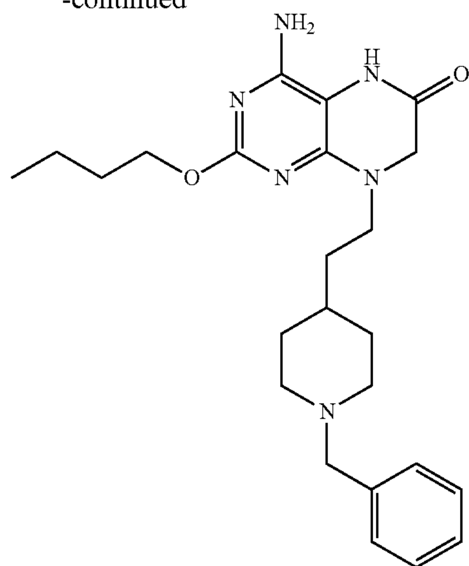
Example 108
