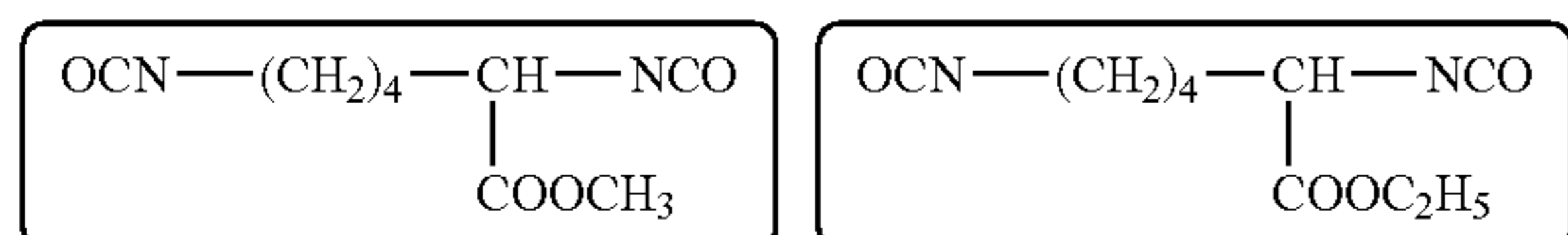
MLDI
