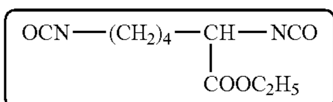
ELDI
