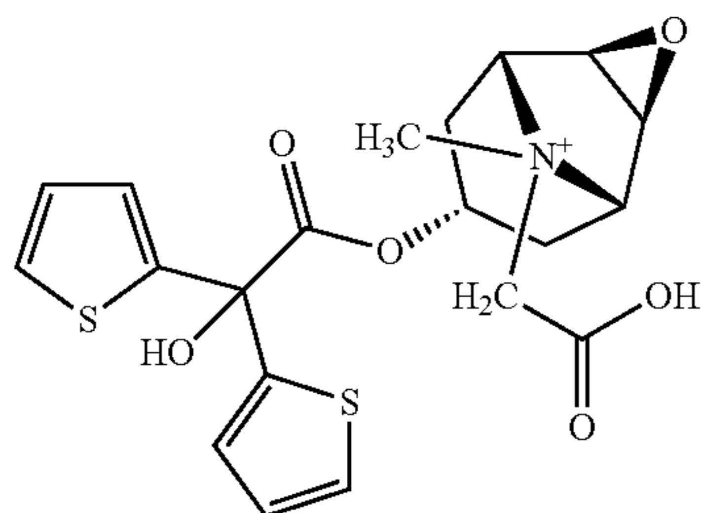
Tiotropium zwitterion
