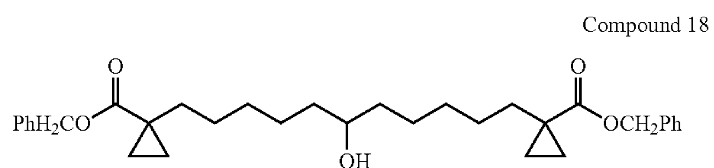
1,11-Bis-(1-benzyloxycarbonyl-cyclopropyl)-undecan-6-ol
