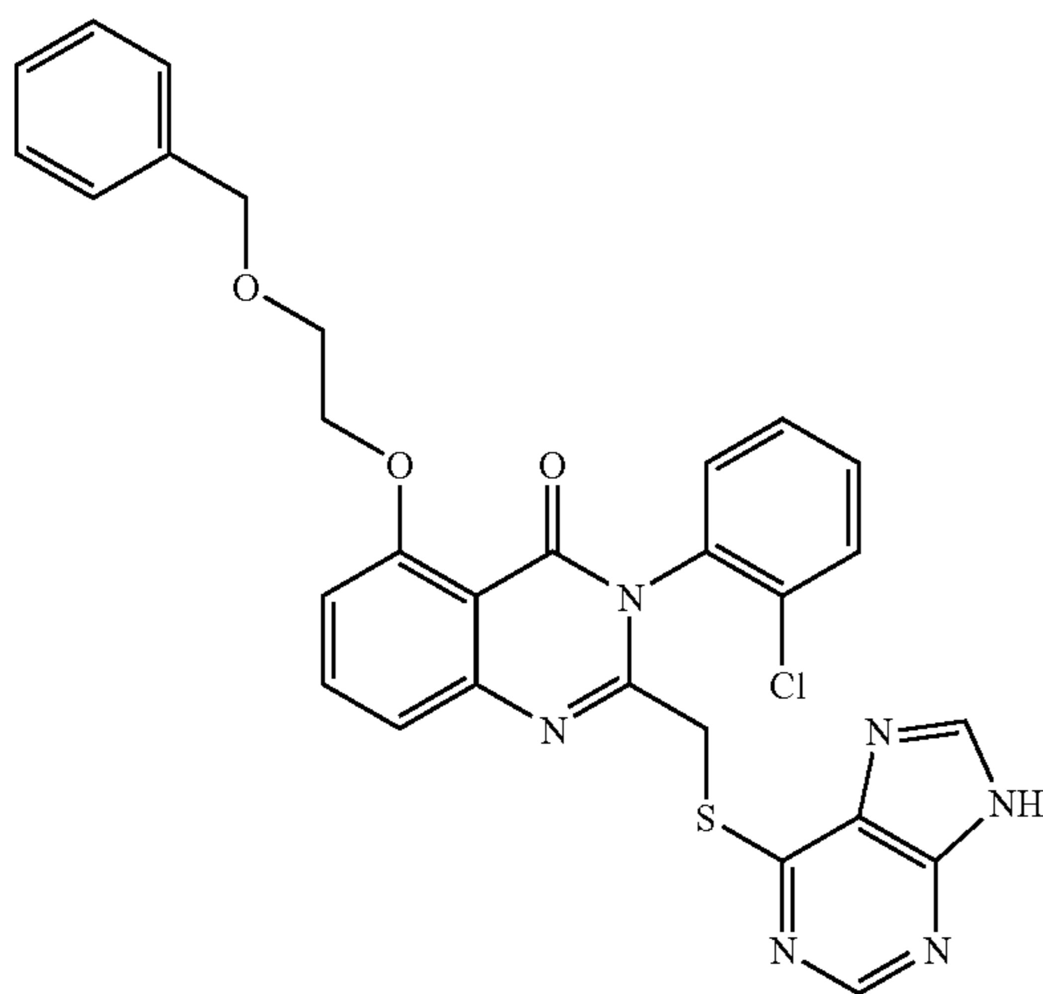
5-(2-Benzyloxyethoxy)-3-(2-chlorophenyl)-2-(9H-purin-6-ylsulfanylmethyl)-3H-quinazolin-4-one (D-078)
