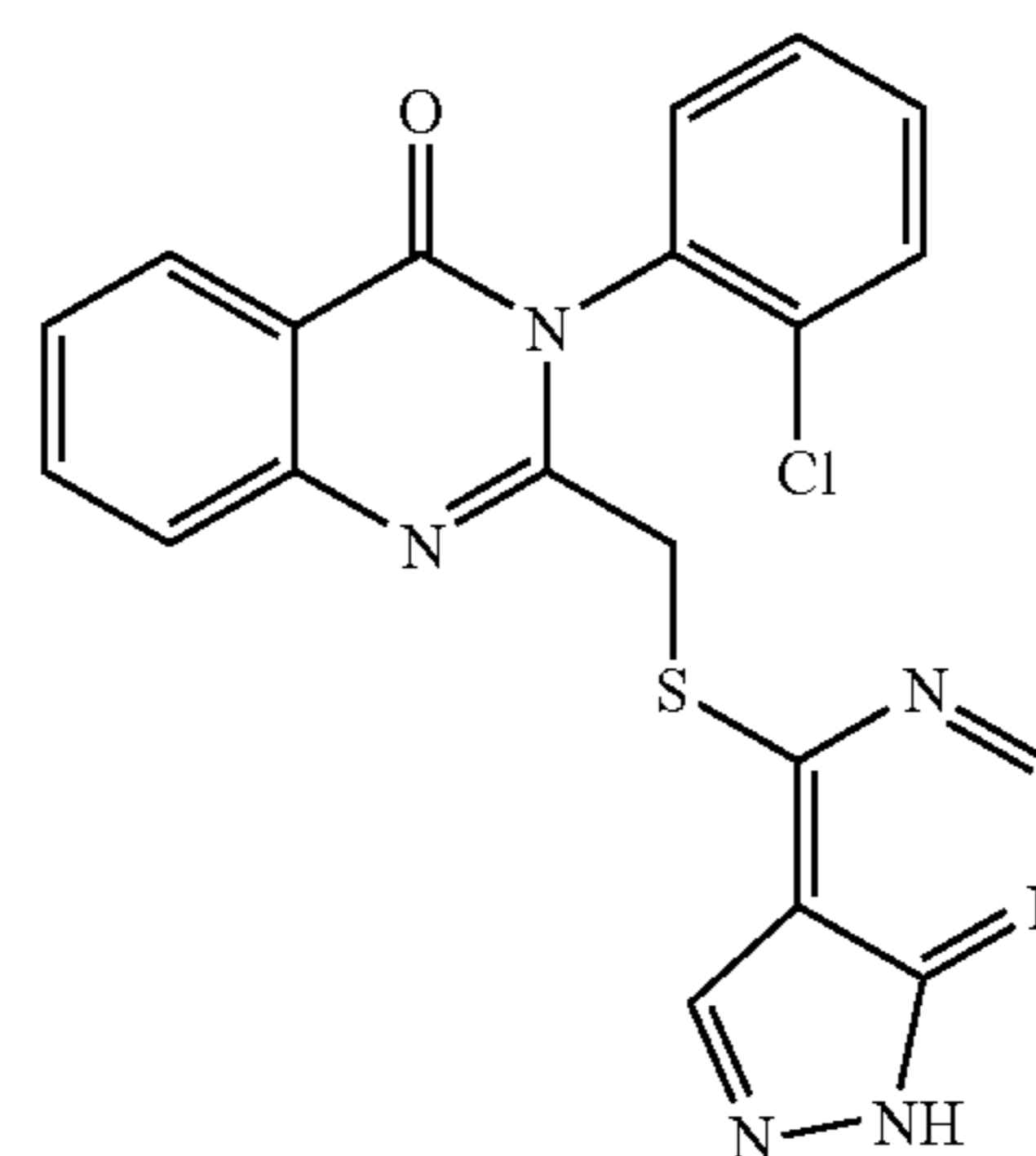
D-999
