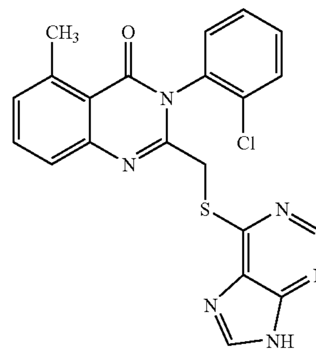
D-026
