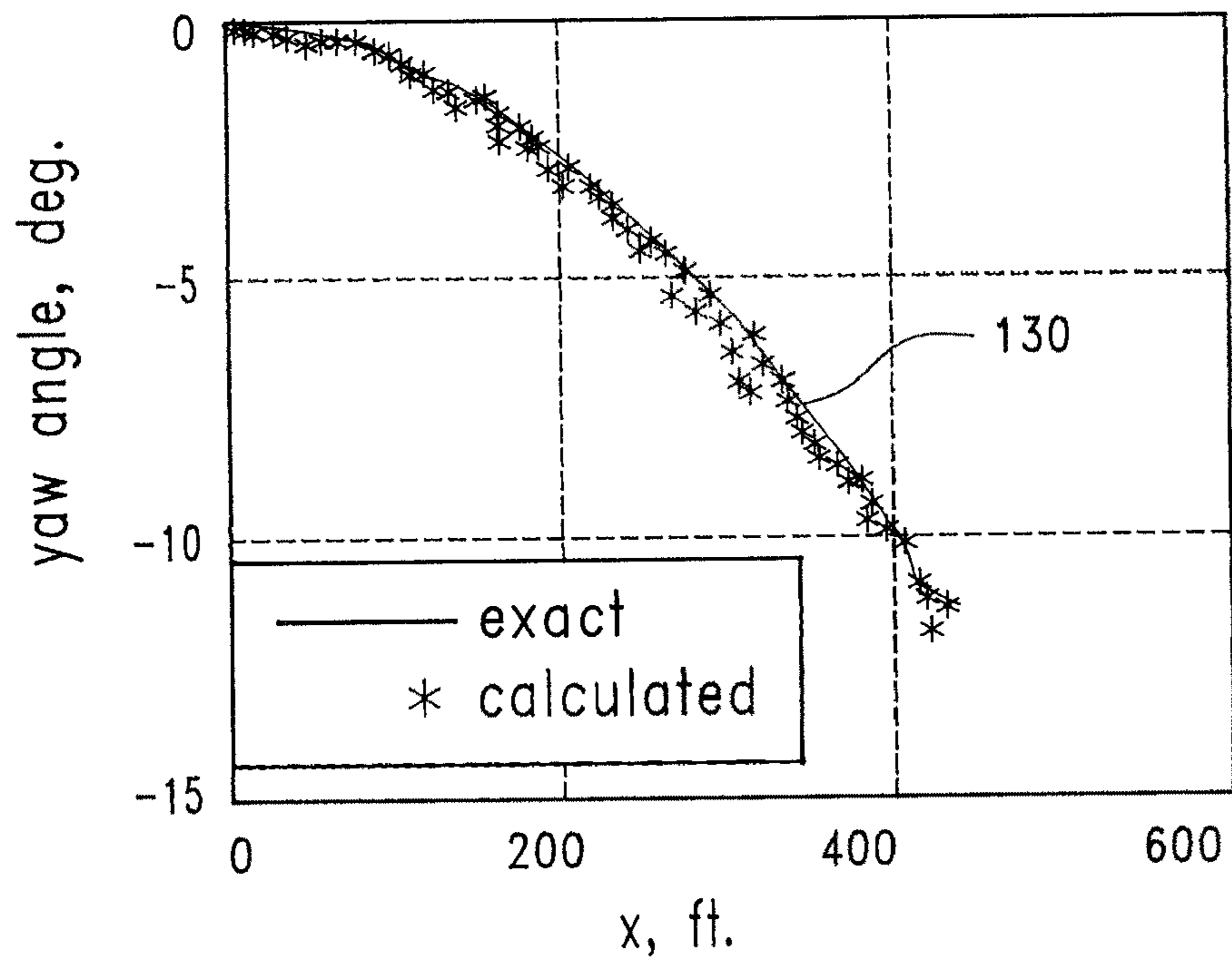
FIG. 7c
