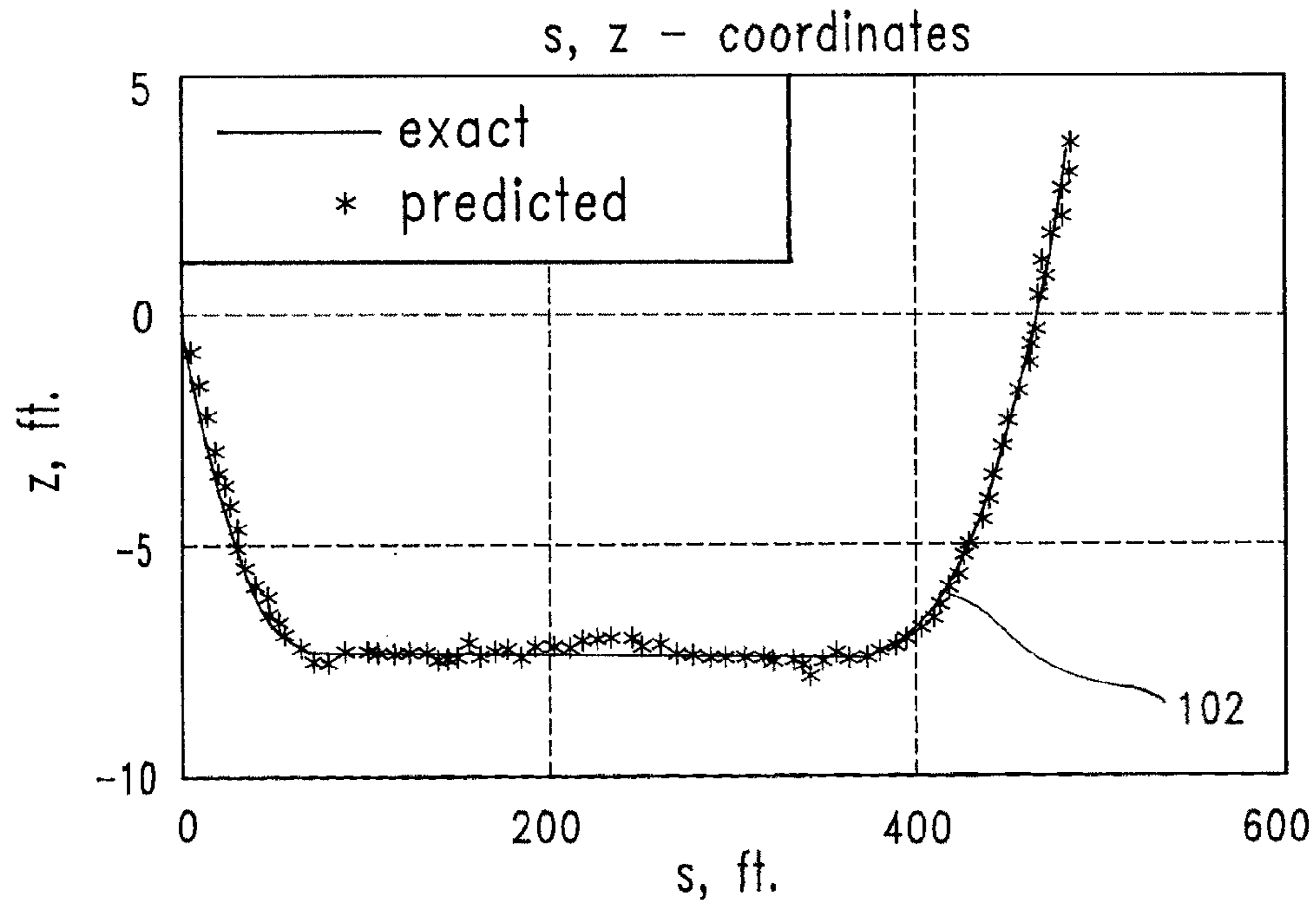
FIG. 5c
