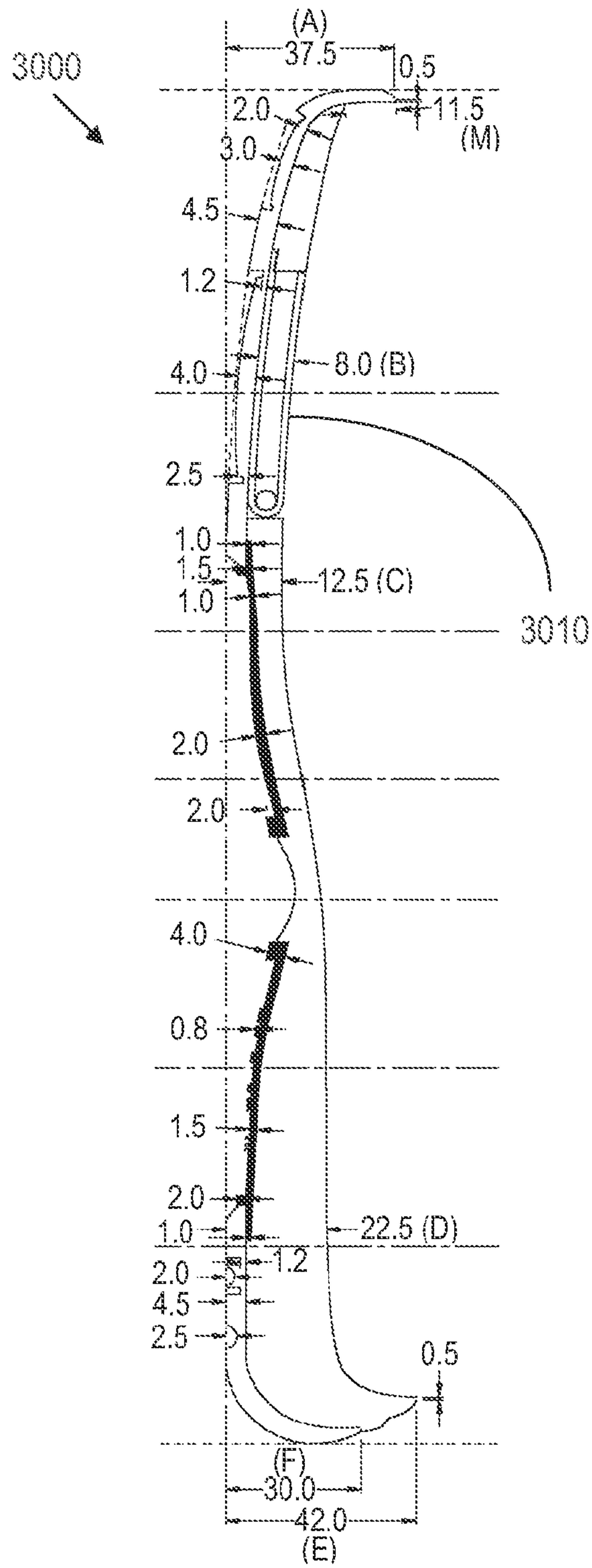
SECTION A-A'
