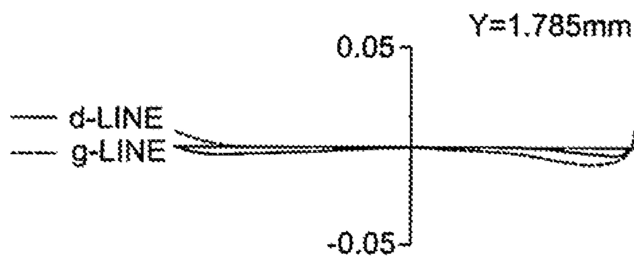
MERIDIONAL COMA (mm)
