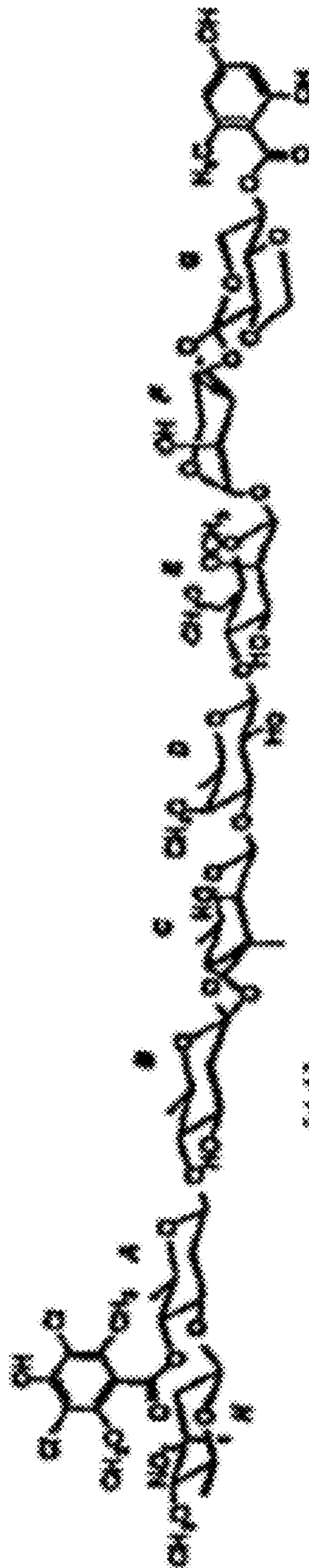
Staurosporine ( S. staurosporeus )
