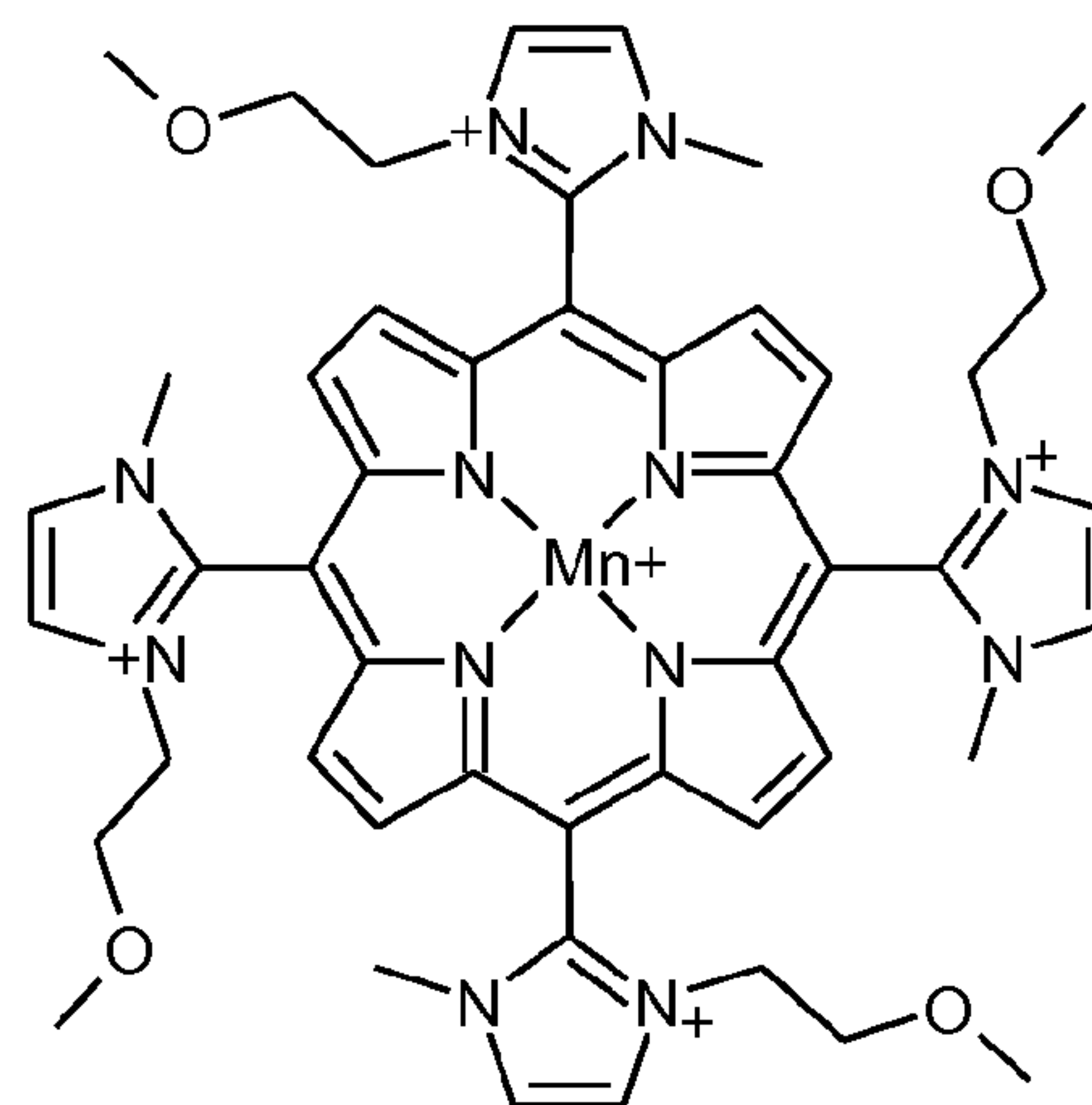
Mn III TM,MOE-2-ImP 5+
