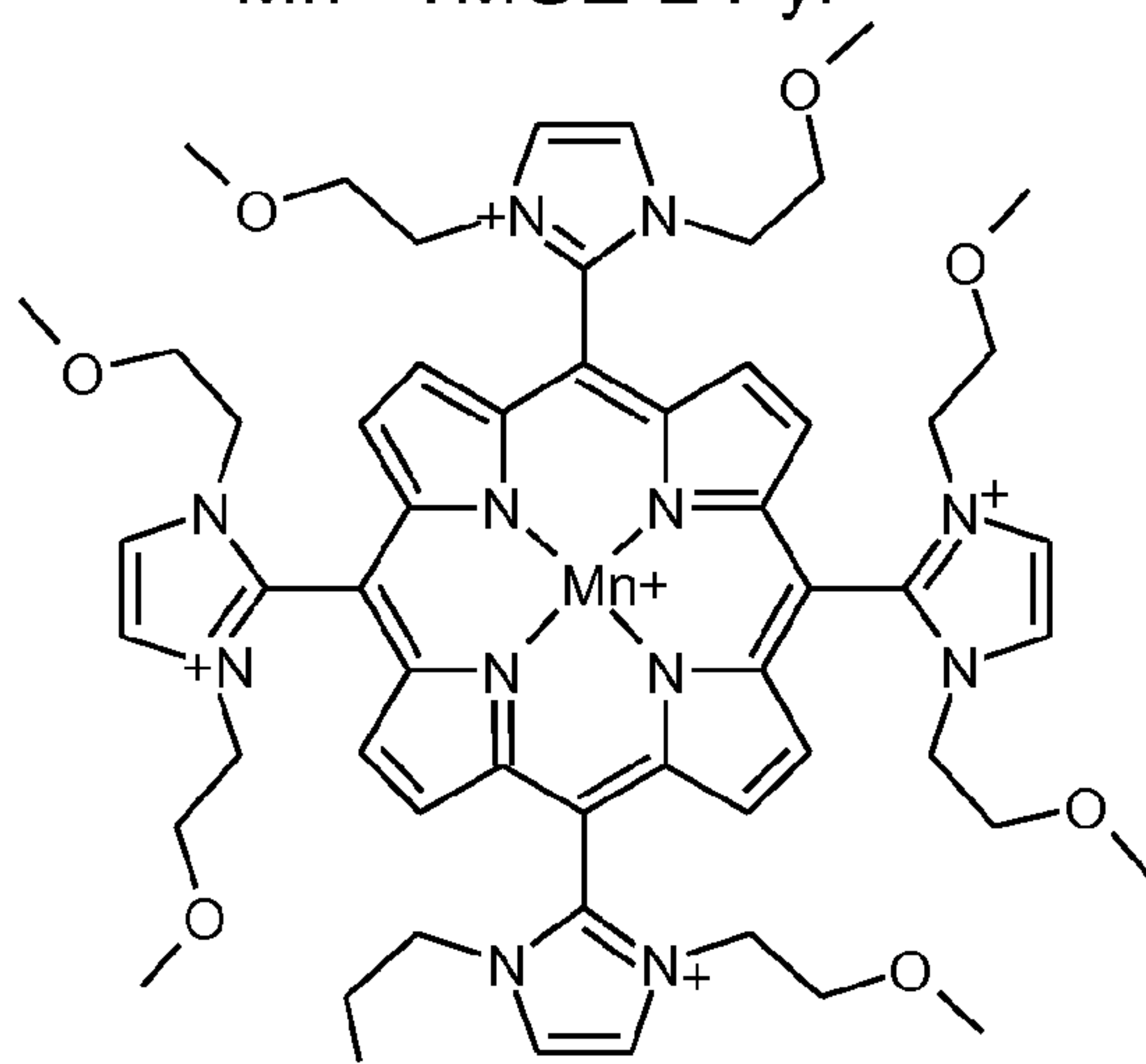
Mn III TMOE-2-PyP 5+
