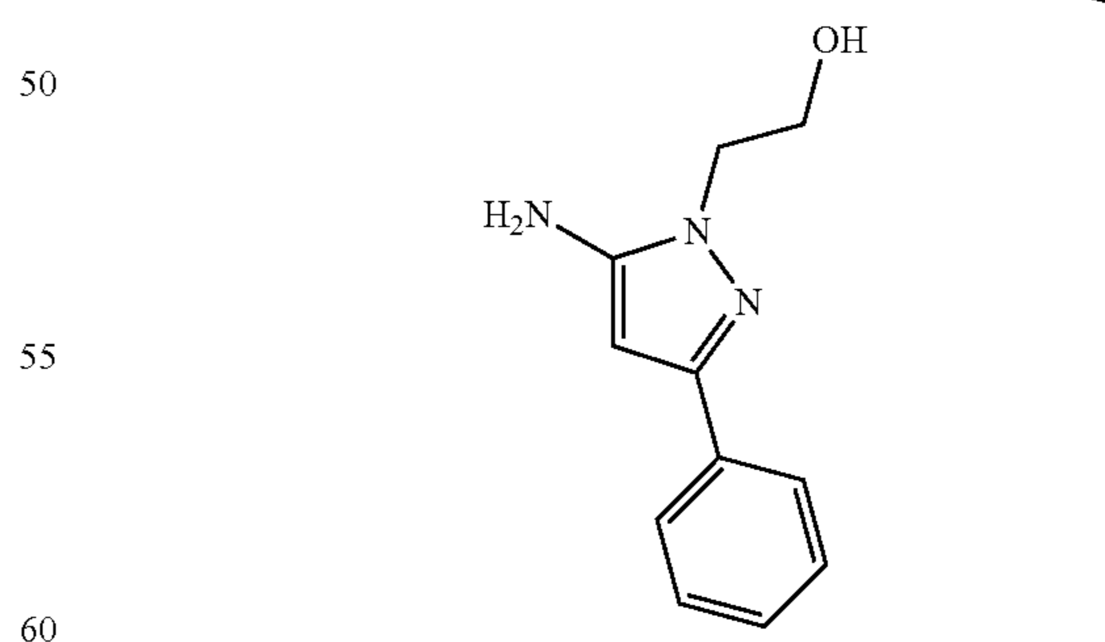
2-(5-Amino-3-phenyl-pyrazol-1-yl)-ethanol
