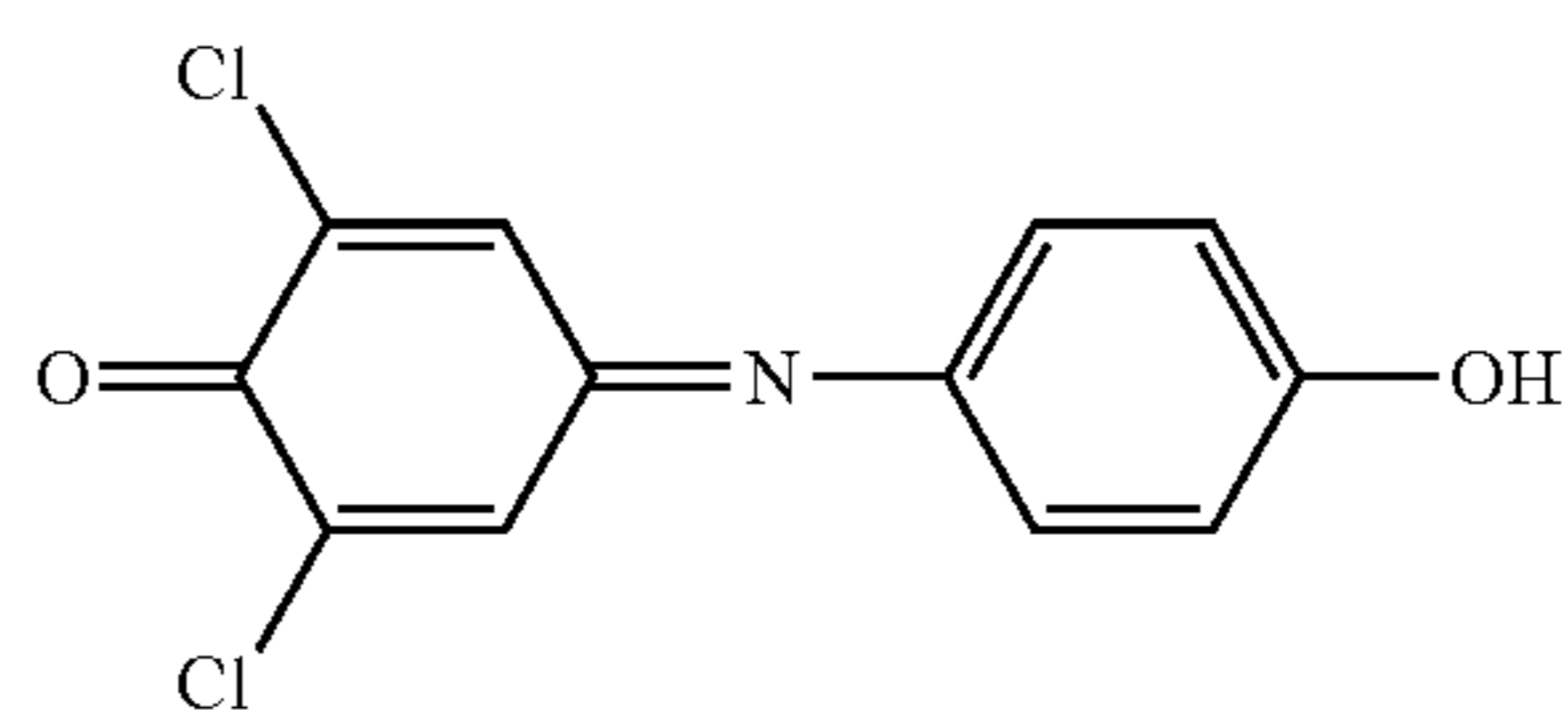
2,6-dichloro-indophenol ("DCI")
