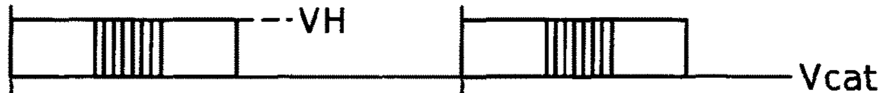
FIG. 32C DUTY40%
