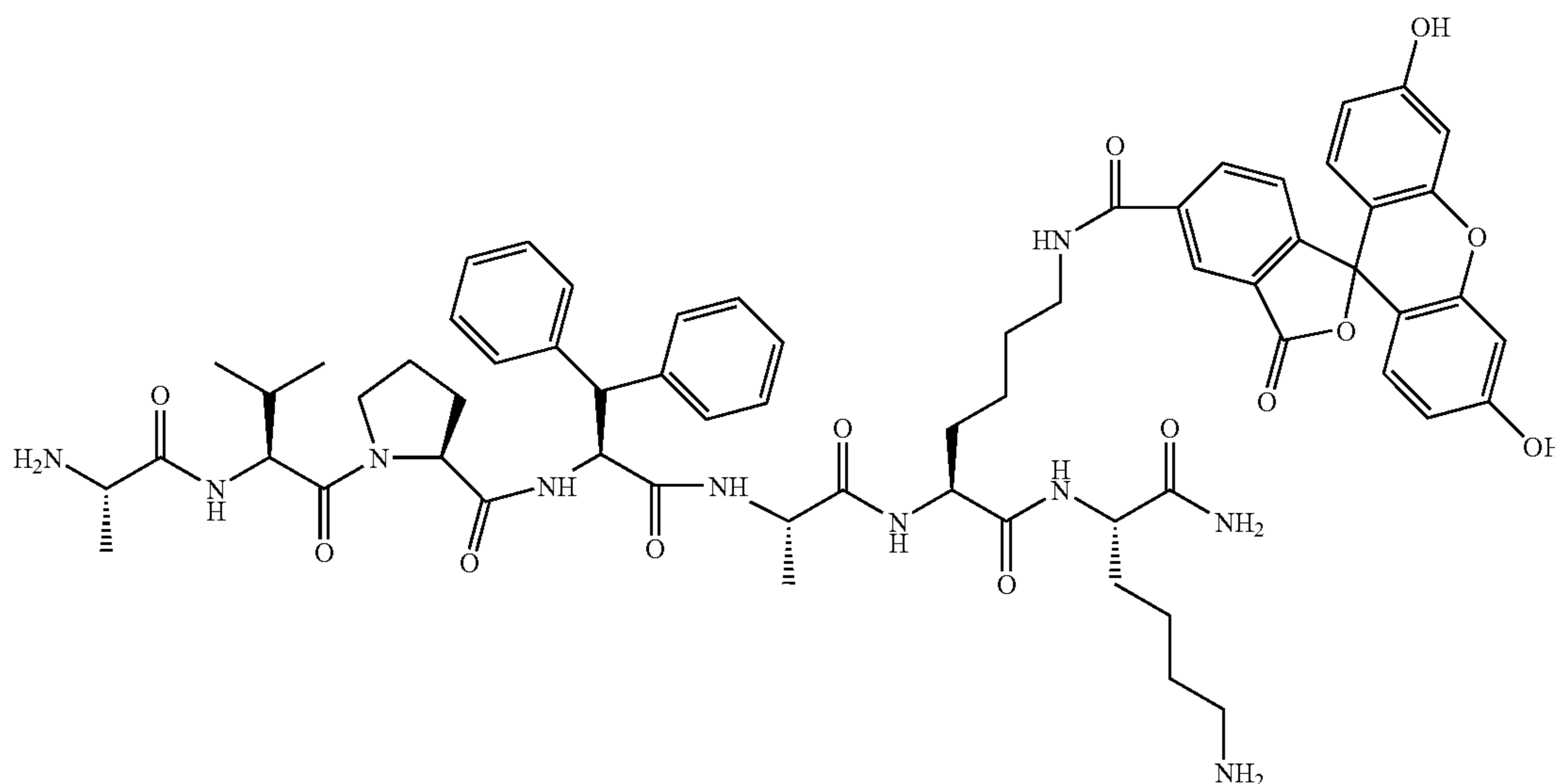
AVP-diPhe-FAM probe
