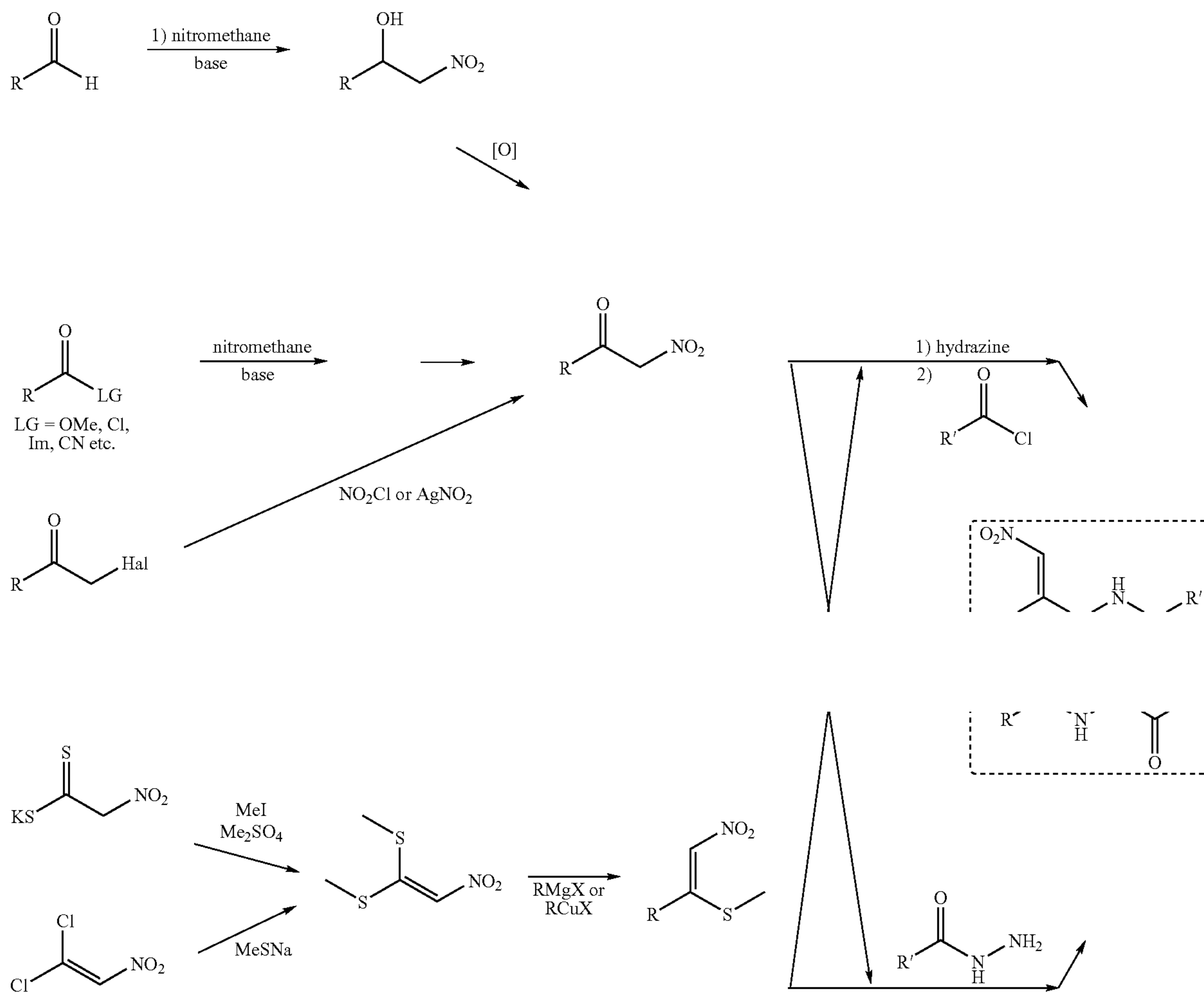
Scheme VI:
