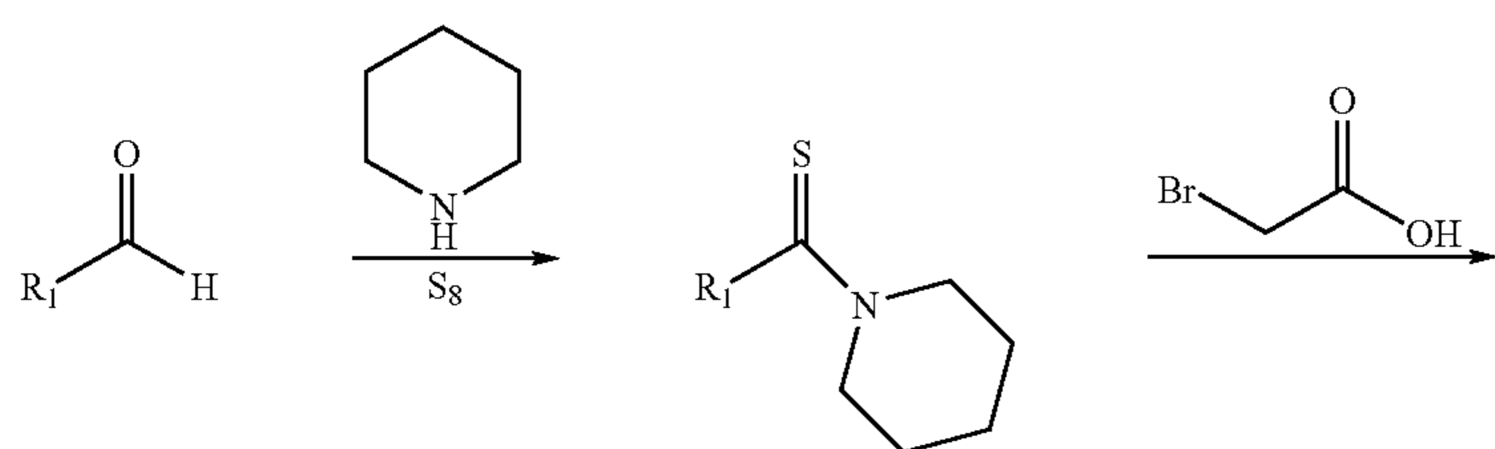
Scheme VII:
