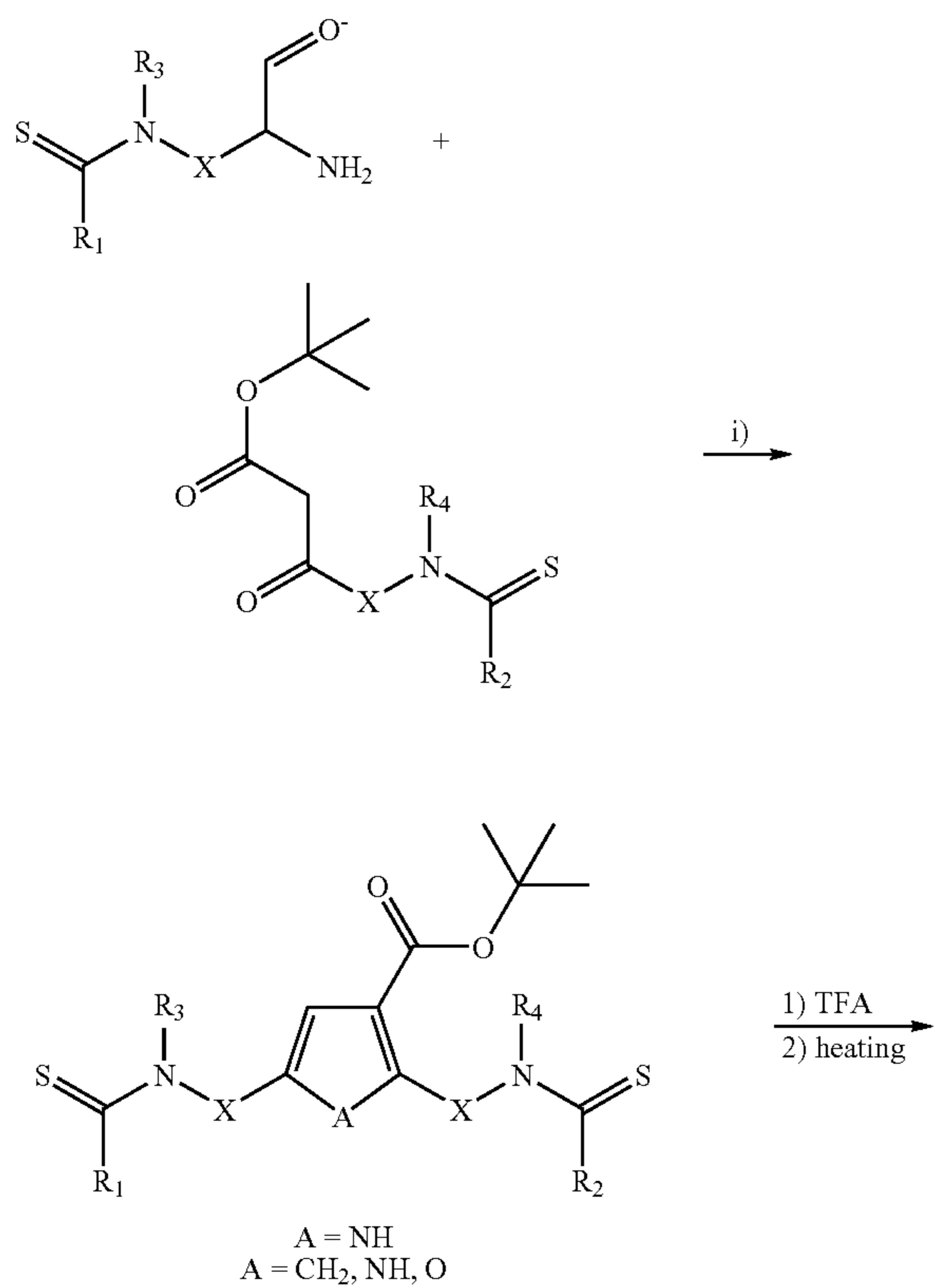
Scheme VIII:
