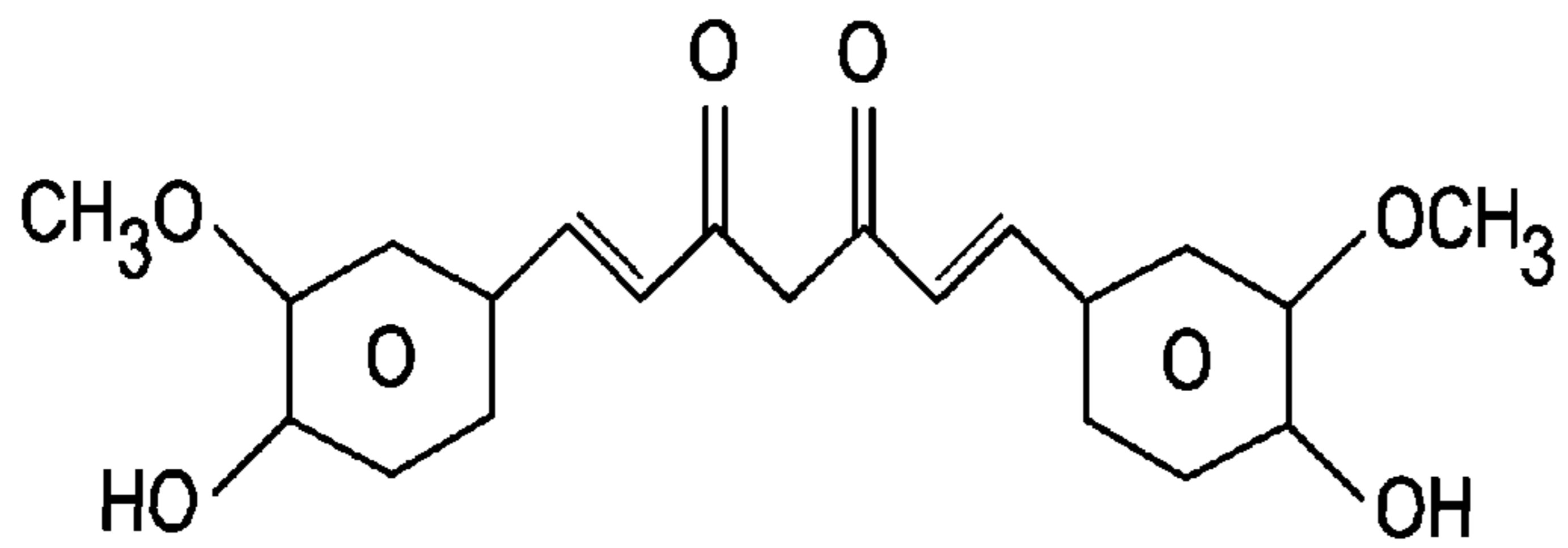
Curcumin
