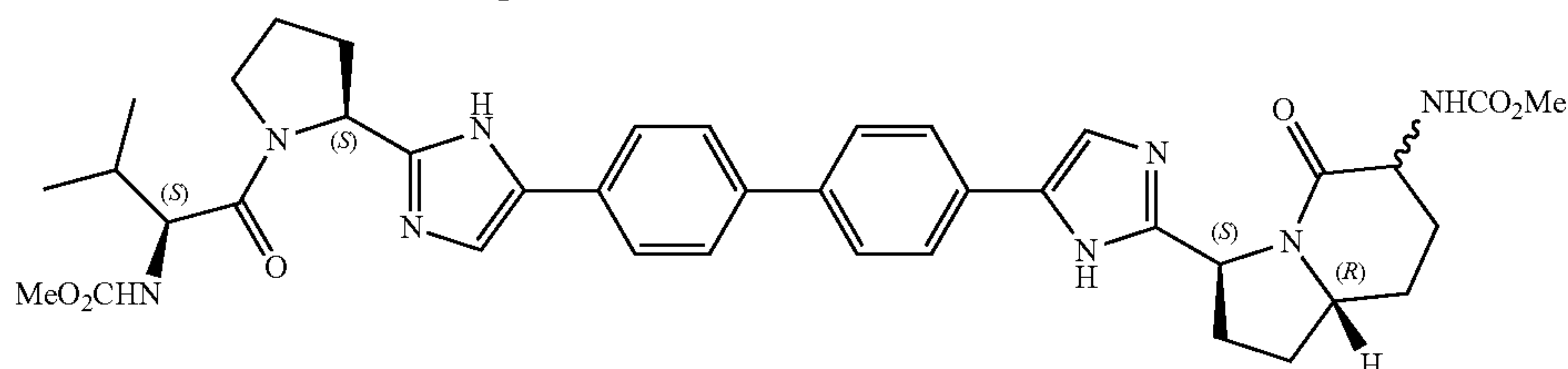
Example 371
