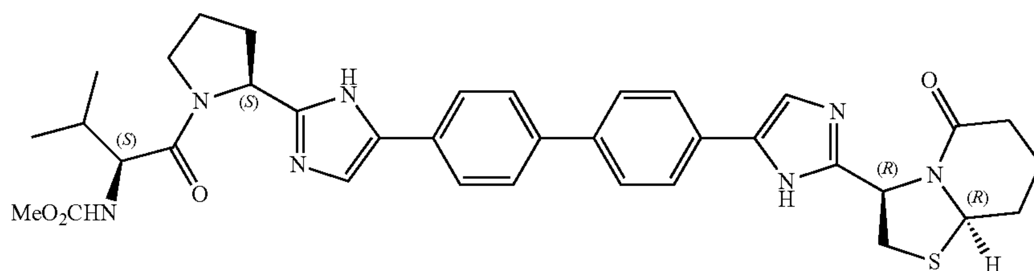
Example 372
