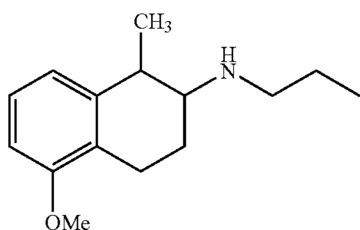
AJ76
