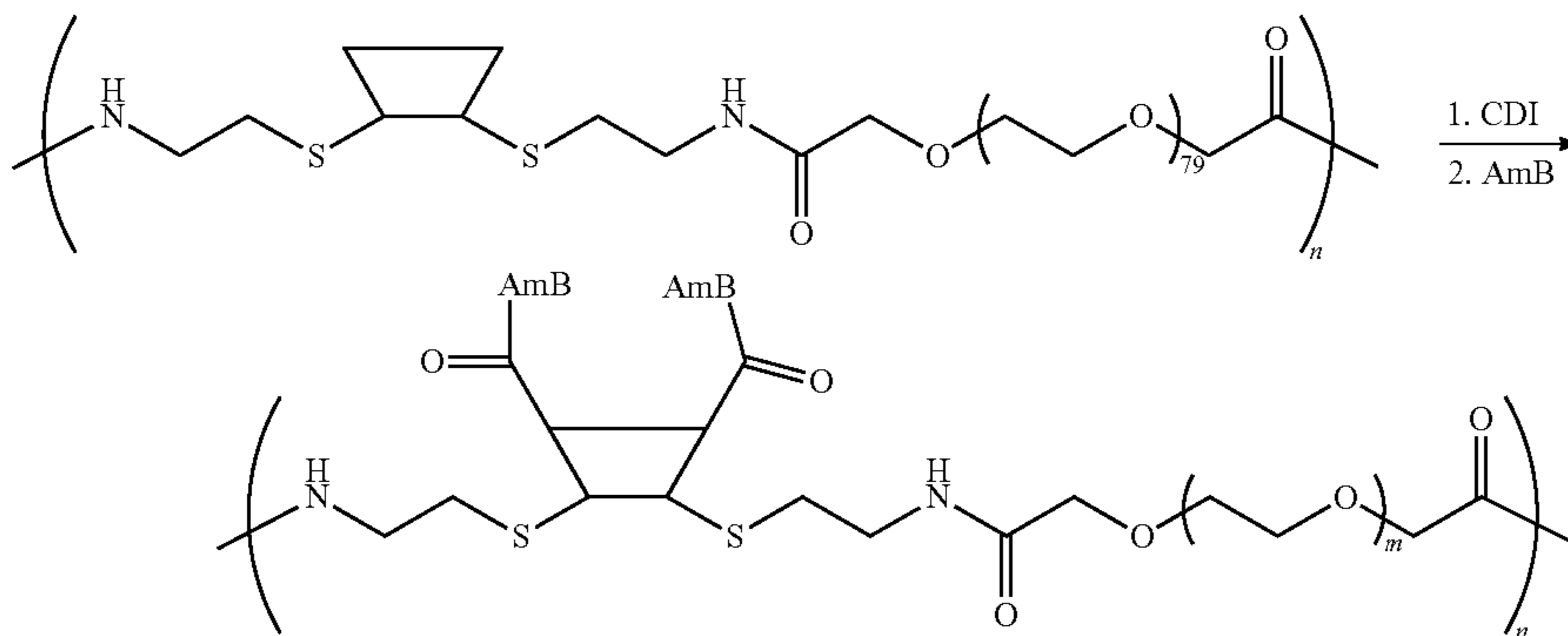
Scheme LII
