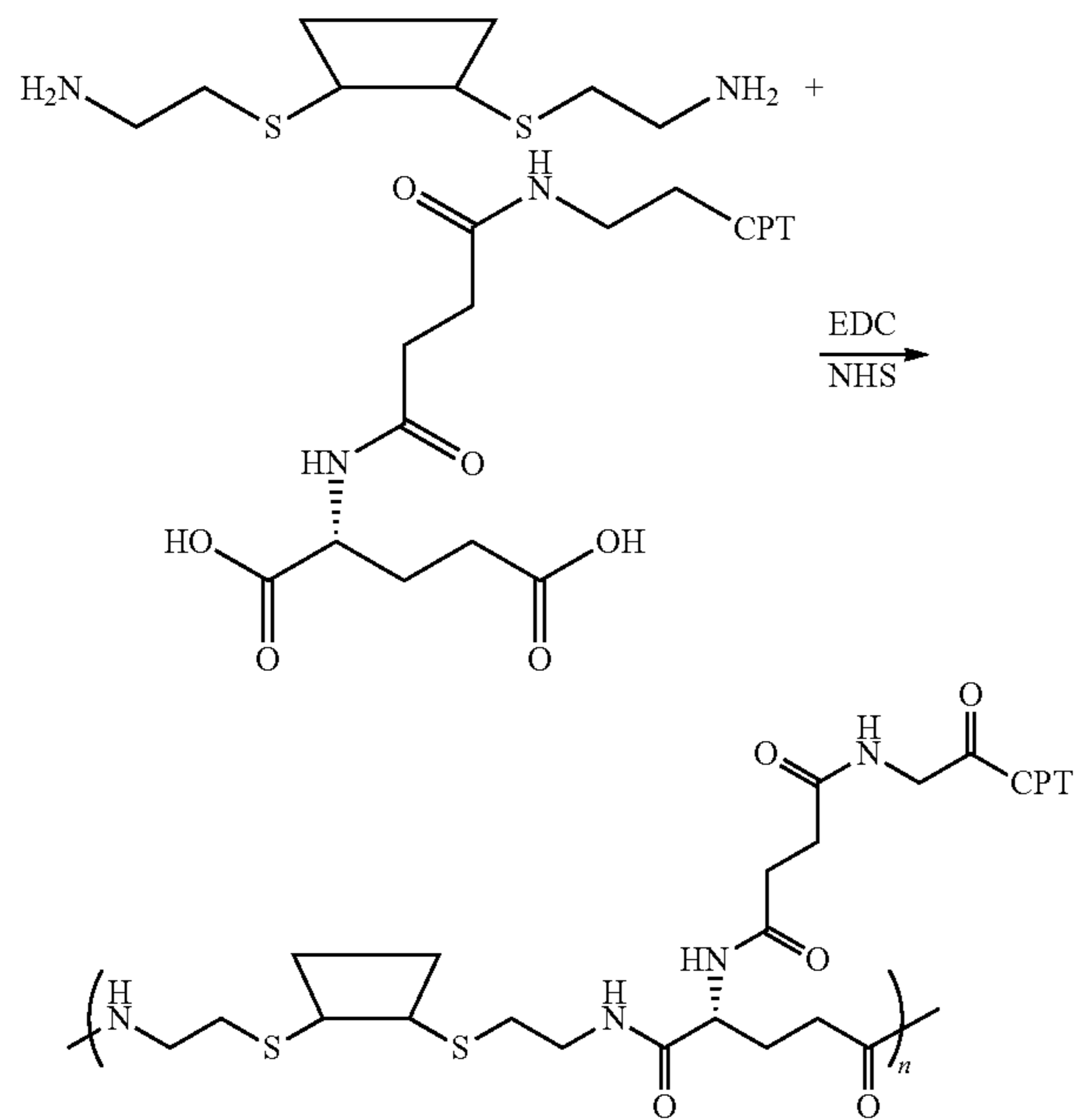
Scheme VI
