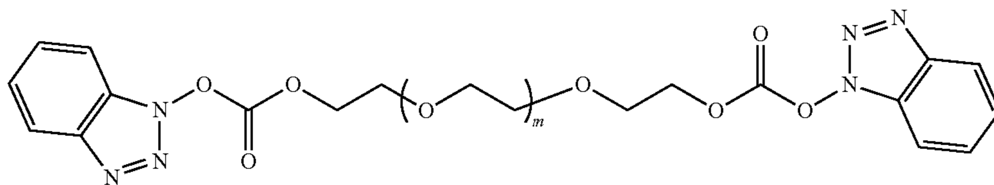
PEG—DiBTC (MW = 3400 Da)
