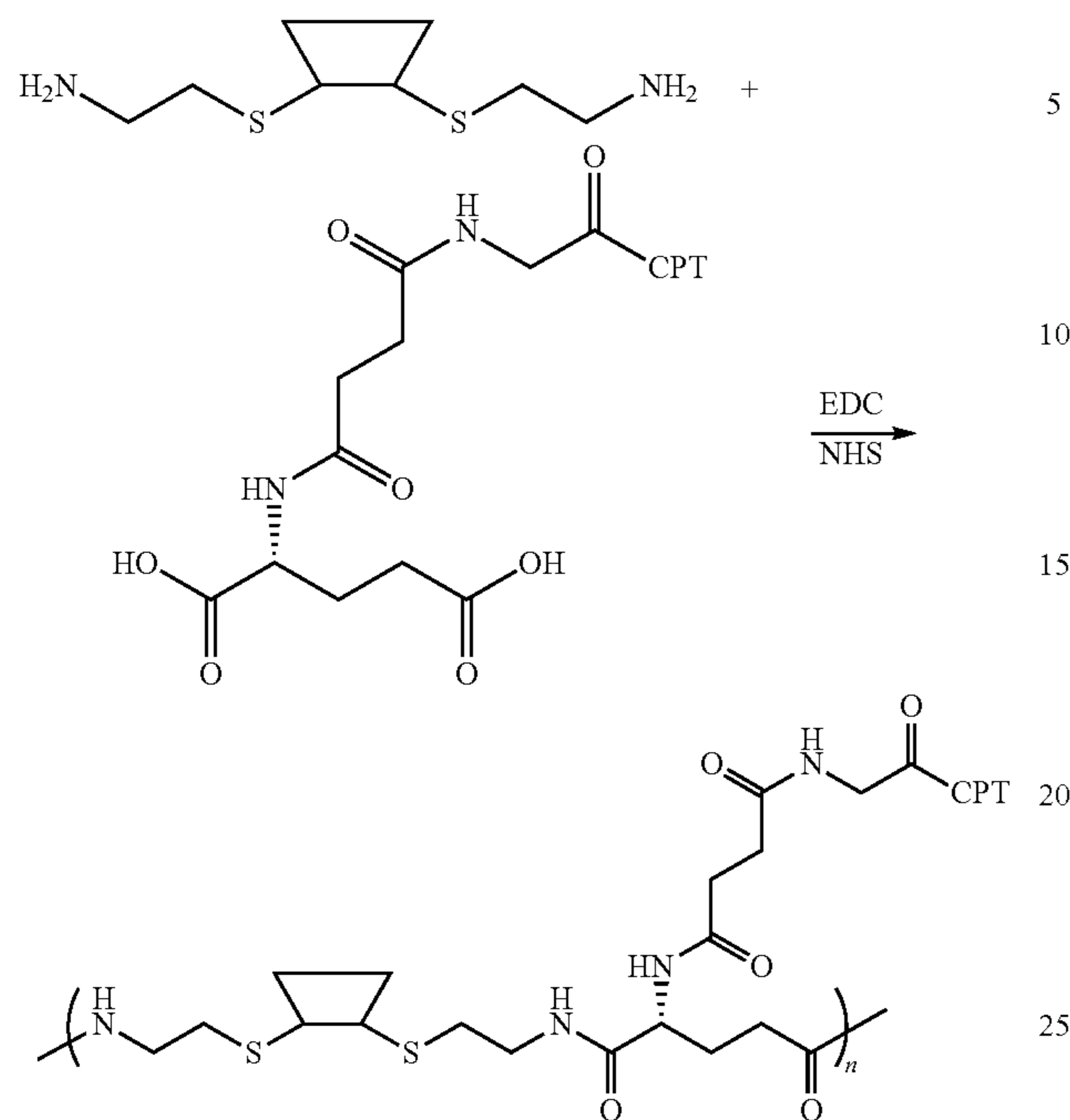
Scheme VI
