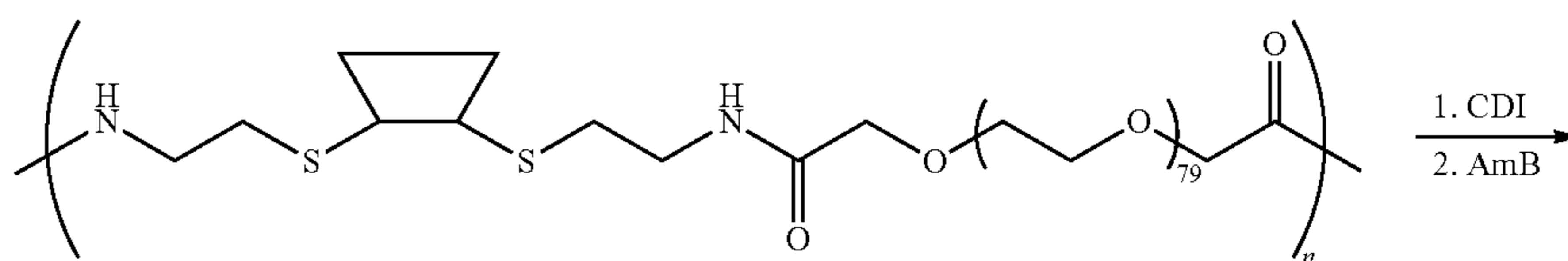
Scheme LII
