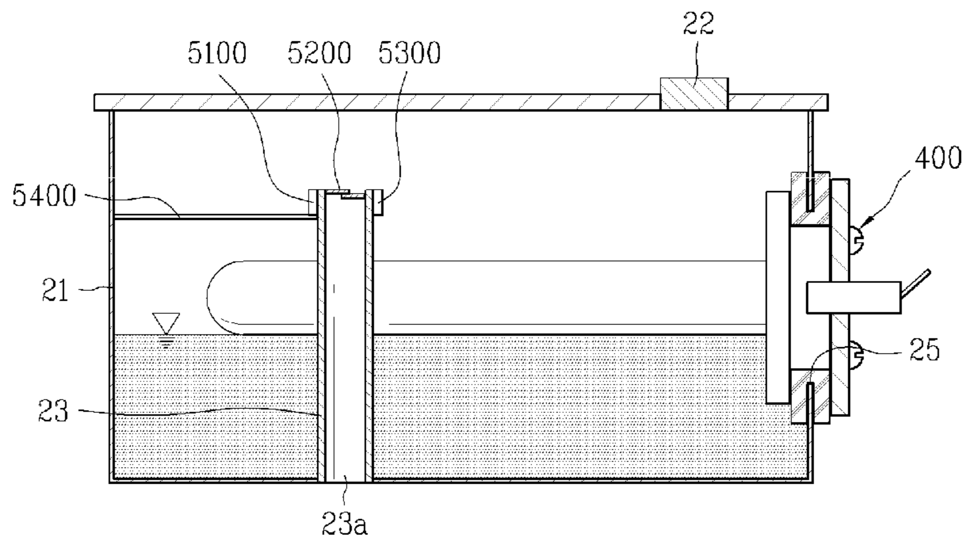
FIG. 6A
