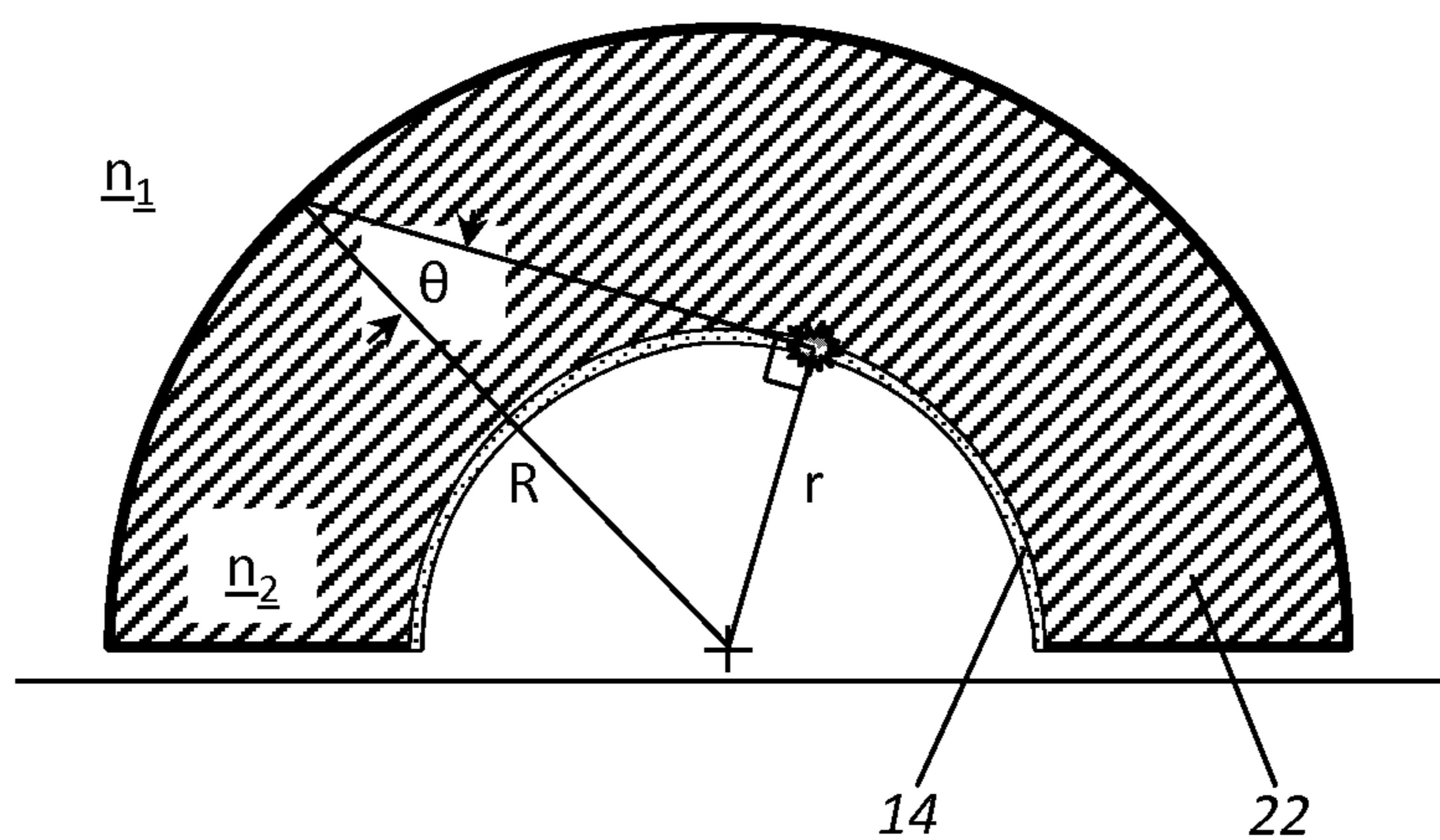
FIG. 5B
