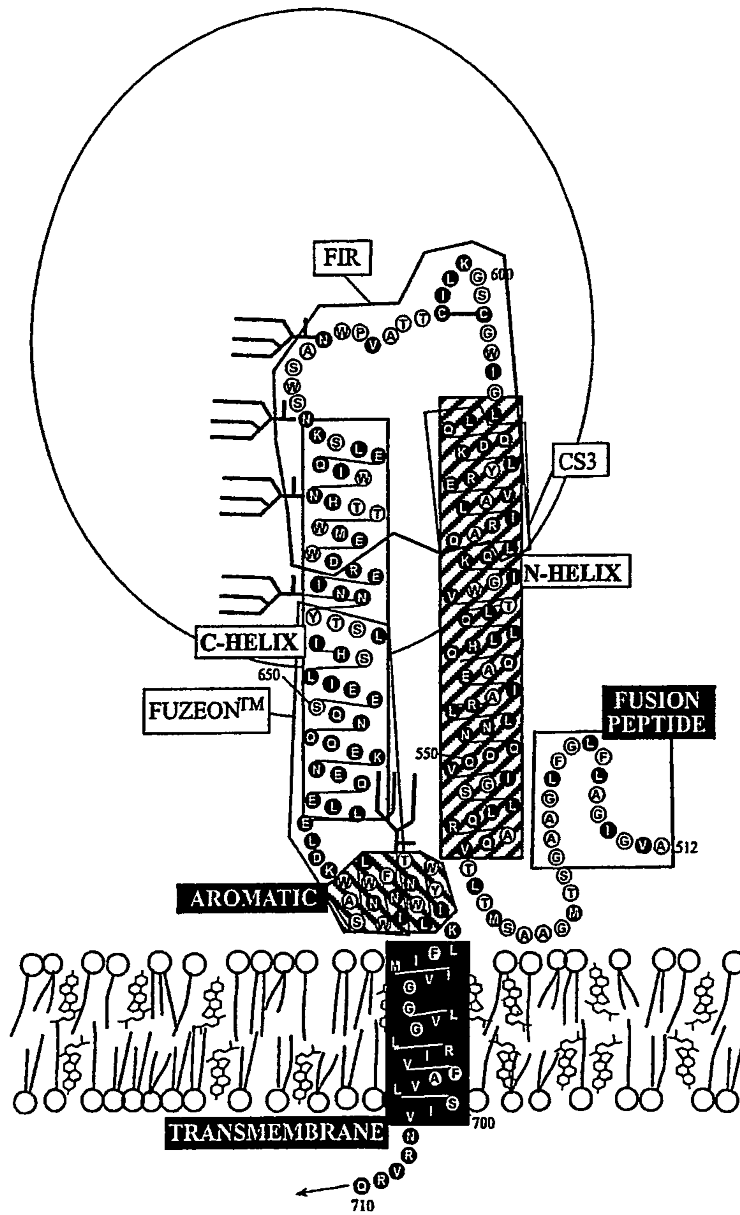
HIV-1 TM Figure 7
