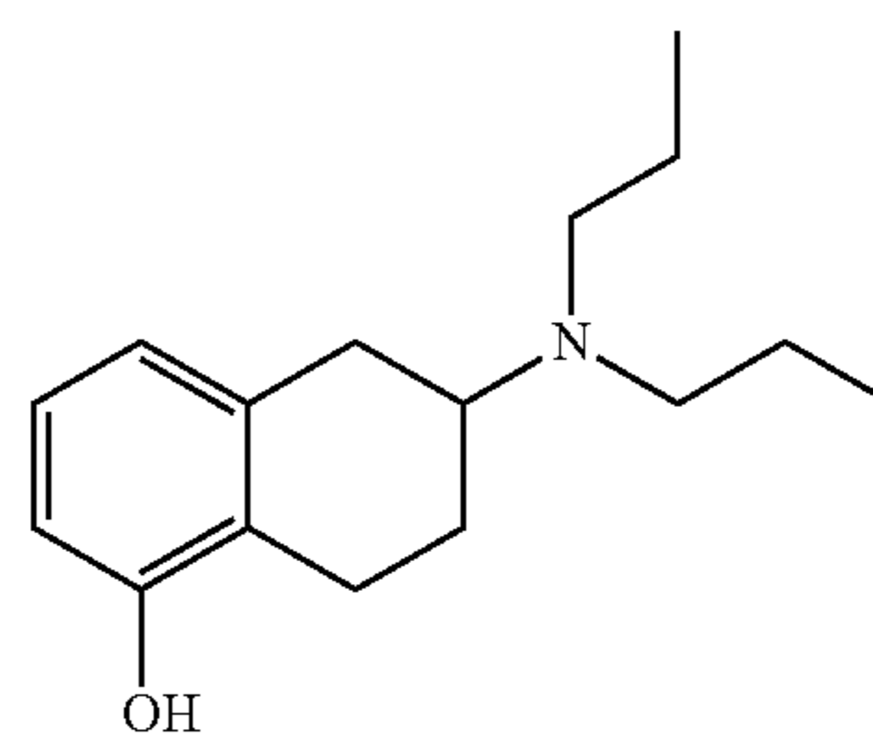
5-OH-DPAT
