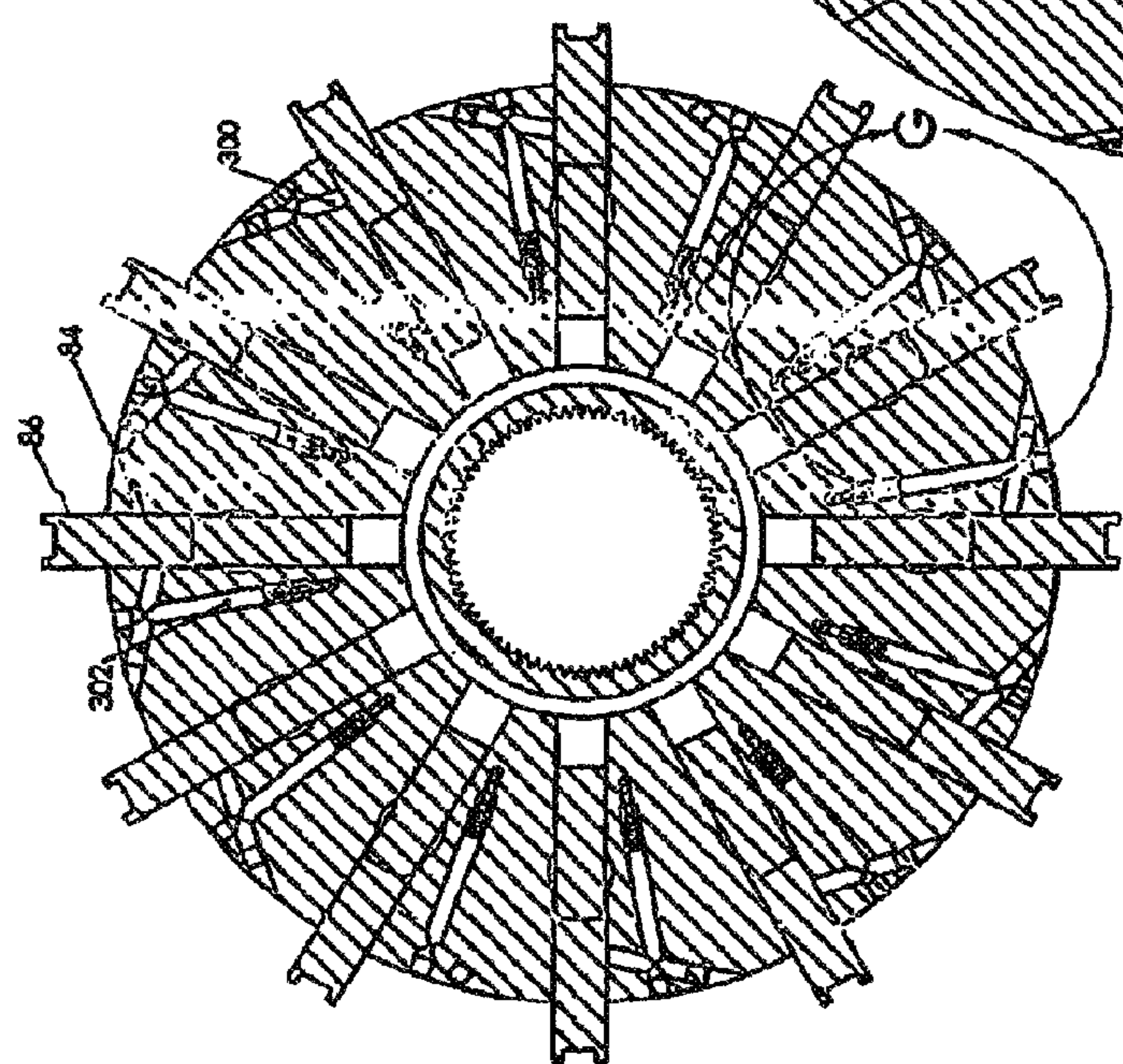
SECTION F-F SCALE 5:1 FIG. 19
