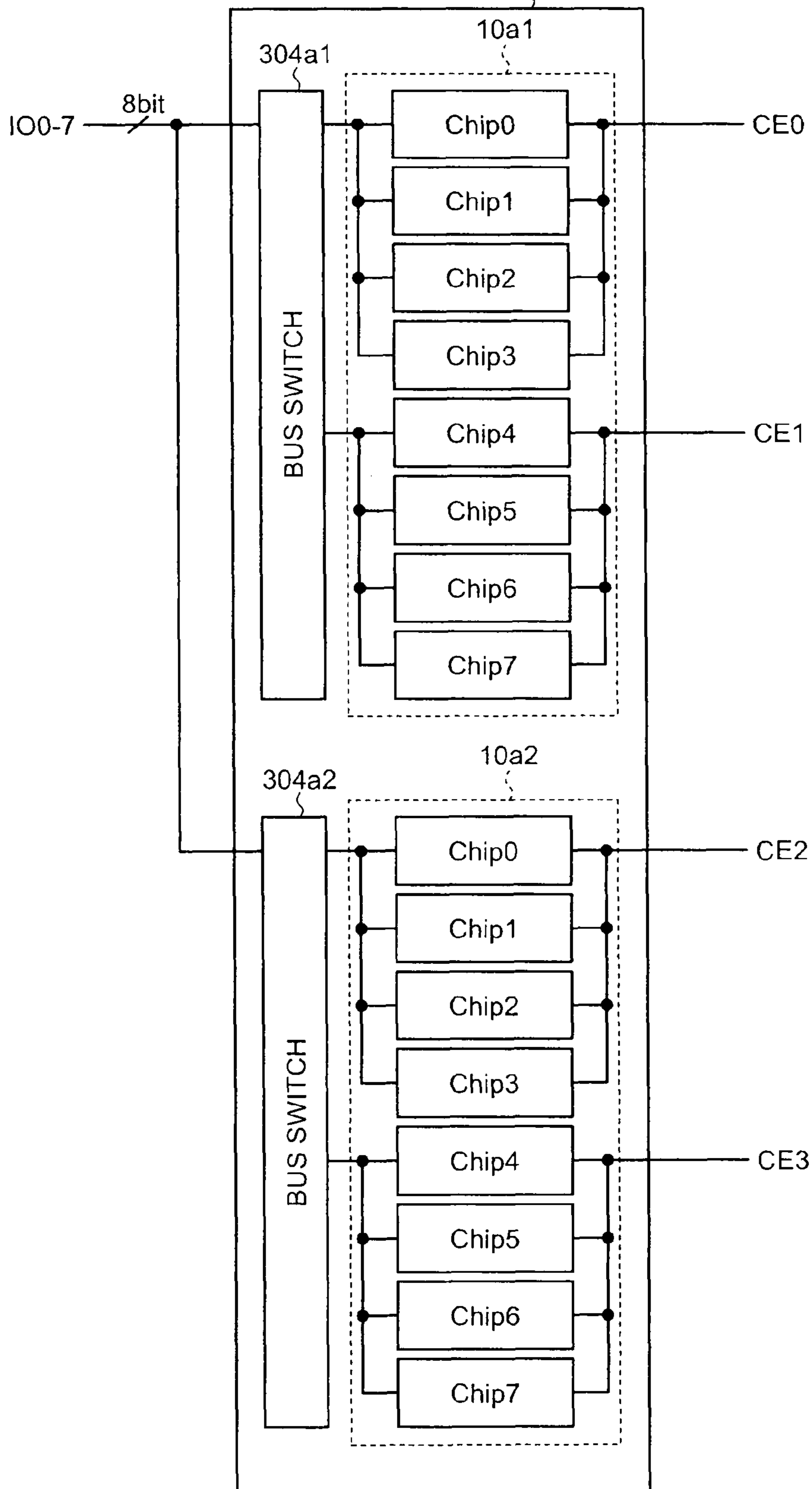
FIG. 15 NAND MEMORY PACKAGE 10a
