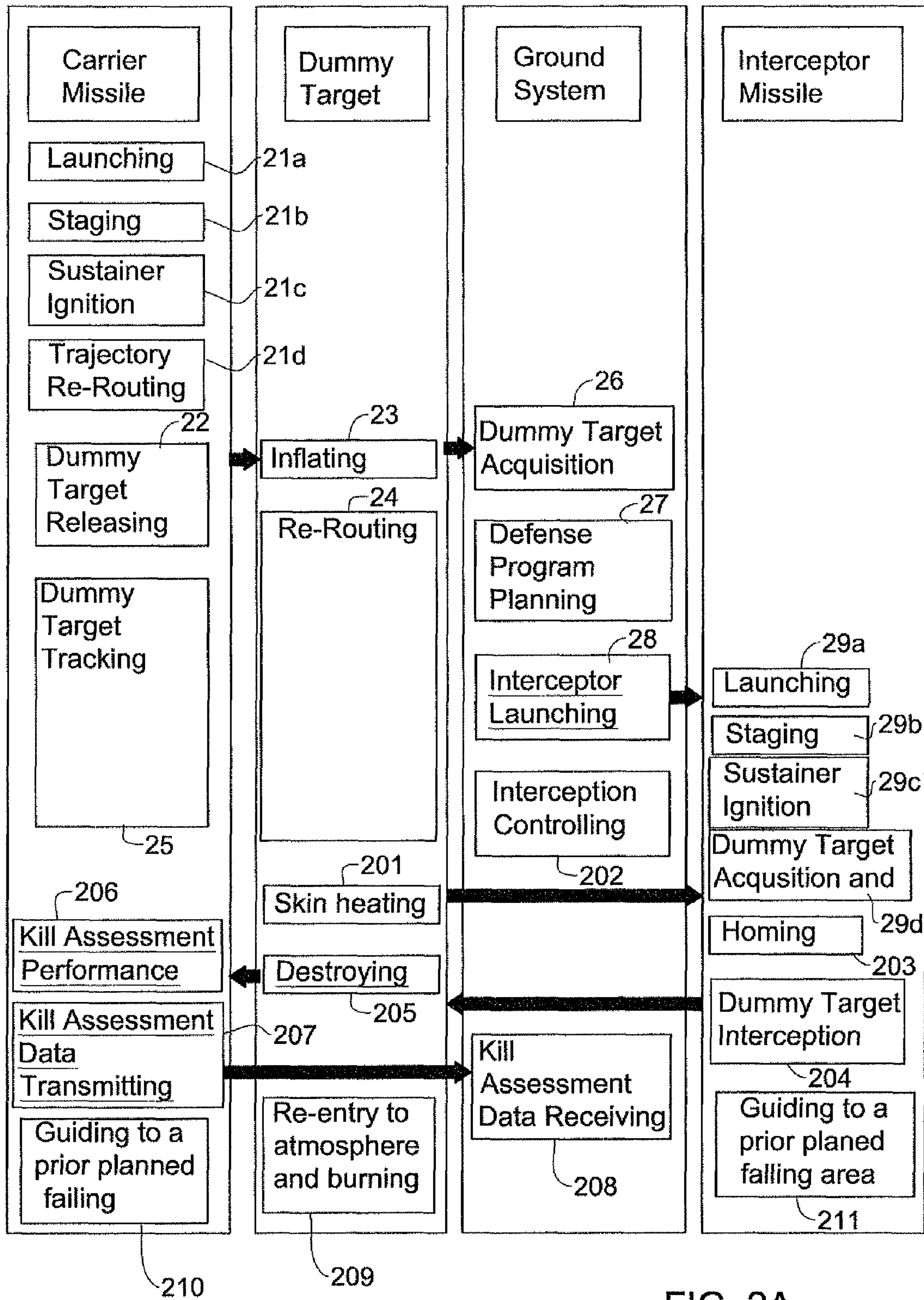
FIG. 2A
