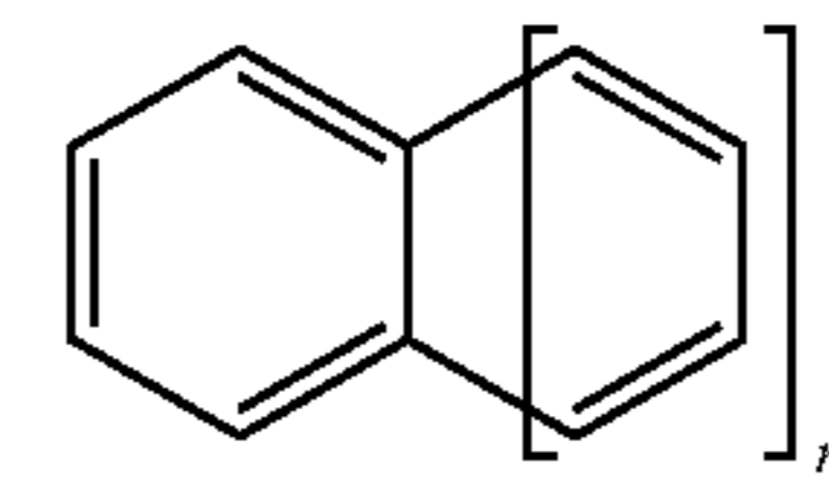
acenes
