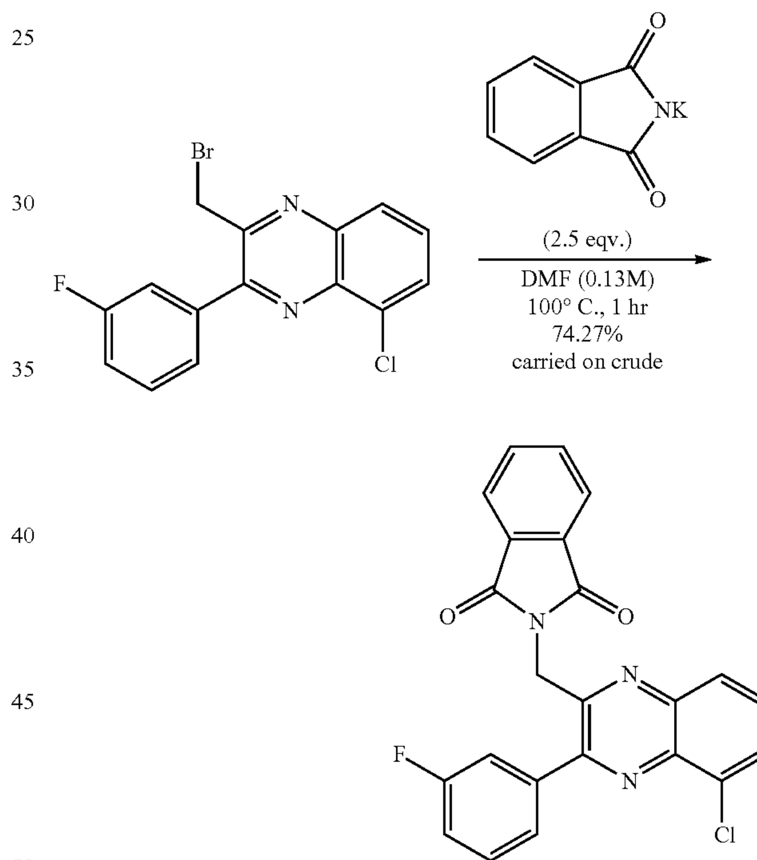
2-(Bromomethyl)-5-chloro-3-(3-fluorophenyl)quinoxaline
