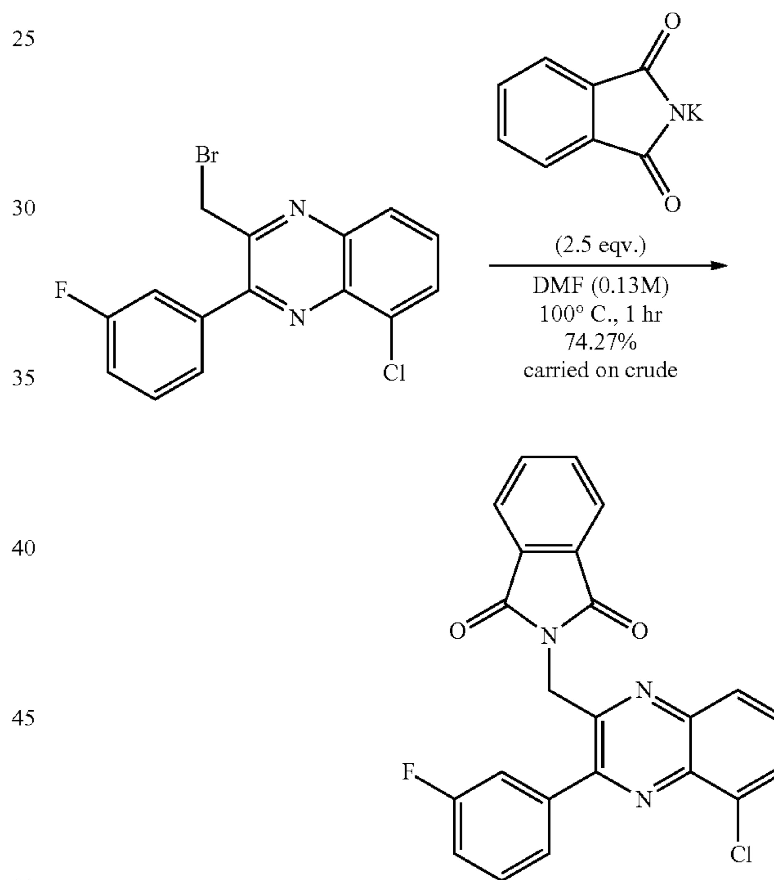
2-(Bromomethyl)-5-chloro-3-(3-fluorophenyl)quinoxaline
