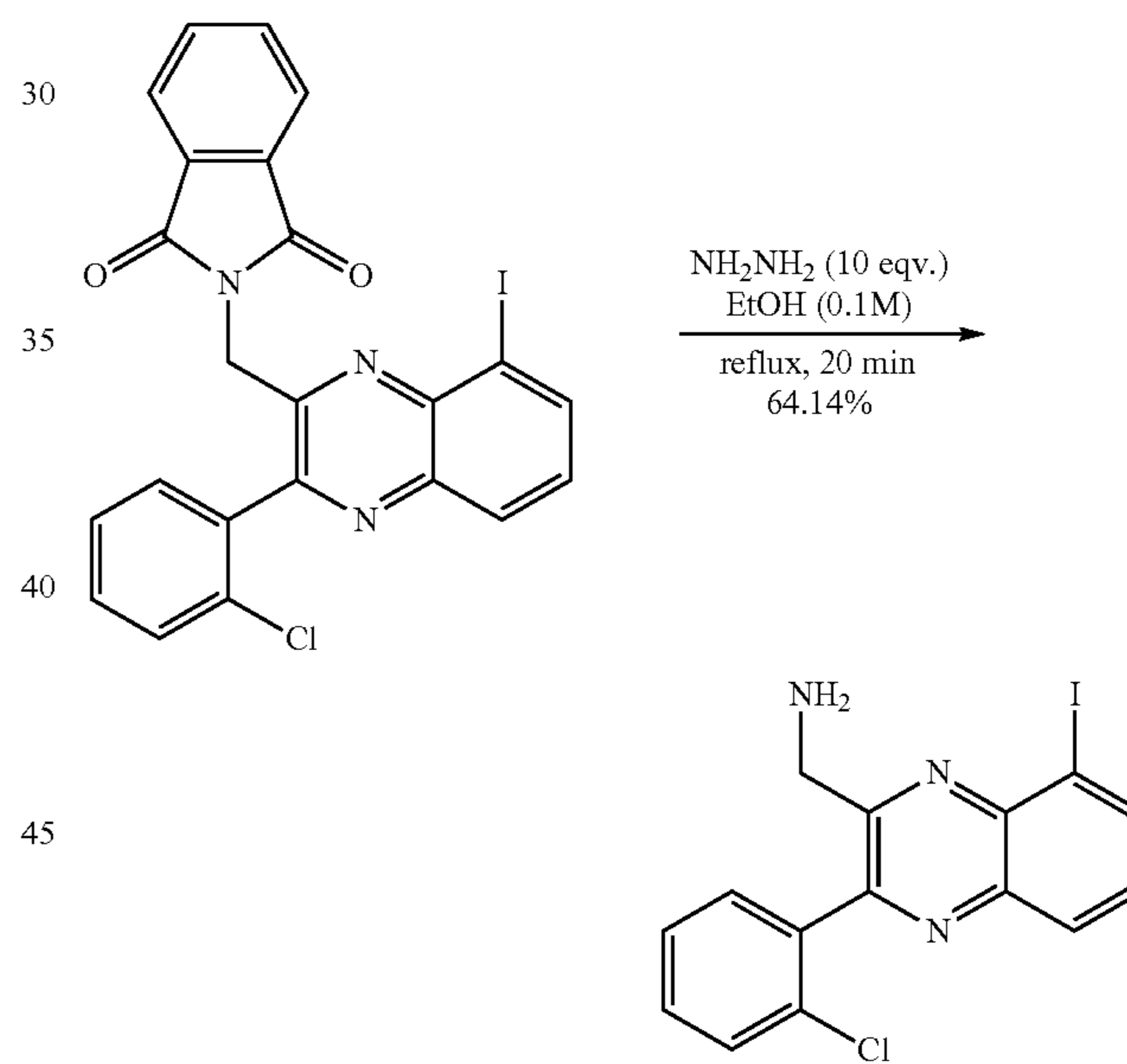
2-((3-(2-Chlorophenyl)-8-iodoquinoxalin-2-yl)methyl)isoindoline-1,3-dione
