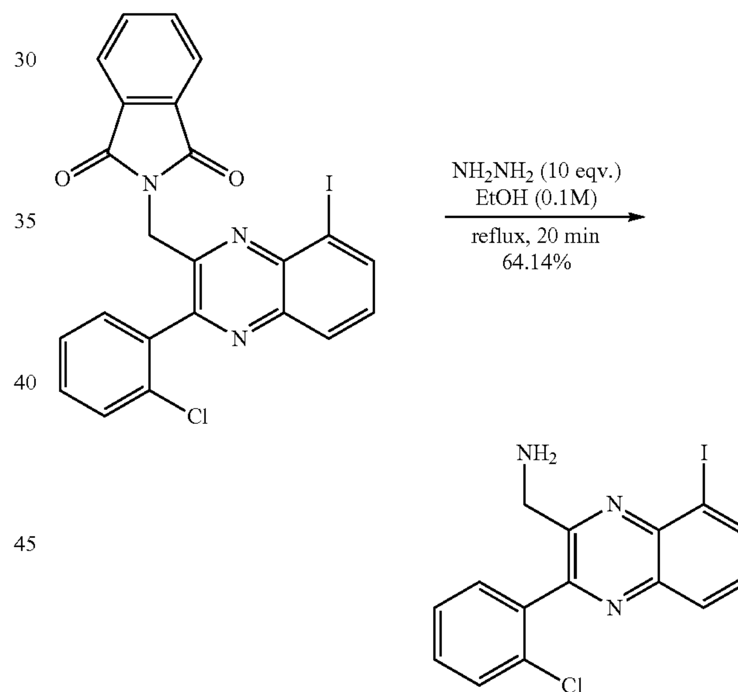
2-((3-(2-Chlorophenyl)-8-iodoquinoxalin-2-yl)methyl)isoindoline-1,3-dione
