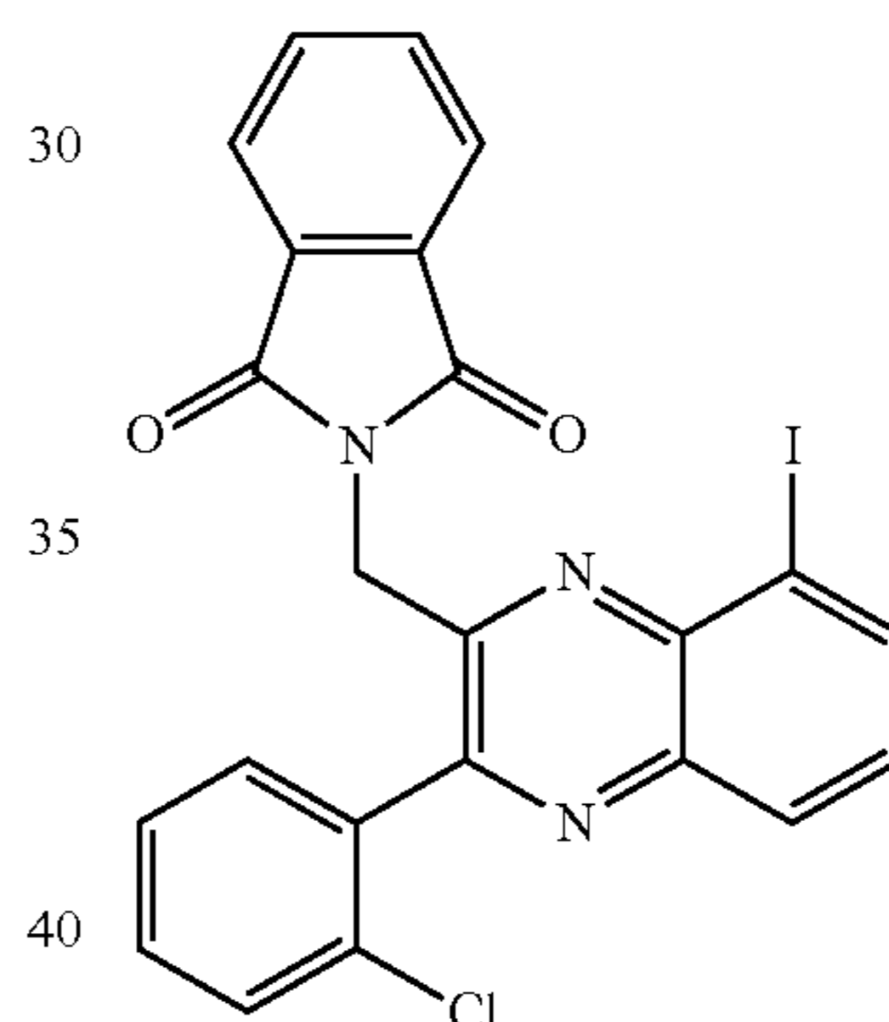
2-((3-(2-Chlorophenyl)-8-iodoquinoxalin-2-yl)methyl)isoindoline-1,3-dione
