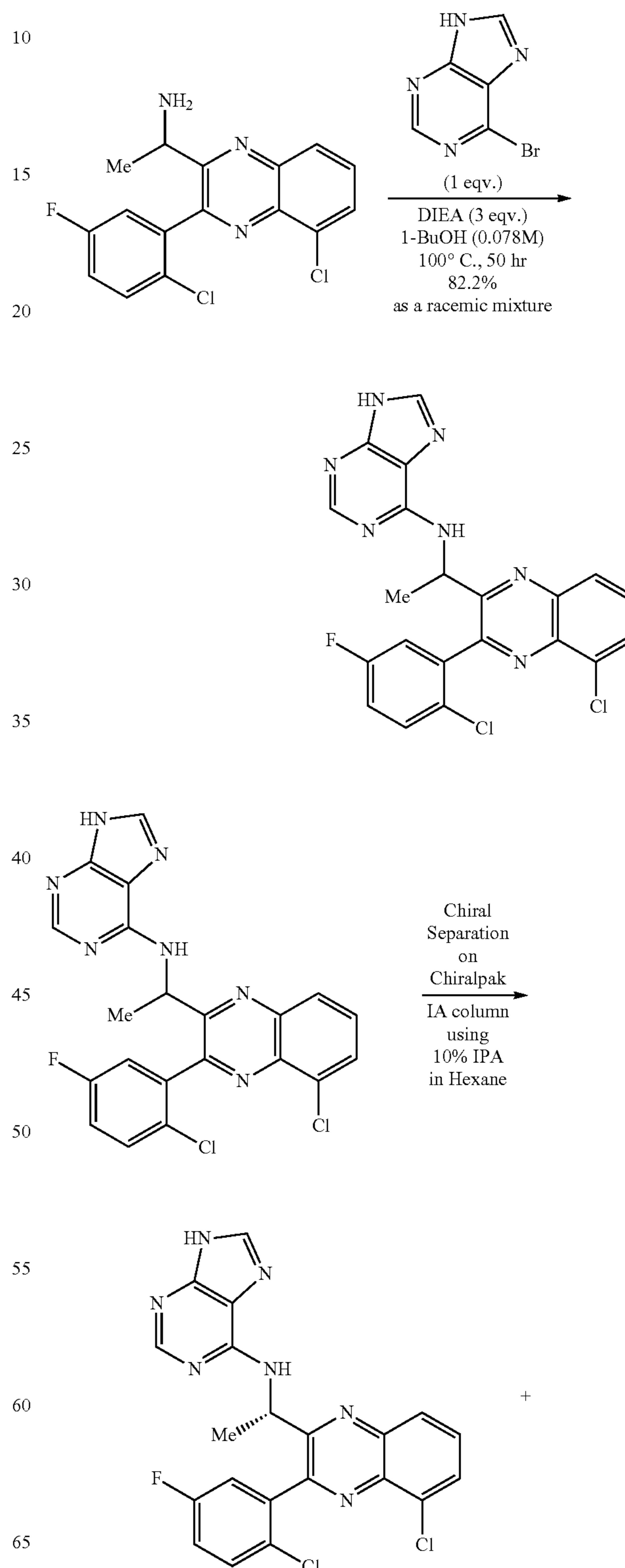
1-(5-Chloro-3-(2-chloro-5-fluorophenyl)quinoxalin-2-yl)ethanamine
