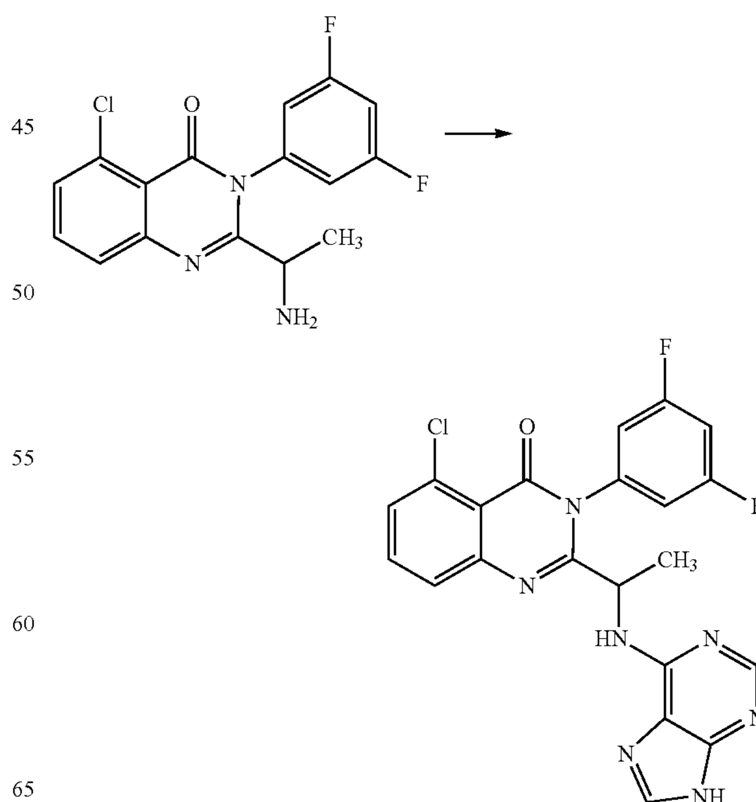
2-(1-amino-ethyl)-5-chloro-3-(3,5-difluoro-phenyl)-3H-quinazolin-4-one (170)
