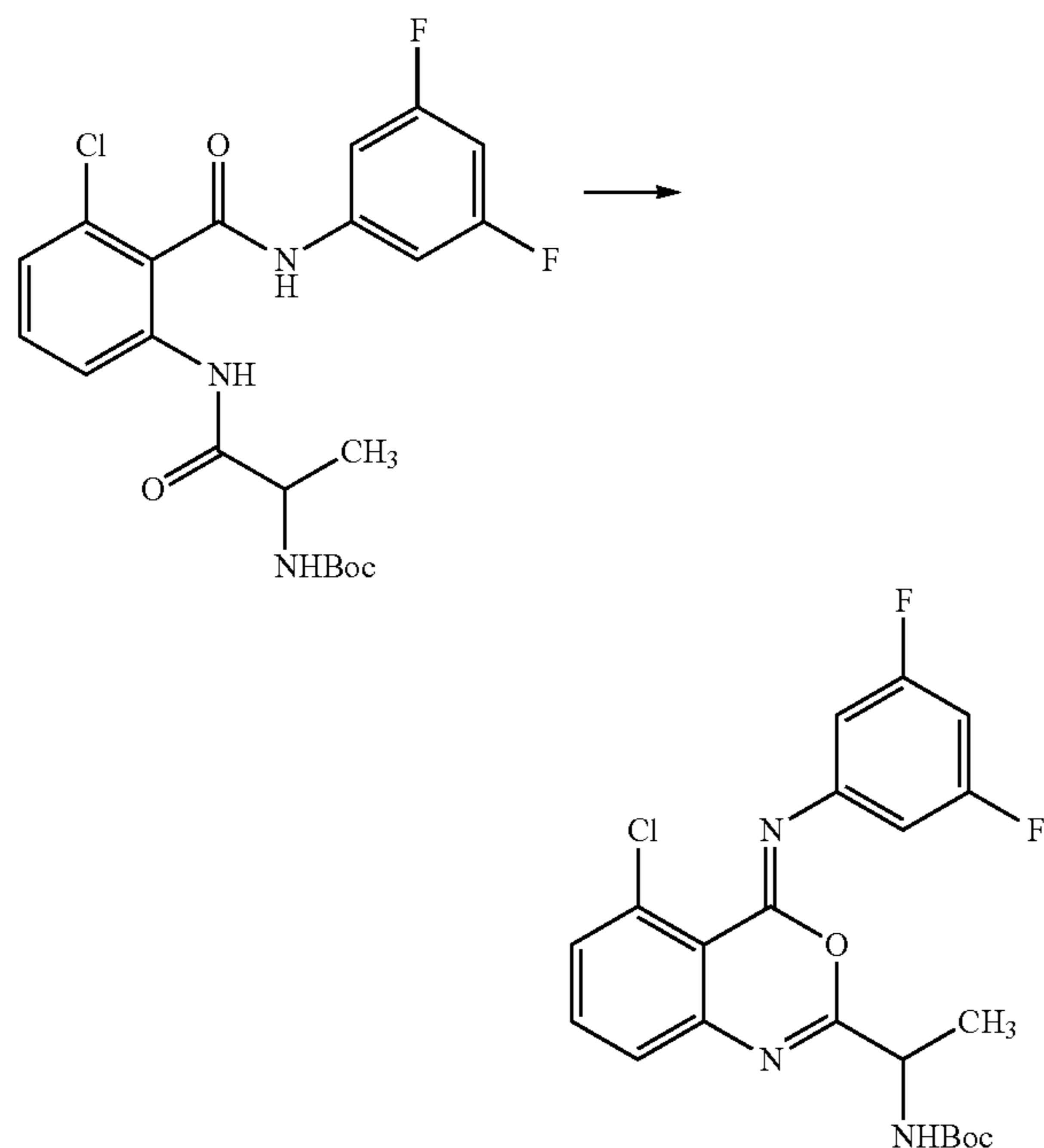
2-(1-amino-ethyl)-5-chloro-3-(3,5-difluoro-phenyl)-3H-quinazolin-4-one (170)
