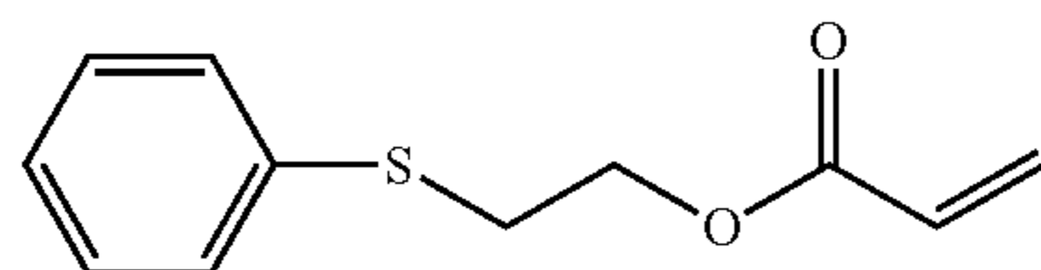
PTEA
