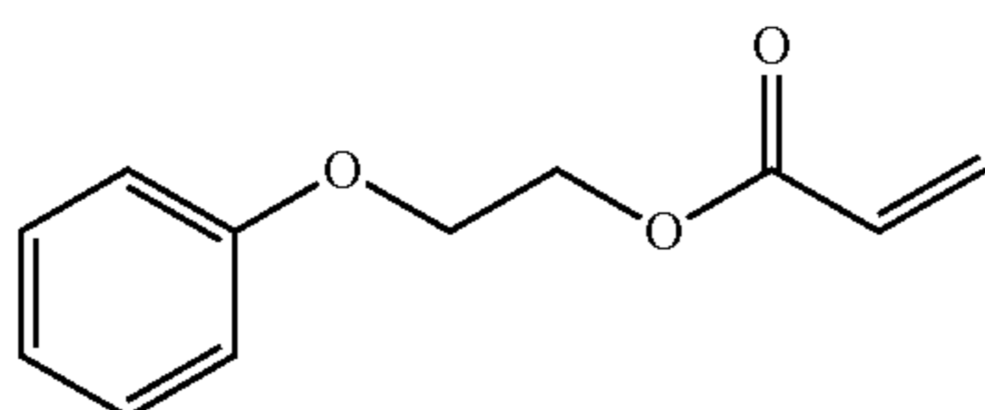
PEA
