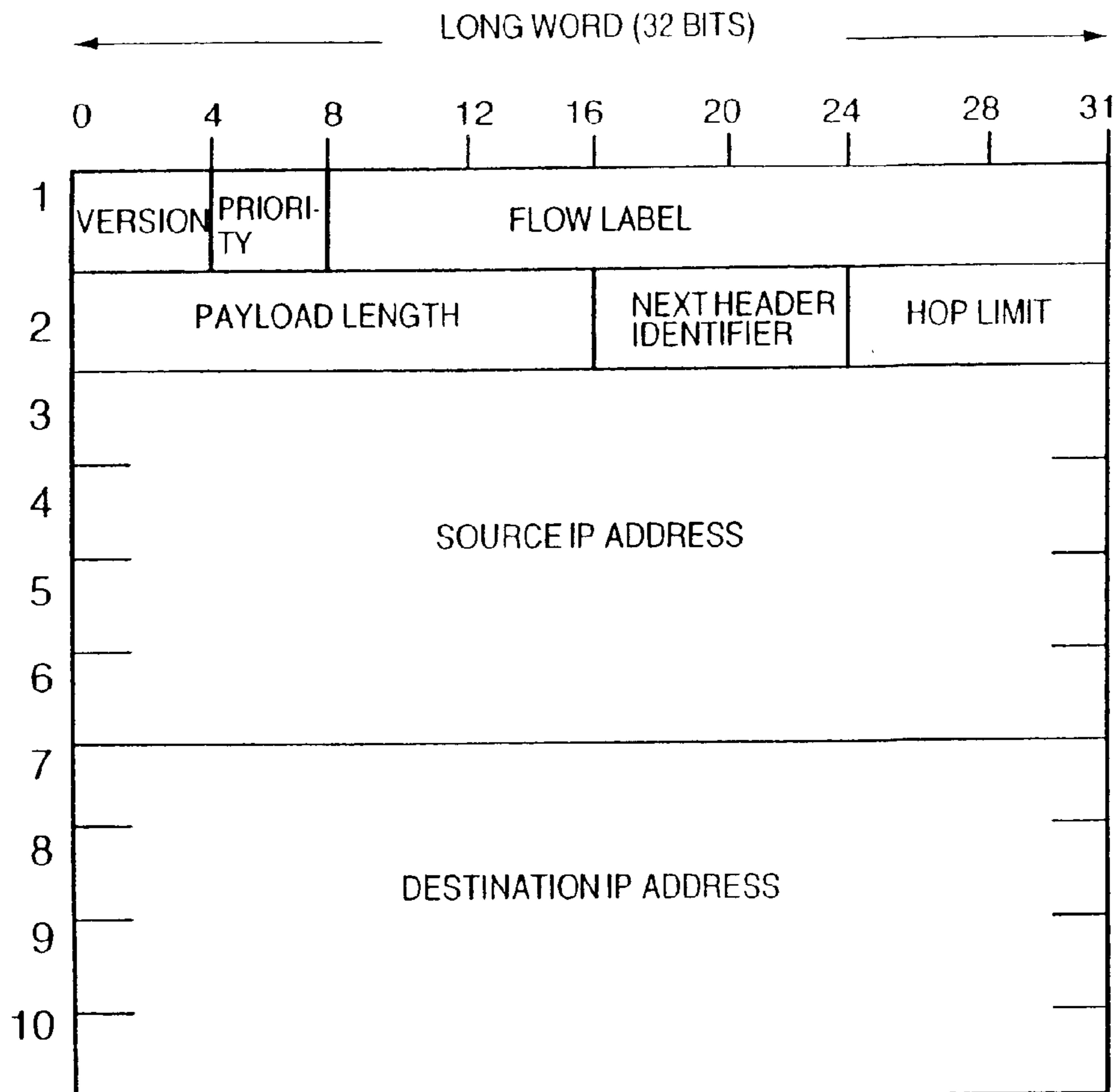
IPv6 HEADER FORMAT
