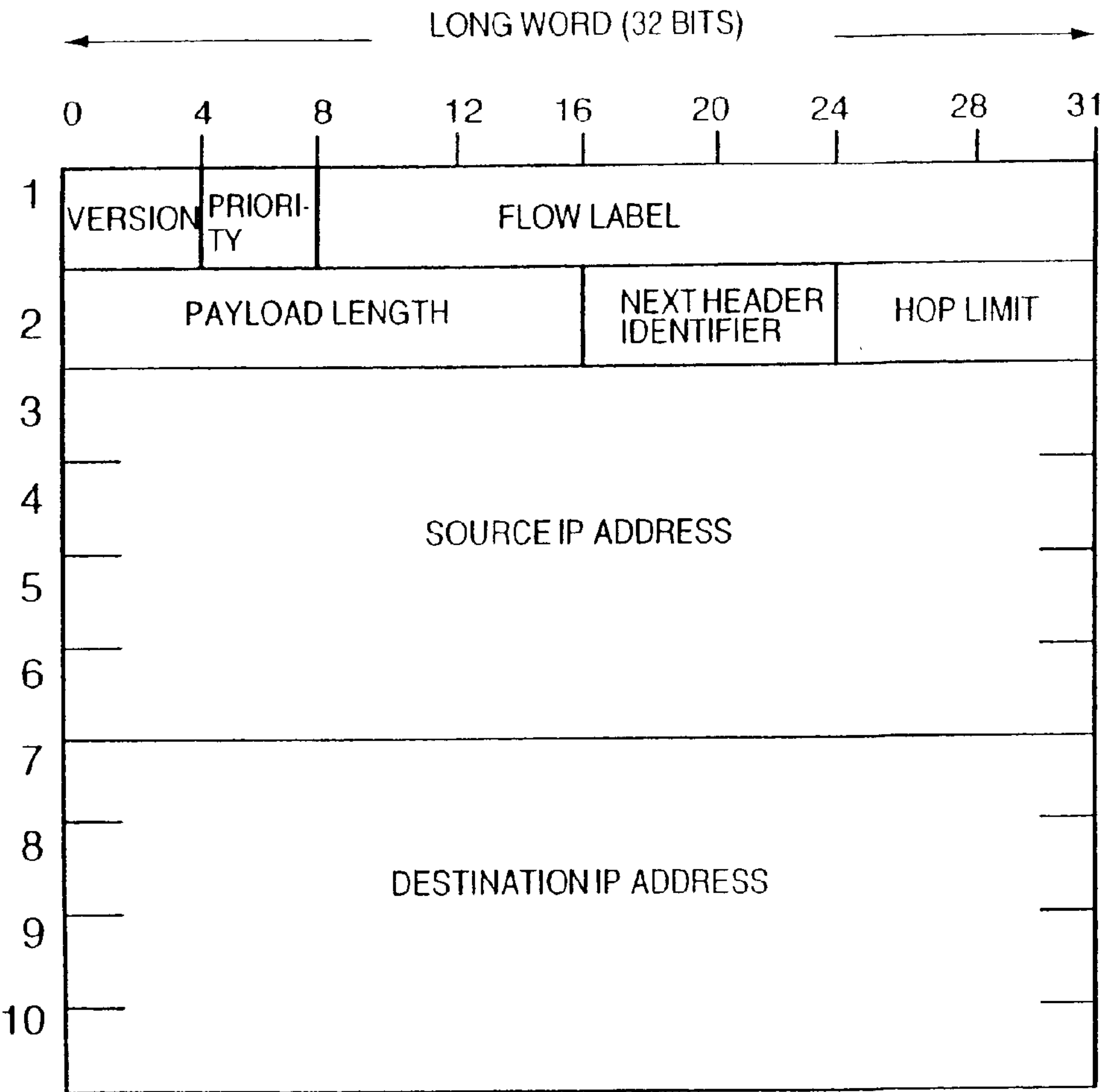
IPv6 HEADER FORMAT
