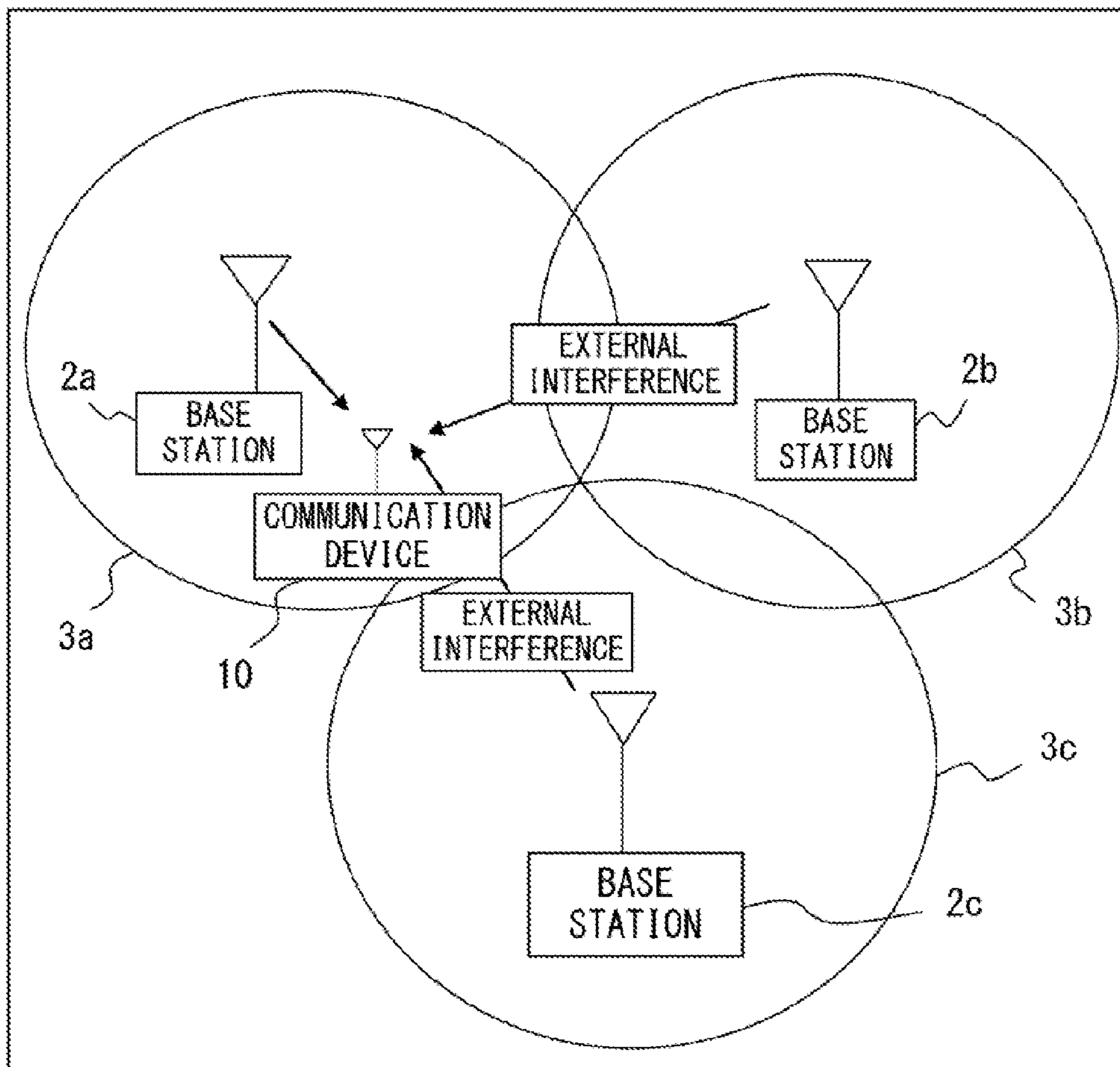
FIG. 4A
