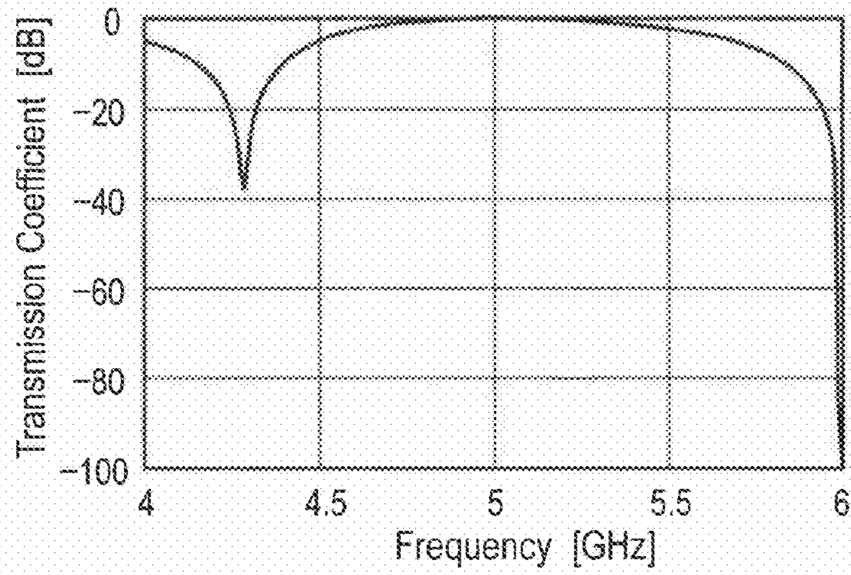
FIG. 12A
