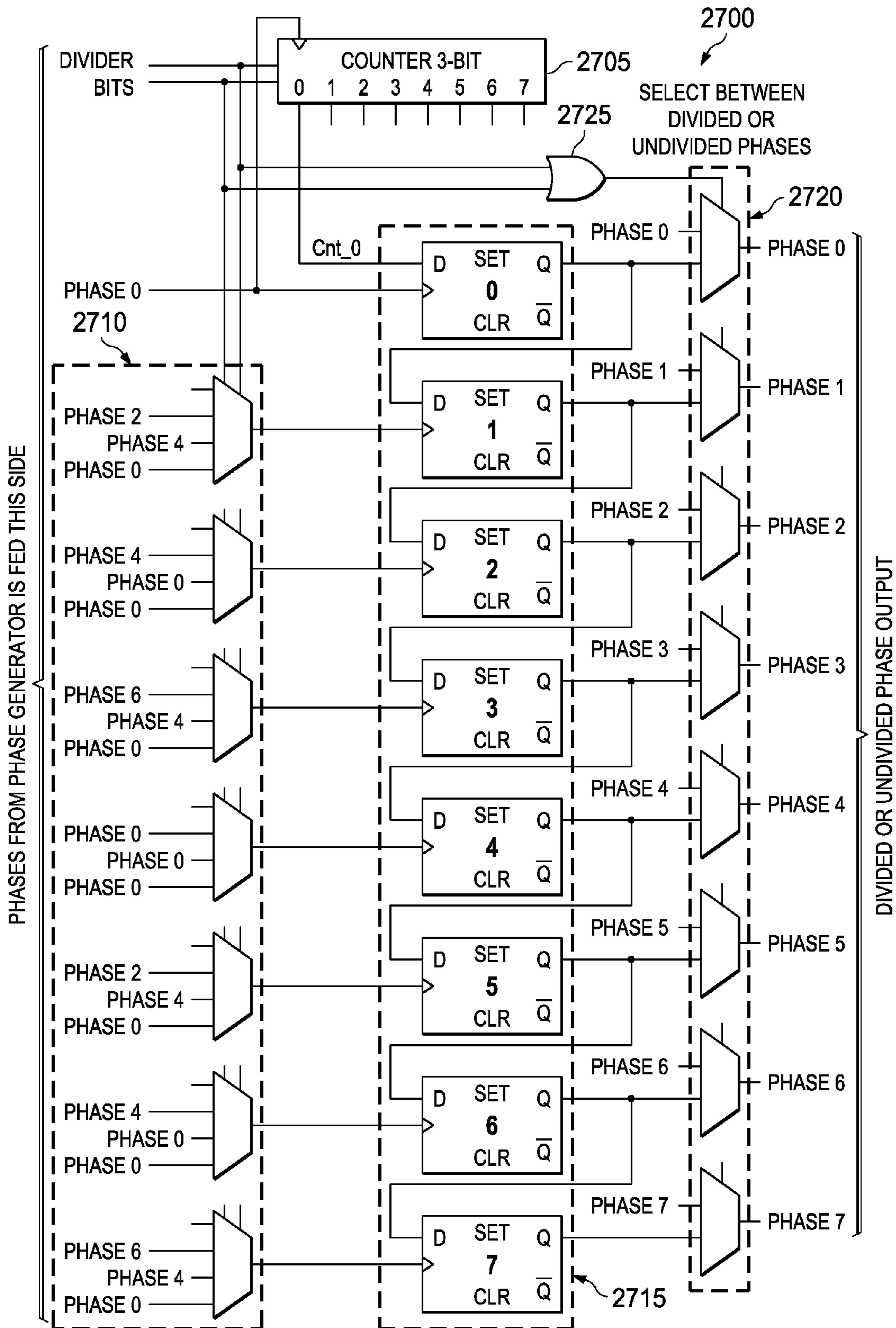
FIG. 27
