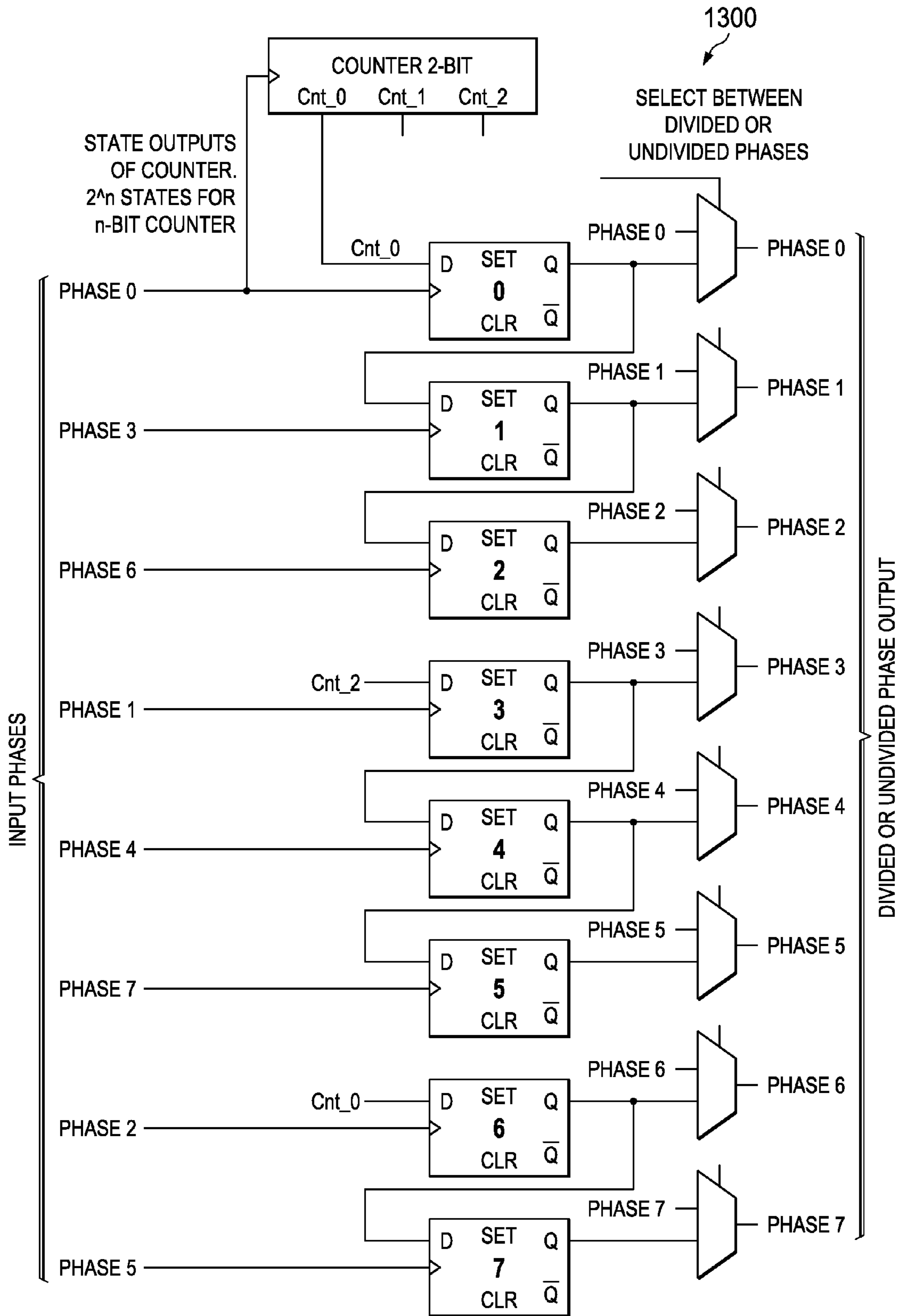
FIG. 13
