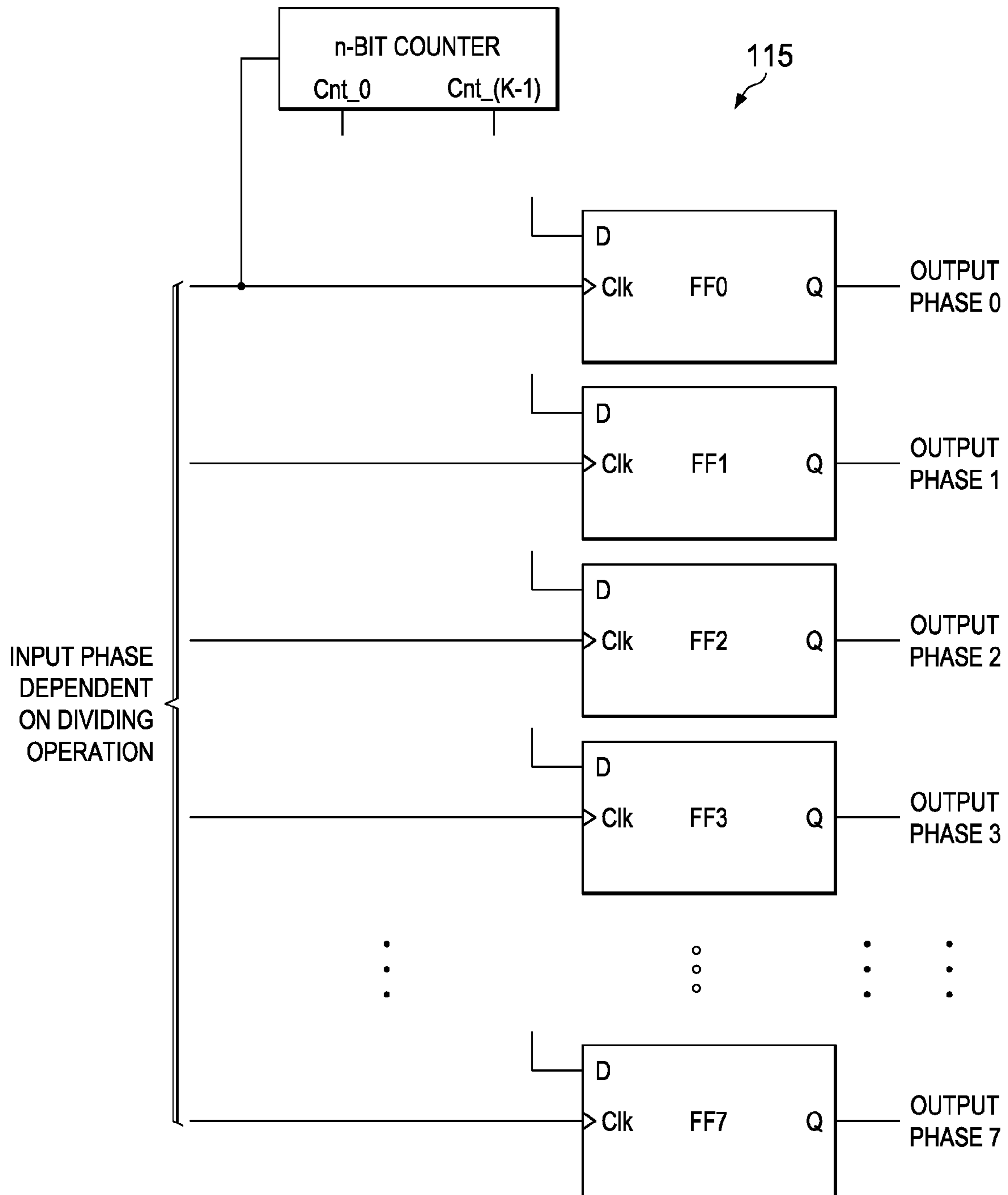
FIG. 6
