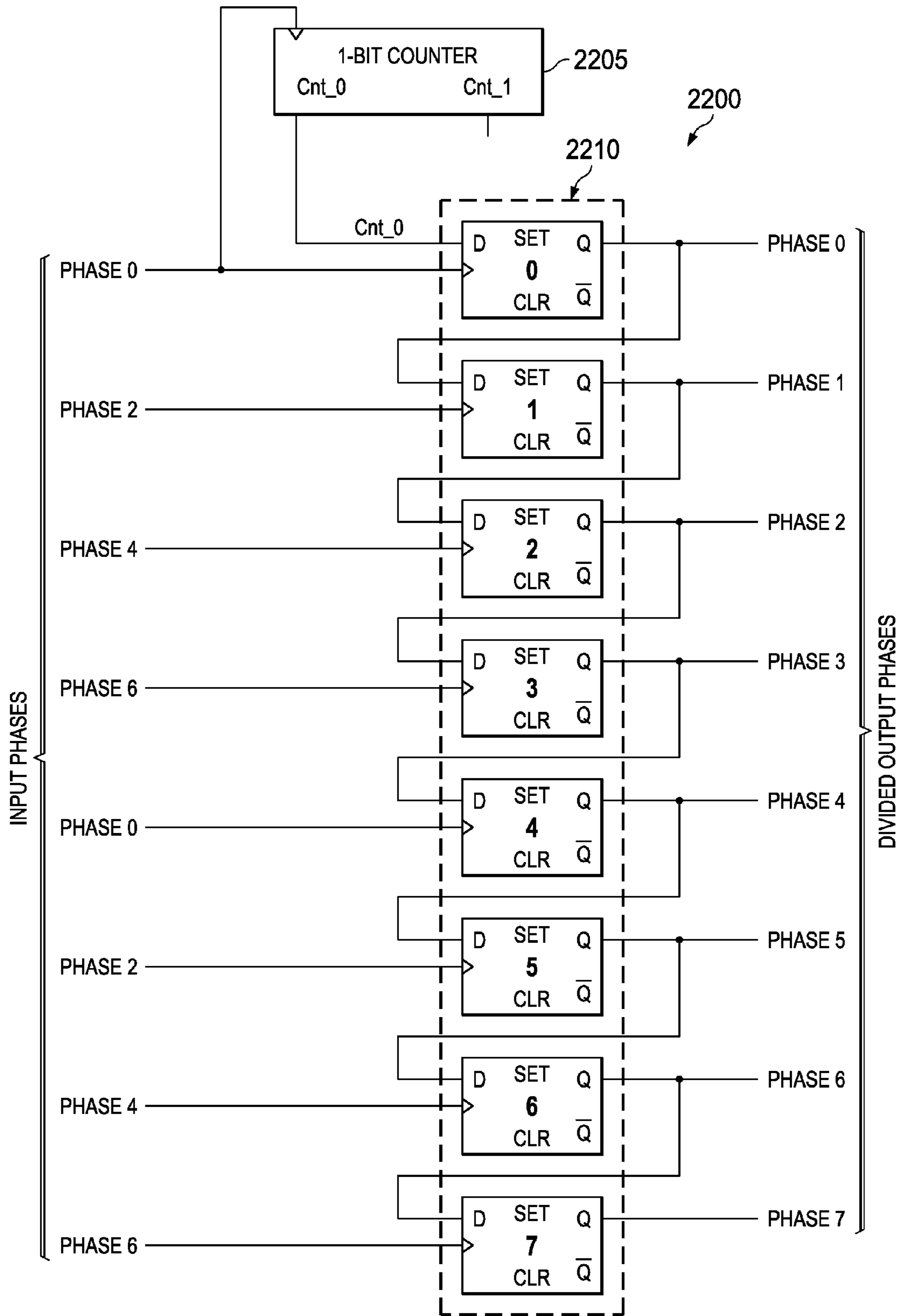
FIG. 22
