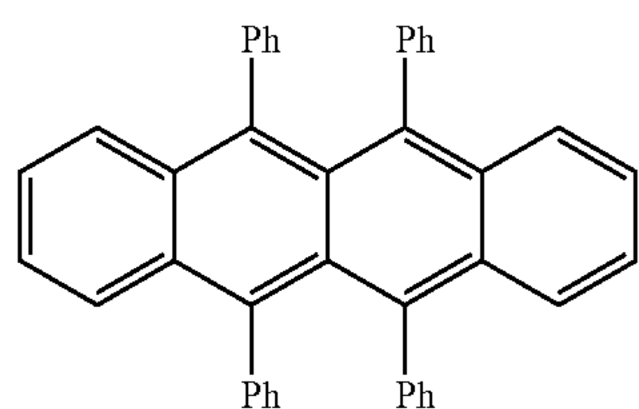
Rubrene
