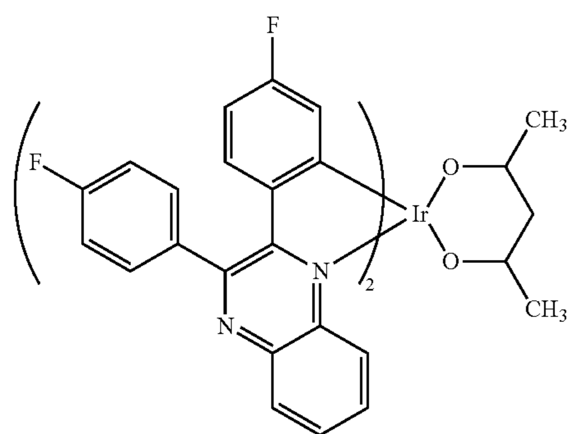
Ir(Fdpq) 2 (acac)
