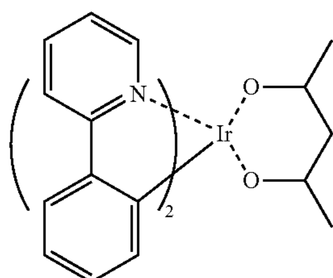
Ir(ppr) 2 acac
