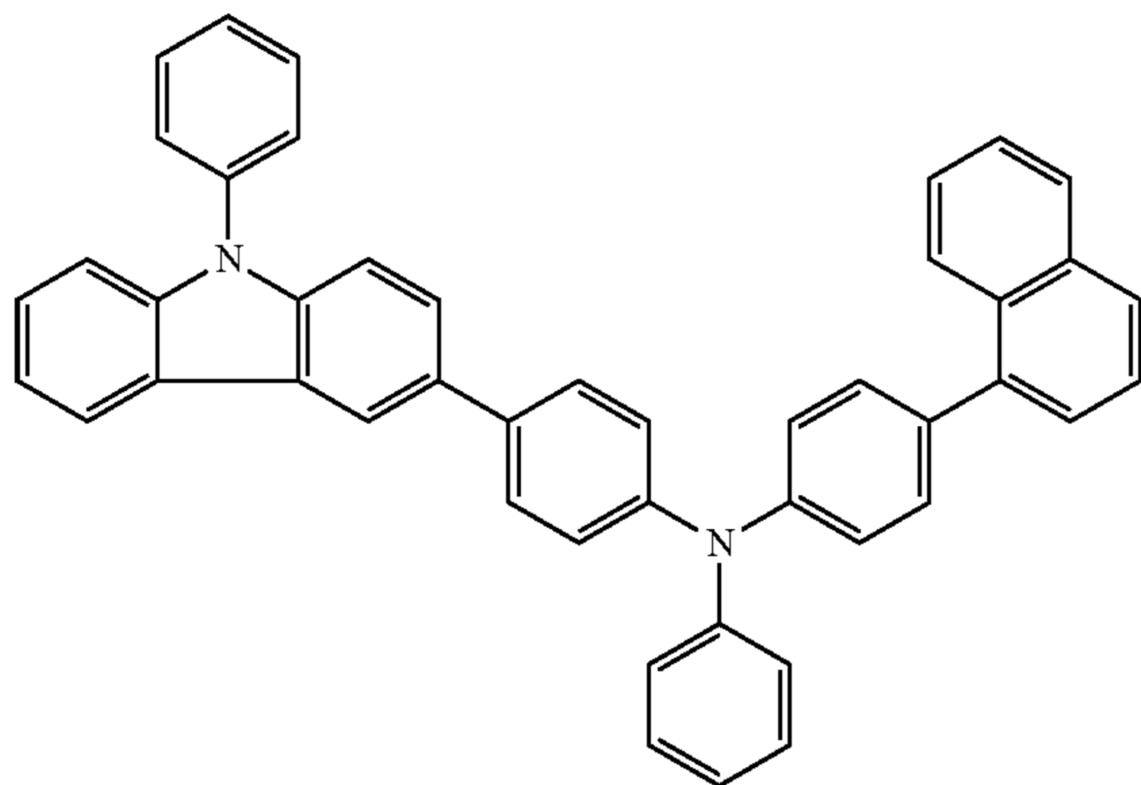
PCBANB
