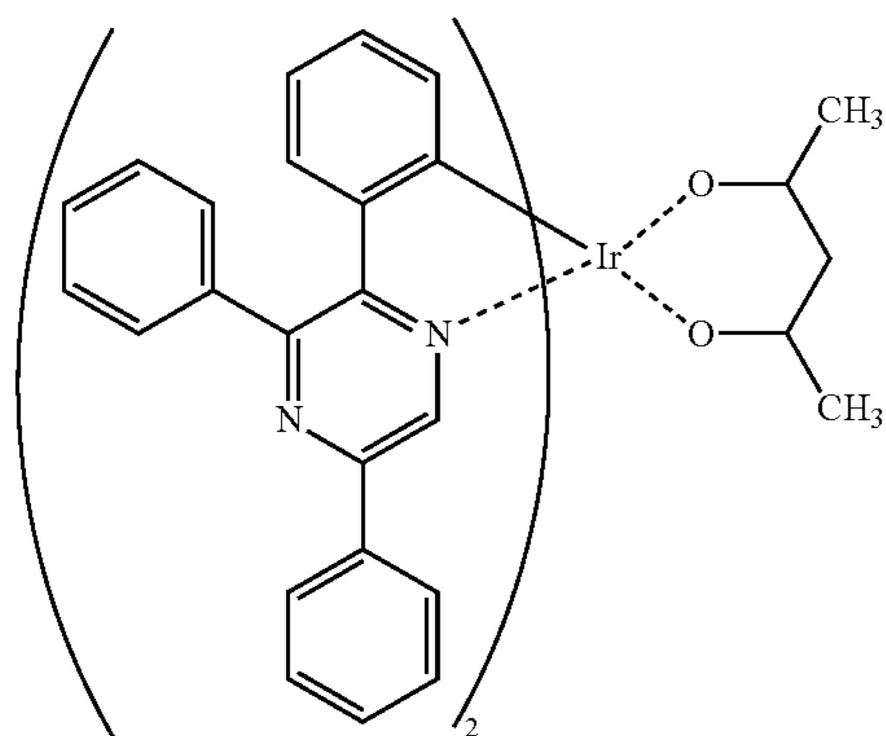
Ir(tppr) 2 acac
