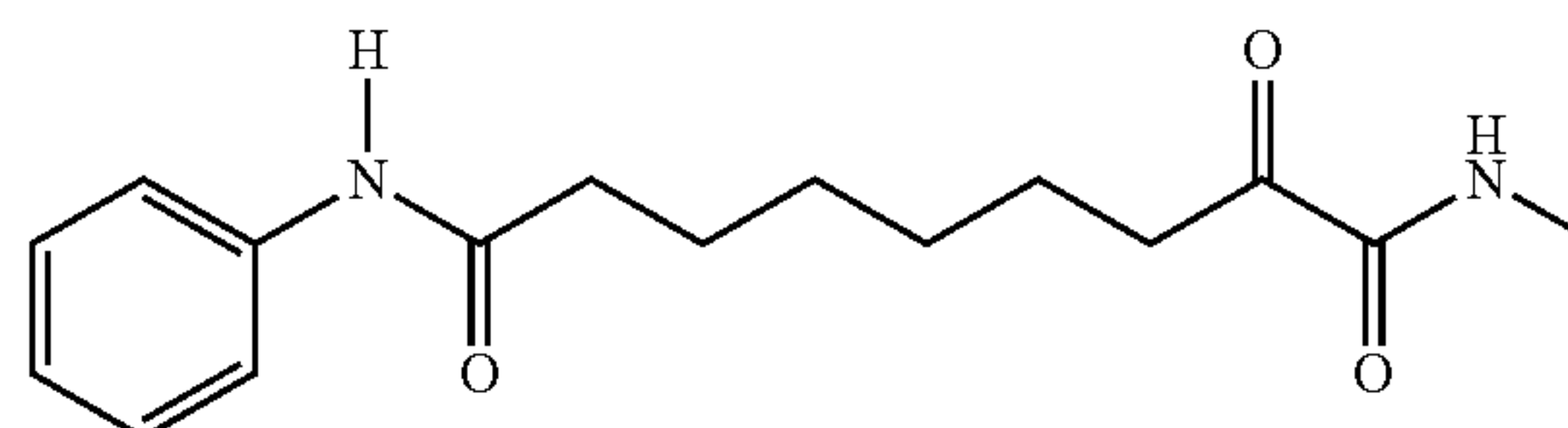
16, alpha-cétoamide
