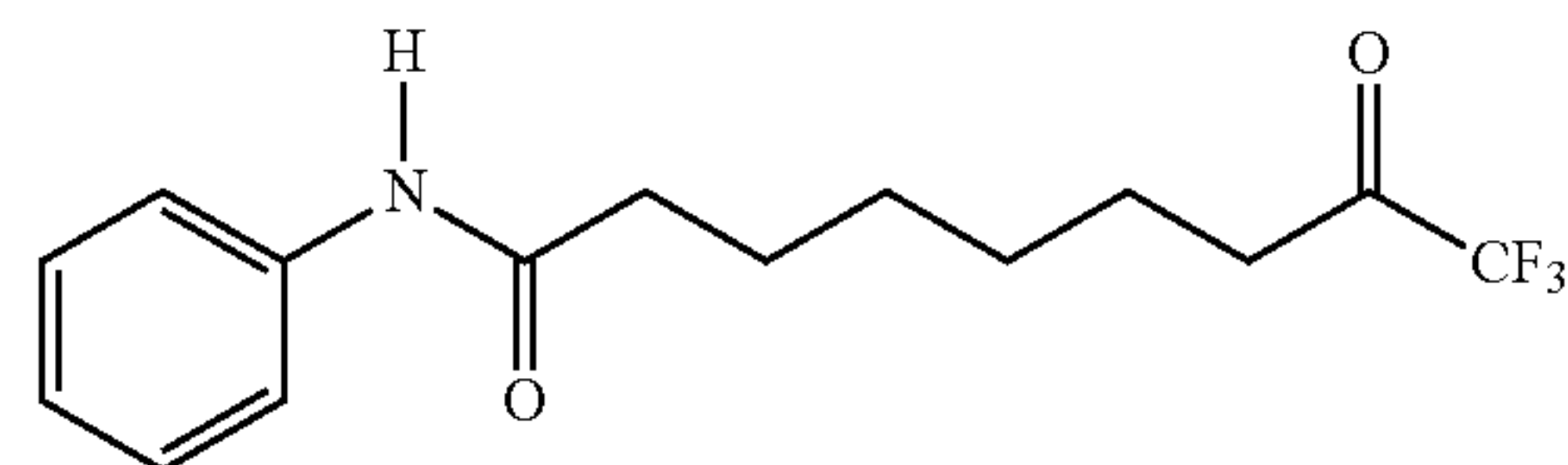
15, Trifluorométhyl cétone
