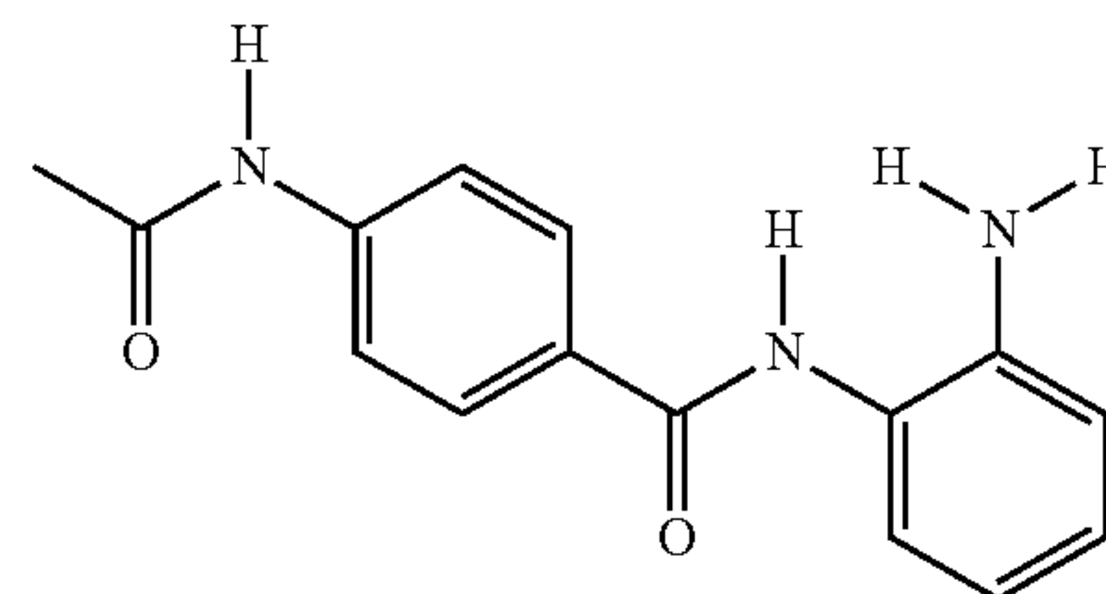
14, CI-994
