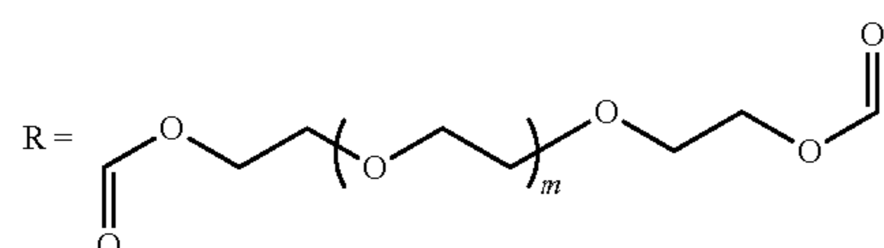
Poly(CDDCys—CB—PEG)
