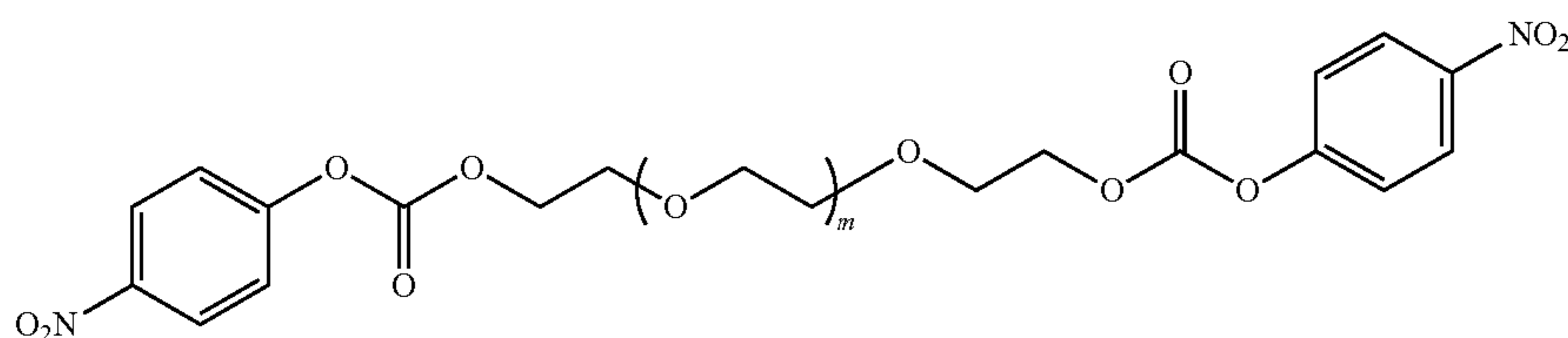
PEG—DiNPC (MW = 3400 kDa)
