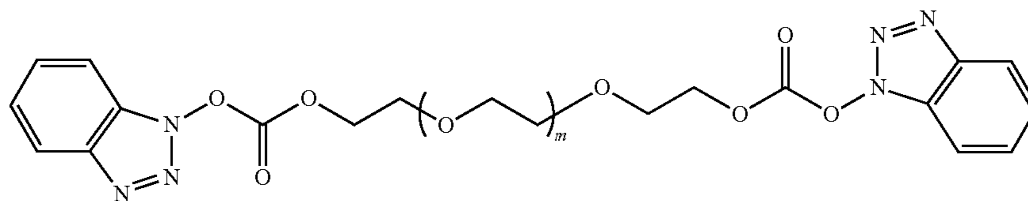
PEG—DiSBA (MW = 3400 kDa)
