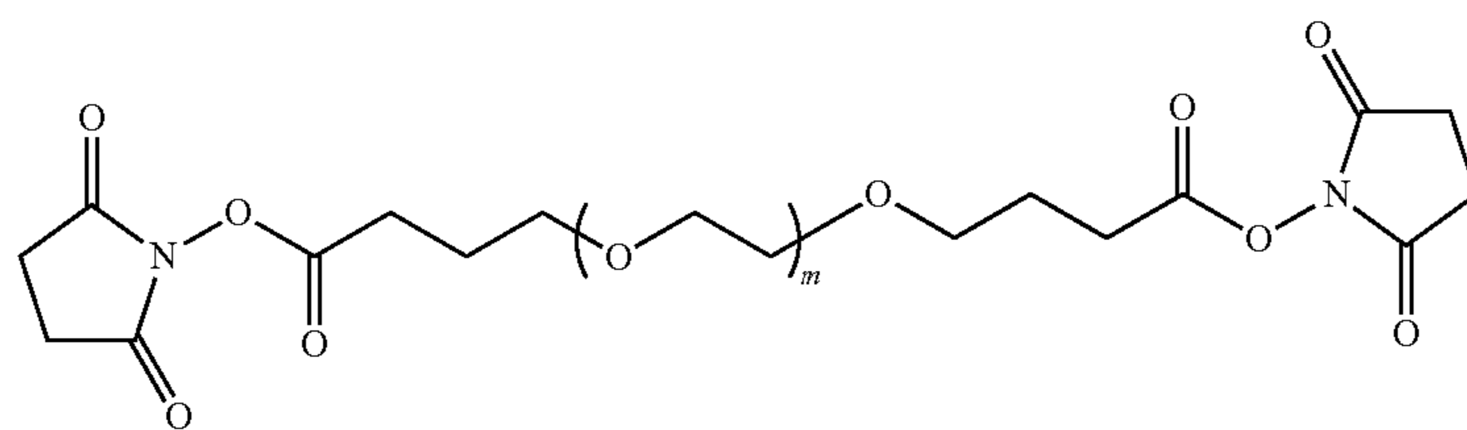
PEG—DiSBA (MW = 3400 kDa)
