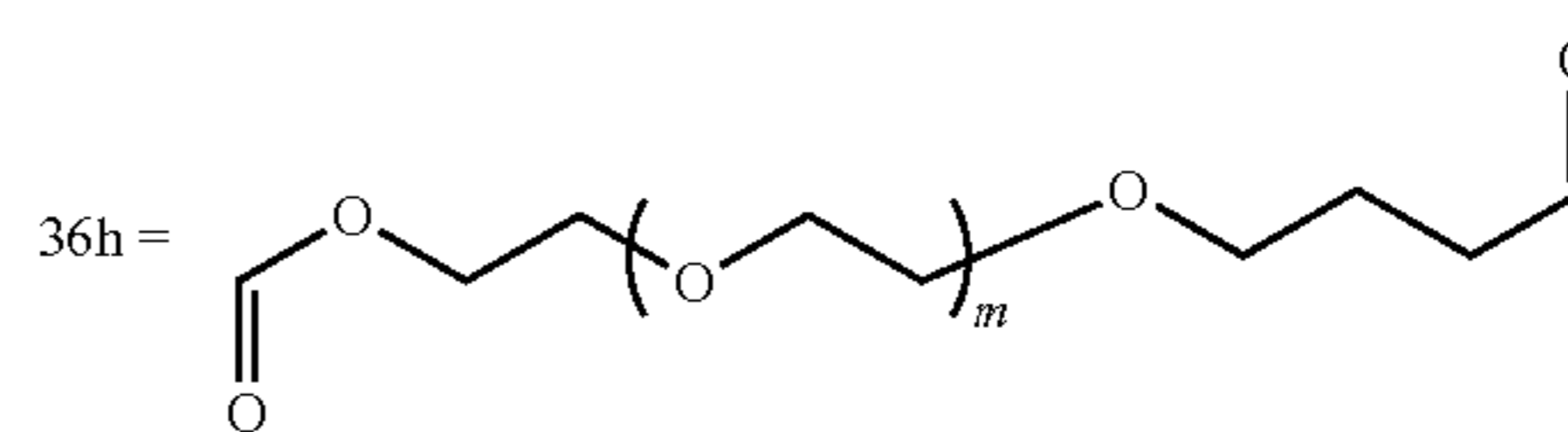
Poly(CDDCys-CB—PEG)
