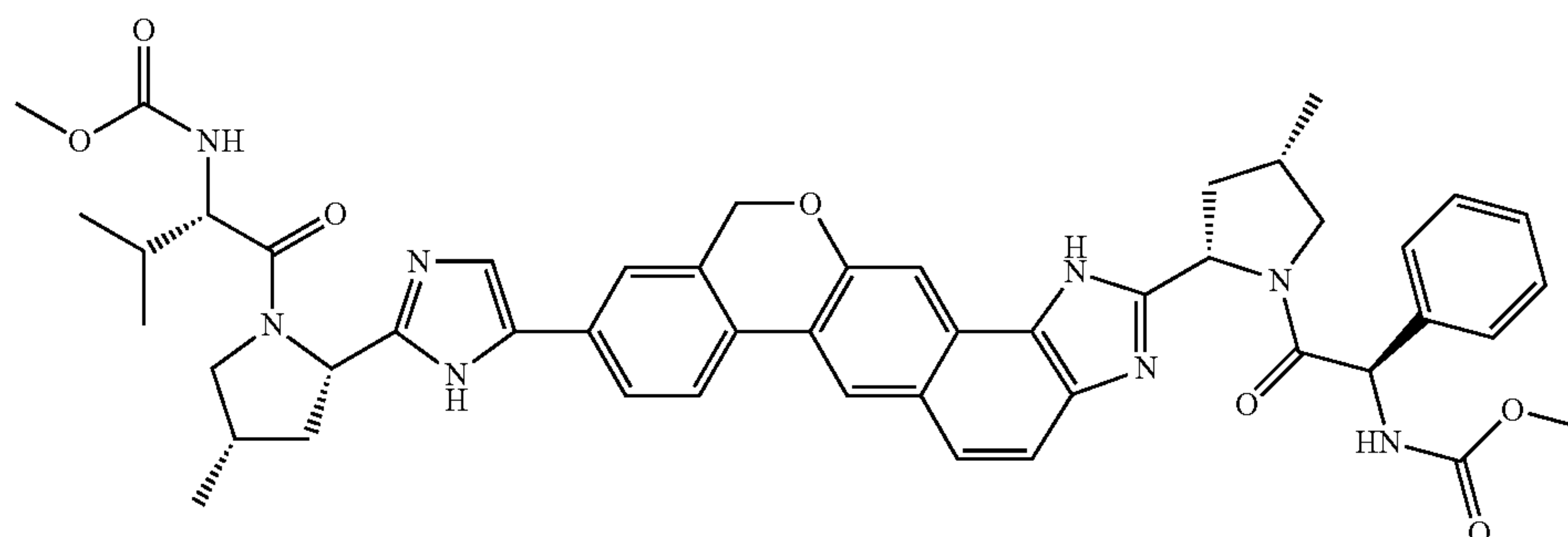
methyl {(2S)-1-[(2S,4S)-2-(5-{2-[(2S,4S)-1-{(2R)-2-[(methoxycarbonyl)amino]-2-phenylacetyl}-4-methylpyrrolidin-2-yl]-1,11-dihydroisochromeno[4',3':6,7]naphtho[1,2-d]imidazol-9-yl}-1H-imidazol-2-yl)-4-methylpyrrolidin-1-yl]-3-methyl-1-oxobutan-2-yl}carbamate
