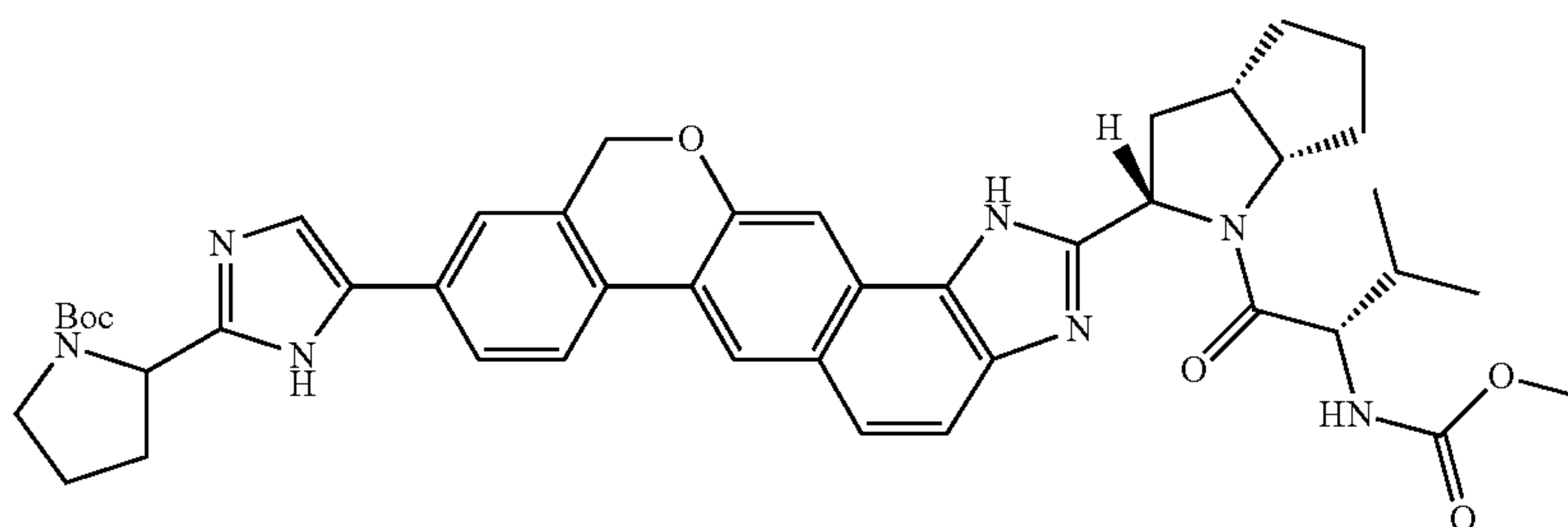
tert-butyl 2-[5-(2-((2S,3aS,6aS)-1-[N-(methoxycarbonyl)-L-valyl]octahydrocyclopenta[b]pyrrol-2-yl)-1,11-dihydroisochromeno[4',3':6,7]naphtho[1,2-d]imidazol-9-yl)-1H-imidazol-2-yl]pyrrolidine-1-carboxylate
