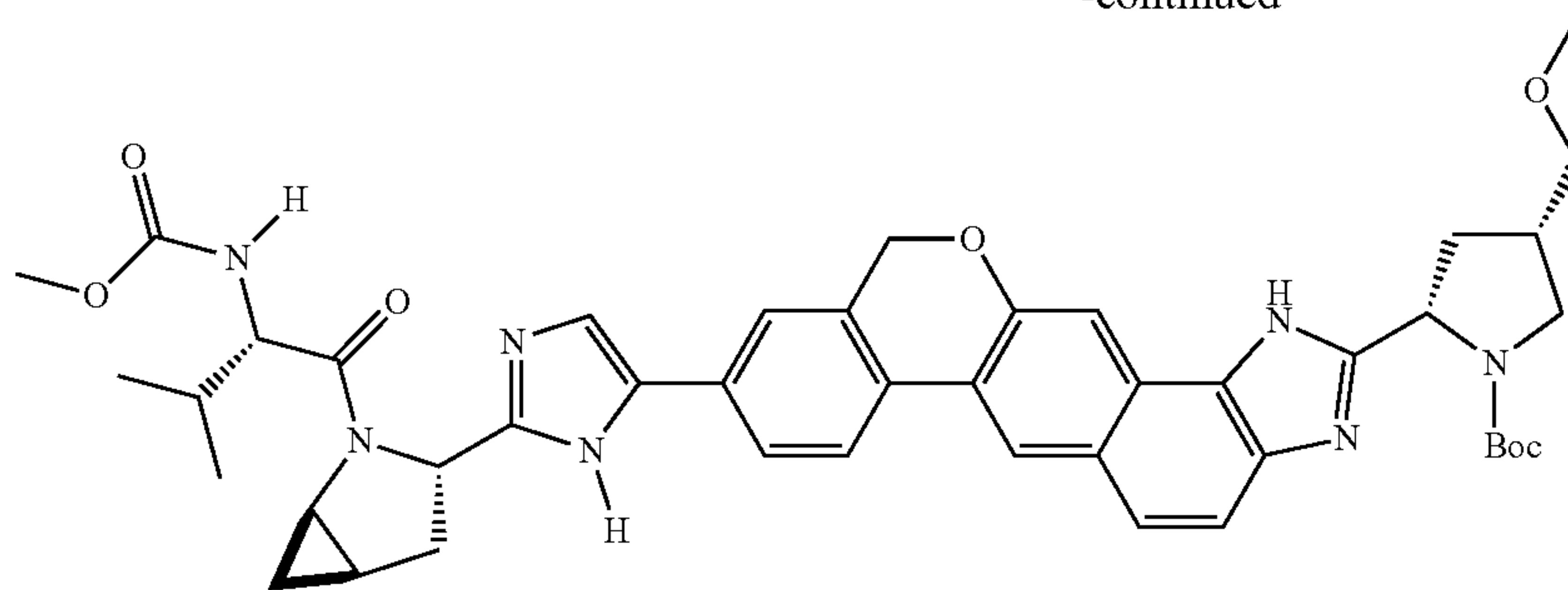
(2S,4S)-tert-butyl 2-(9-(2-((S)-1-((S)-2-(methoxycarbonylamino)-3-methylbutanoyl)azabicyclo[3.1.0]hexan-3-yl)-1H-imidazol-5-yl)-5H-naphtho[c,g]chromeno[8,9-d]imidazol-2-yl)-4-(methoxymethyl)pyrrolidine-1-carboxylate
