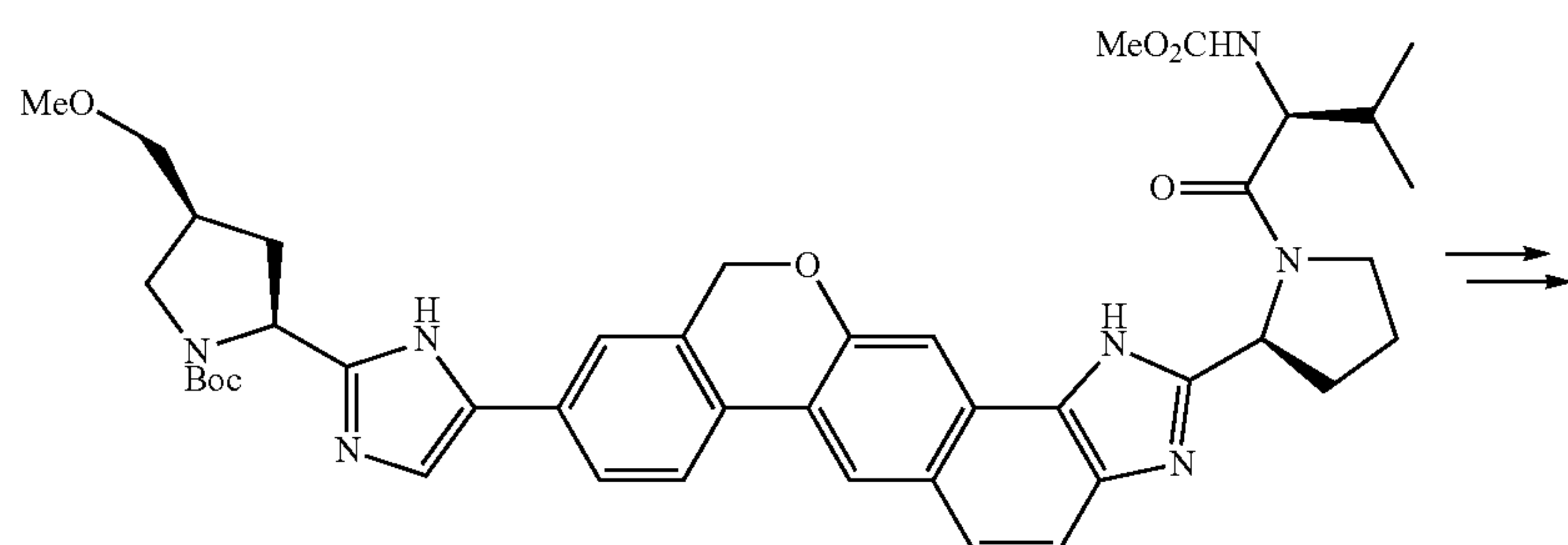
tert-butyl (2S,4S)-2-[5-(2-((2S)-1-[N-(methoxycarbonyl)-L-valyl]pyrrolidin-2-yl)-1,11-dihydroisochromeno[4',3':6,7]naphtho[1,2-d]imidazol-9-yl)-1H-imidazol-2-yl]-4-(methoxymethyl)pyrrolidine-1-carboxylate
