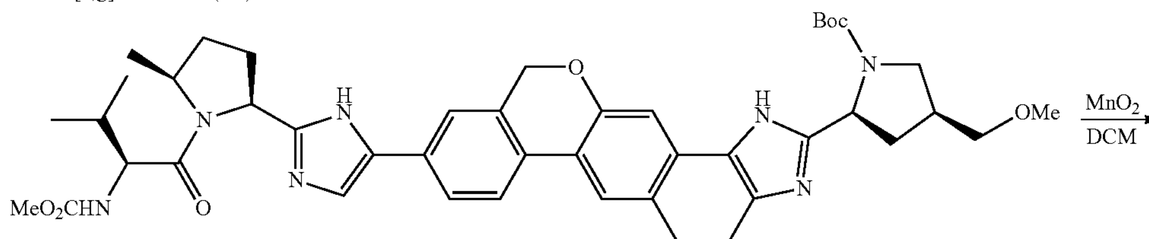
tert-butyl (2S,4S)-2-[9-(2-((2S,5S)-1-[N-(methoxycarbonyl)-L-valyl]-5-methylpyrrolidin-2-yl)-1H-imidazol-5-yl)-1,4,5,11-tetrahydroisochromeno[4',3':6,7]naphtho[1,2-d]imidazol-2-yl]-4-(methoxymethyl)pyrrolidine-1-carboxylate
