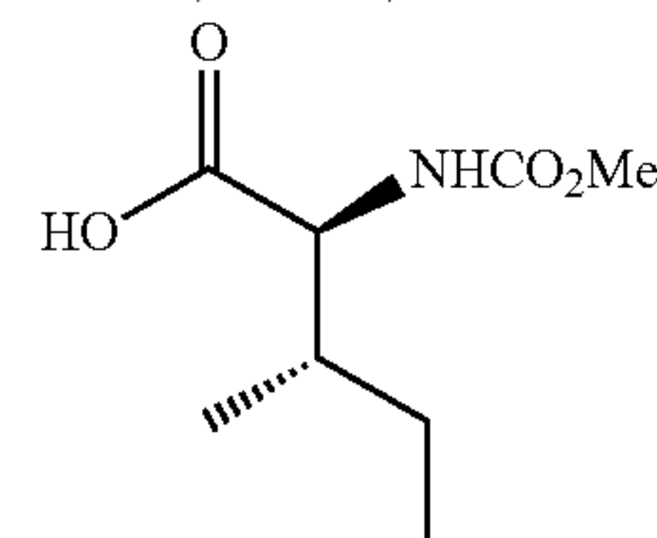
(2S,3S)-2-(methoxycarbonylamino)-3-methylpentanoic acid
