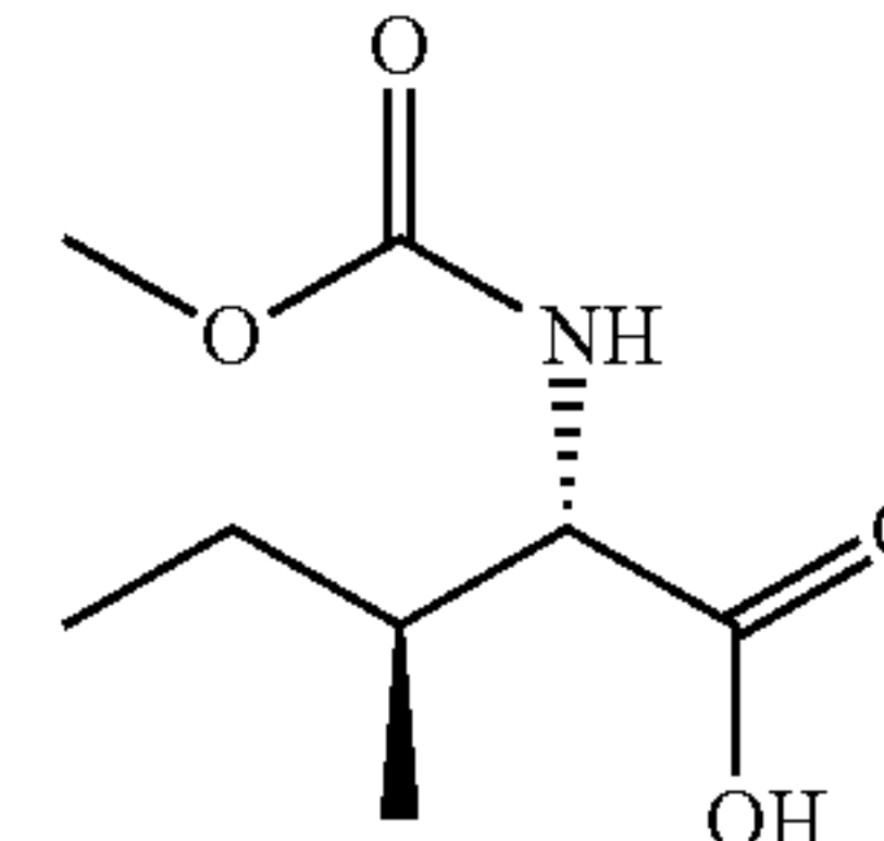
(2S,3S)-2-(methoxycarbonylamino)-3-methylpentanoic acid
