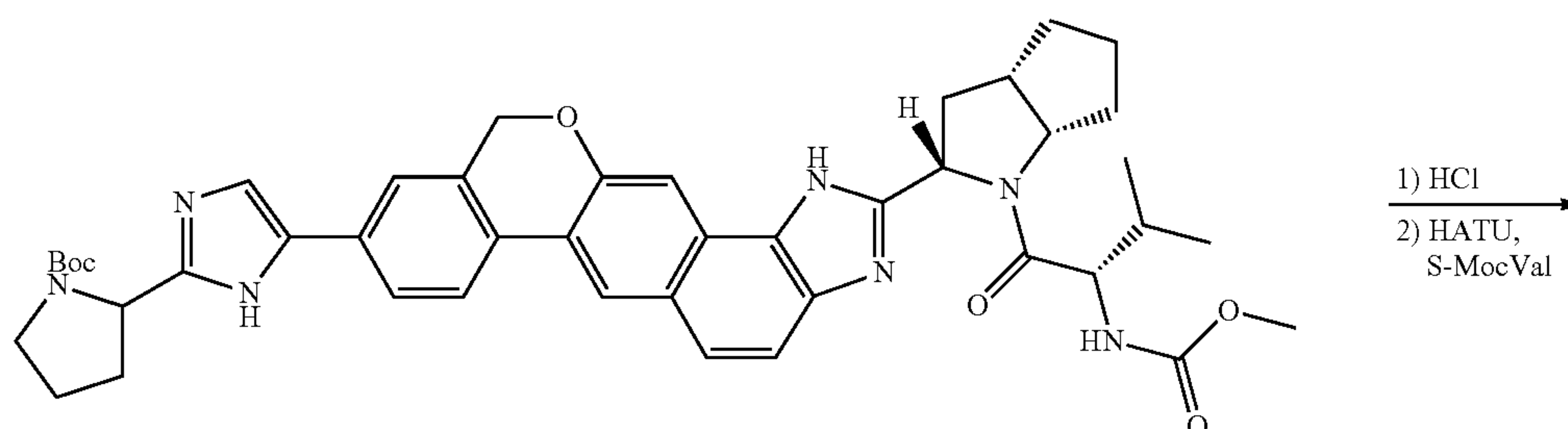
tert-butyl 2-[5-(2-{(2S,3aS,6aS)-1-[N-(methoxycarbonyl)-L-valyl]octahydrocyclopenta[b]pyrrol-2-yl]-1,11-dihydroisochromeno[4',3':6,7]naphtho[1,2-d]imidazol-9-yl)-1H-imidazol-2-yl]pyrrolidine-1-carboxylate
