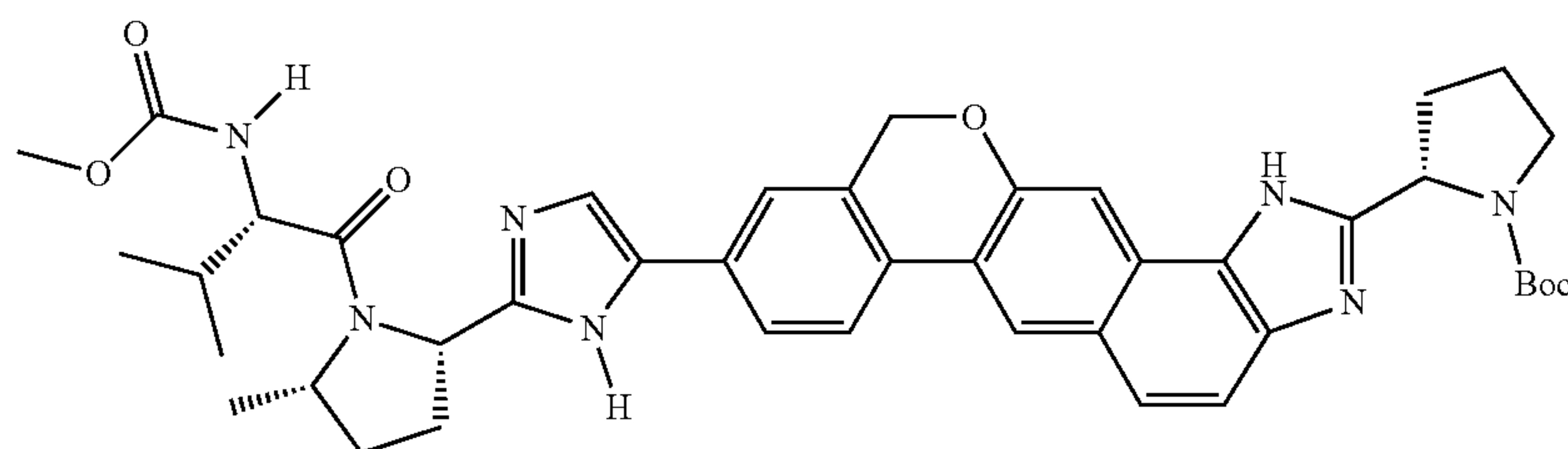
tert-butyl (2S)-2-[9-(2-{(2S,5S)-1-[N-(methoxycarbonyl)-L-valyl]-5-methylpyrrolidin-2-yl]-1H-imidazol-5-yl)-3,11-dihydroisochromeno[4',3':6,7]naphtho[1,2-d]imidazol-2-yl]pyrrolidine-1-carboxylate
