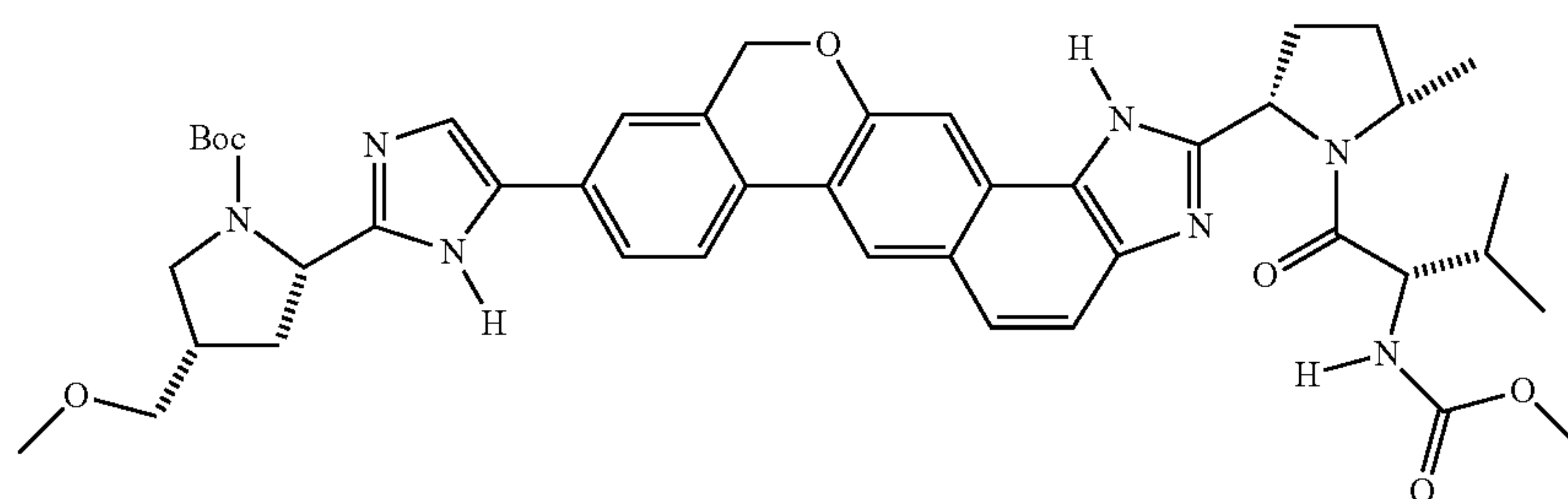
tert-butyl (2S,4S)-2-[5-(2-((2S,5S)-1-[N-(methoxycarbonyl)-L-valyl]-5-methylpyrrolidin-2-yl)-1,11-dihydroisochromeno[4',3':6,7]naphtho[1,2-d]imidazol-9-yl)-1H-imidazol-2-yl]-4-(methoxymethyl)pyrrolidine-1-carboxylate
