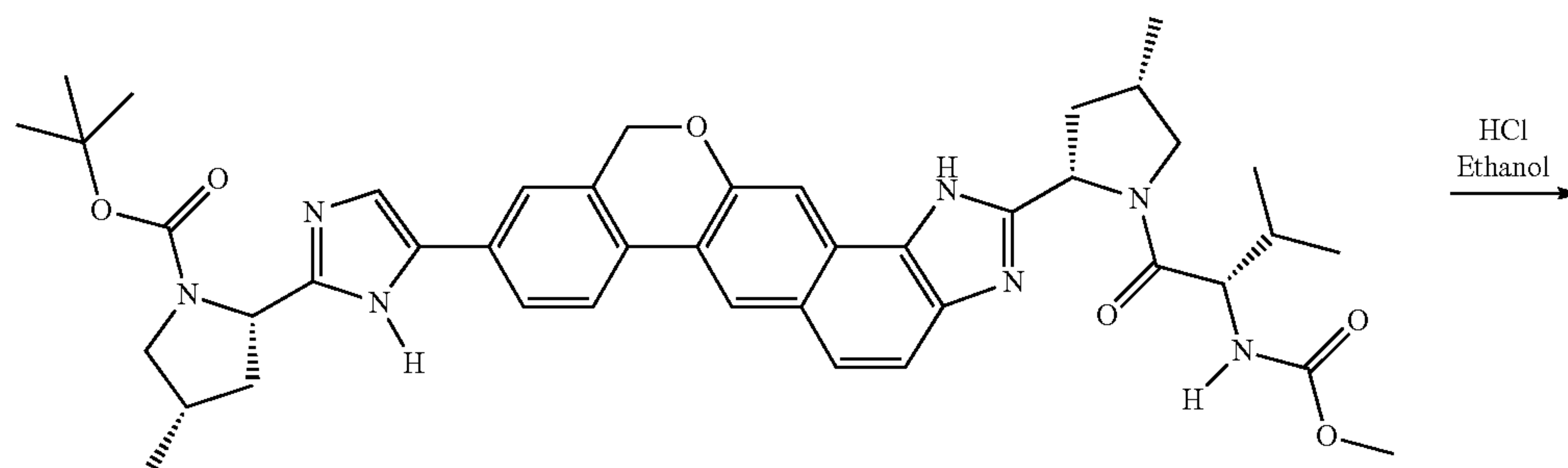
tert-butyl (2S,4S)-2-[5-(2-{(2S,4S)-1-[N-(methoxycarbonyl)-L-valyl]-4-methylpyrrolidin-2-yl]-1,11-dihydroisochromeno[4',3':6,7]naphtho[1,2-d]imidazol-9-yl)-1H-imidazol-2-yl]-4-methylpyrrolidine-1-carboxylate
