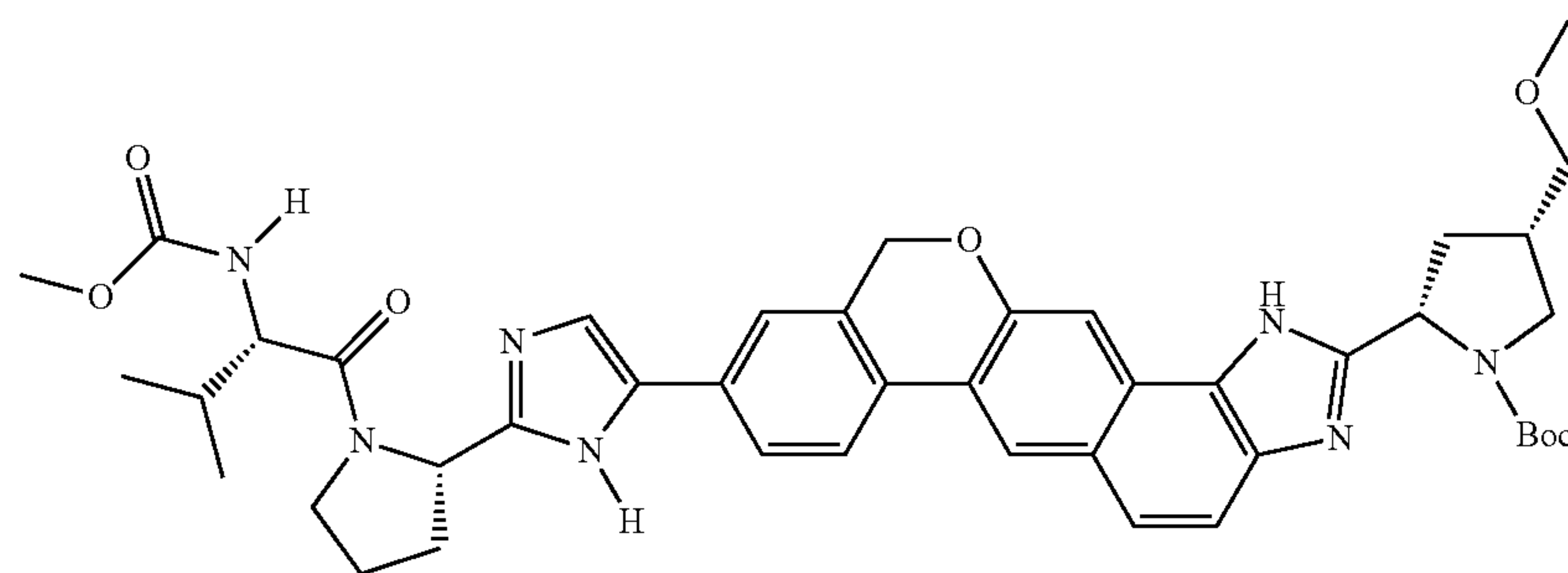
(2S,4S)-tert-butyl 2-(9-(2-(((S)-1-((S)-2-(methoxycarbonylamino)-3-methylbutanoyl)pyrrolidin-2-yl)-1H-imidazol-5-yl)-5H-naphtho[c,g]chromeno[8,9-d]imidazol-2-yl)-4-(methoxymethyl)pyrrolidine-1-carboxylate
