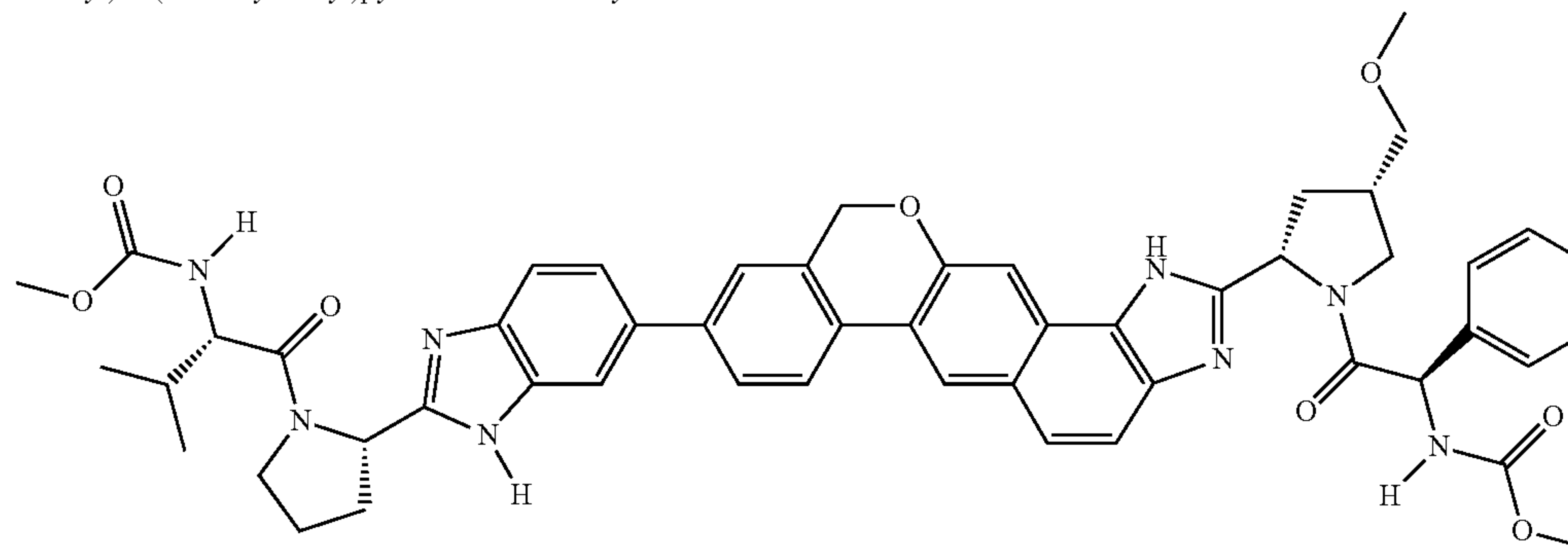
(2S,4S)-tert-butyl 2-(9-(2-((S)-1-((S)-2-(methoxycarbonylamino)-3-methylbutanoyl)pyrrolidin-2-yl)-1H-benzo[d]imidazol-6-yl)-1,11-dihydroisochromeno[4',3':6,7]naphtho[1,2-d]imidazol-2-yl)-4-(methoxymethyl)pyrrolidine-1-carboxylate
