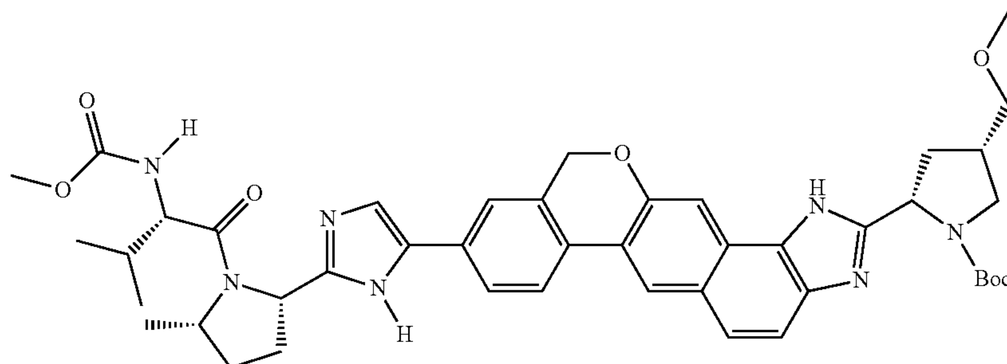
tert-butyl (2S,4S)-2-[9-(2-((2S,5S)-1-[N-(methoxycarbonyl)-L-valyl]-5-methylpyrrolidin-2-yl)-1H-imidazol-5-yl)-3,11-dihydroisochromeno[4',3':6,7]naphtho[1,2-d]imidazol-2-yl]-4-(methoxymethyl)pyrrolidine-1-carboxylate
