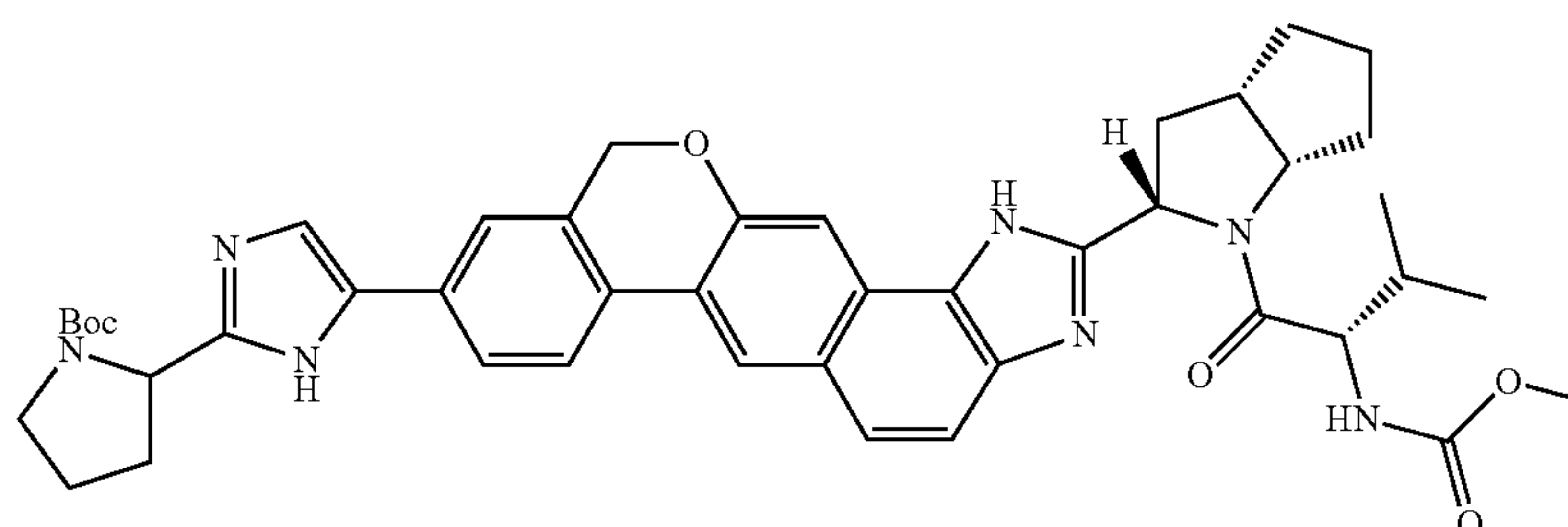
tert-butyl 2-[5-(2-{(2S,3aS,6aS)-1-[N-(methoxycarbonyl)-L-valyl]octahydrocyclopenta[b]pyrrol-2-yl]-1,11-dihydroisochromeno[4',3':6,7]naphtho[1,2-d]imidazol-9-yl)-1H-imidazol-2-yl]pyrrolidine-1-carboxylate
