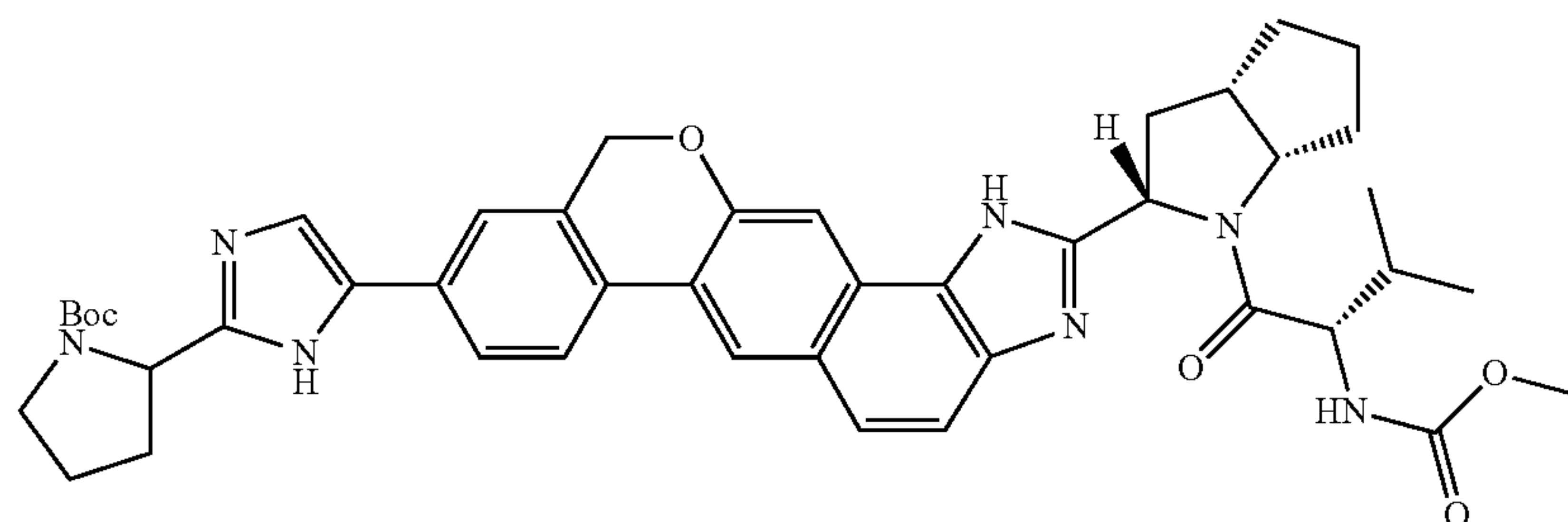
tert-butyl 2-[5-(2-((2S,3aS,6aS)-1-[N-(methoxycarbonyl)-L-valyl]octahydrocyclopenta[b]pyrrol-2-yl)-1,11-dihydroisochromeno[4',3':6,7]naphtho[1,2-d]imidazol-9-yl)-1H-imidazol-2-yl]pyrrolidine-1-carboxylate
