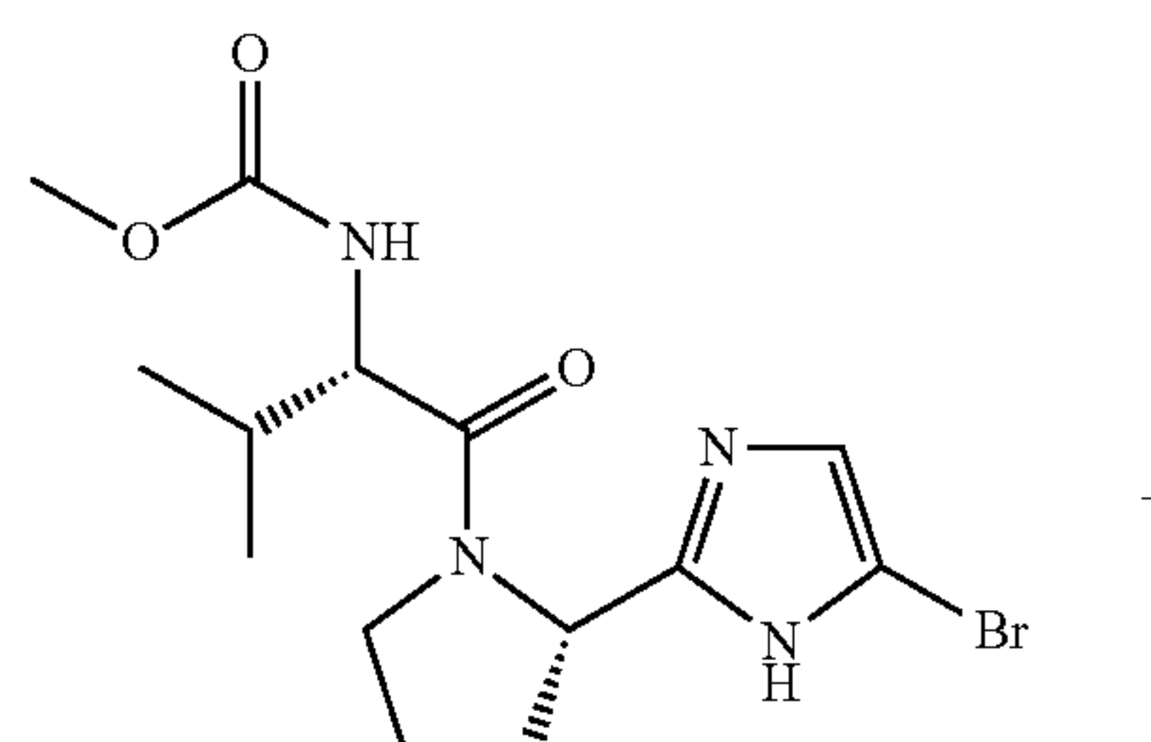
methyl(S)-1-((S)-2-(5-bromo-1H-imidazol-2-yl)pyrrolidin-1-yl)-3-methyl-1-oxobutan-2-ylcarbamate
