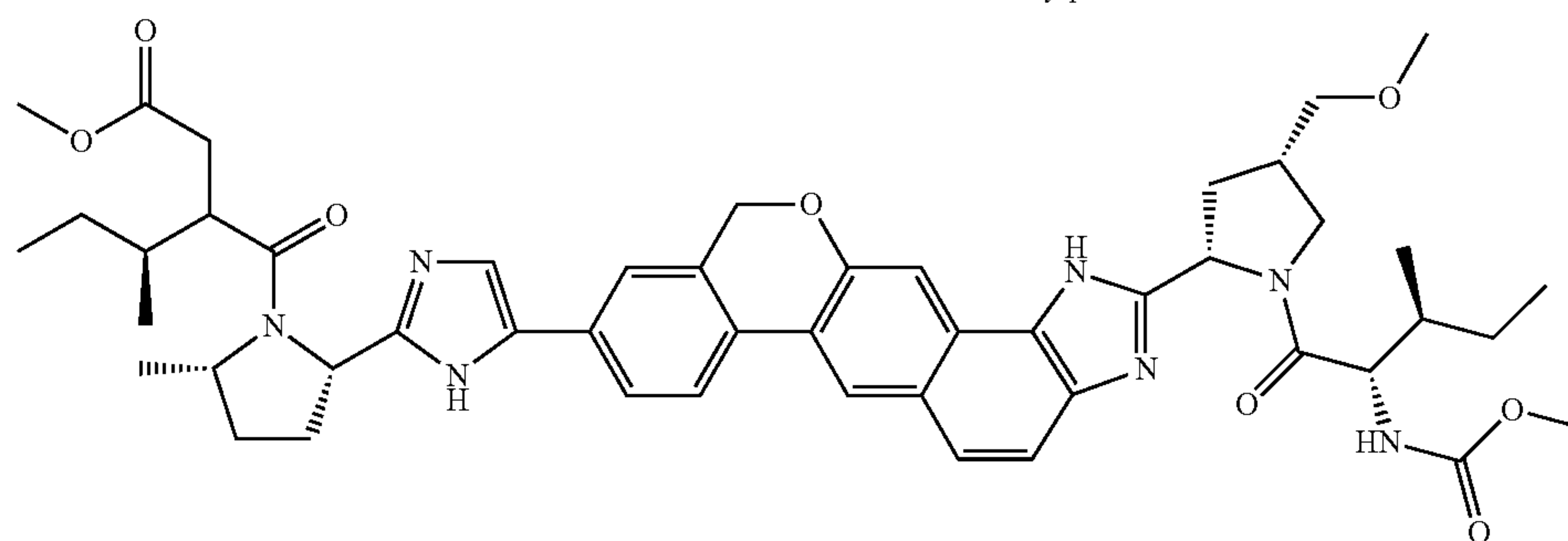
(2S,3S)-2-(methoxycarbonylamino)-3-methylpentanoic acid
