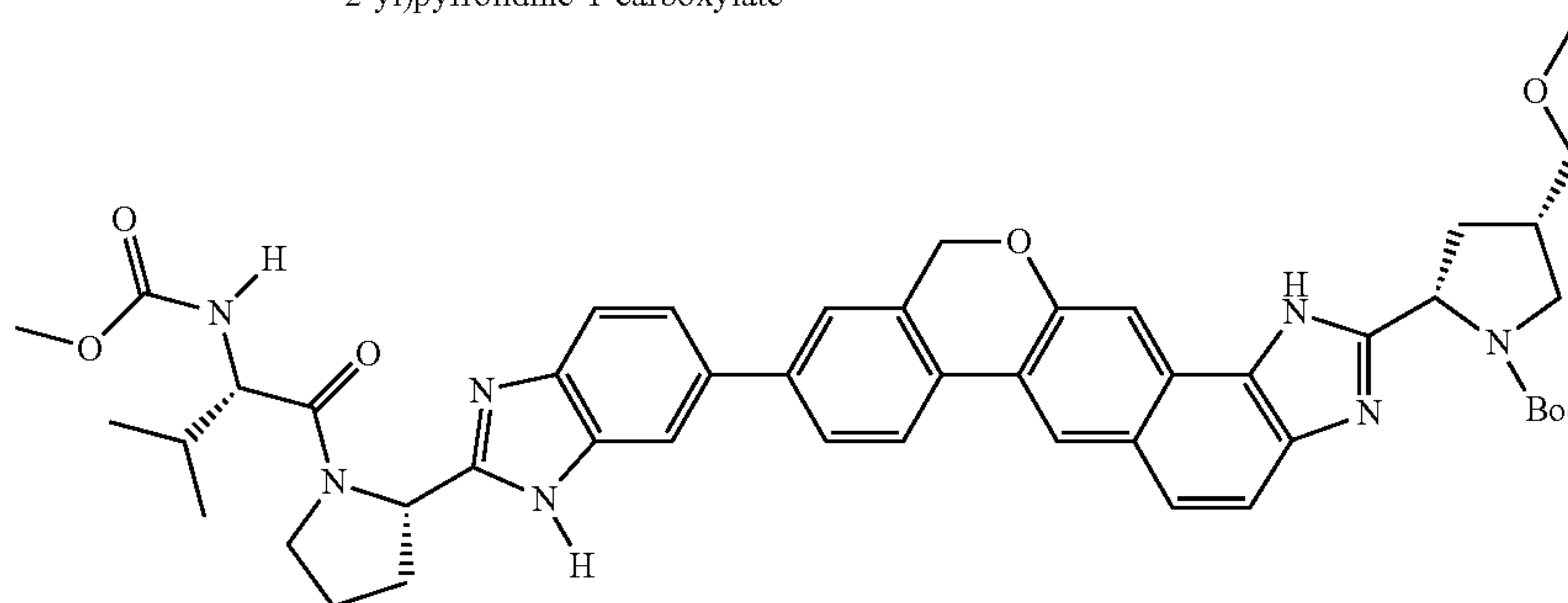
(2S,4S)-tert-butyl 2-(9-(2-((S)-1-((S)-2-(methoxycarbonylamino)-3-methylbutanoyl)pyrrolidin-2-yl)-1H-benzo[d]imidazol-6-yl)-1,11-dihydroisochromeno[4',3':6,7]naphtho[1,2-d]imidazol-2-yl)-4-(methoxymethyl)pyrrolidine-1-carboxylate
