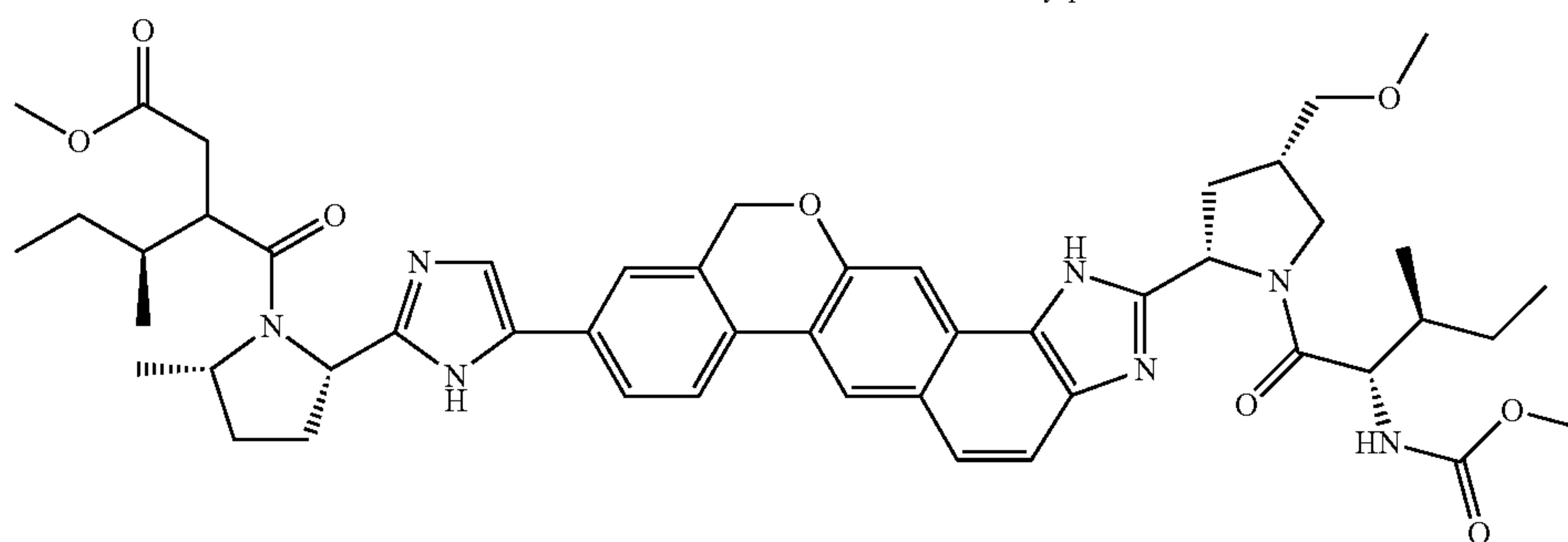
(2S,3S)-2-(methoxycarbonylamino)-3-methylpentanoic acid
