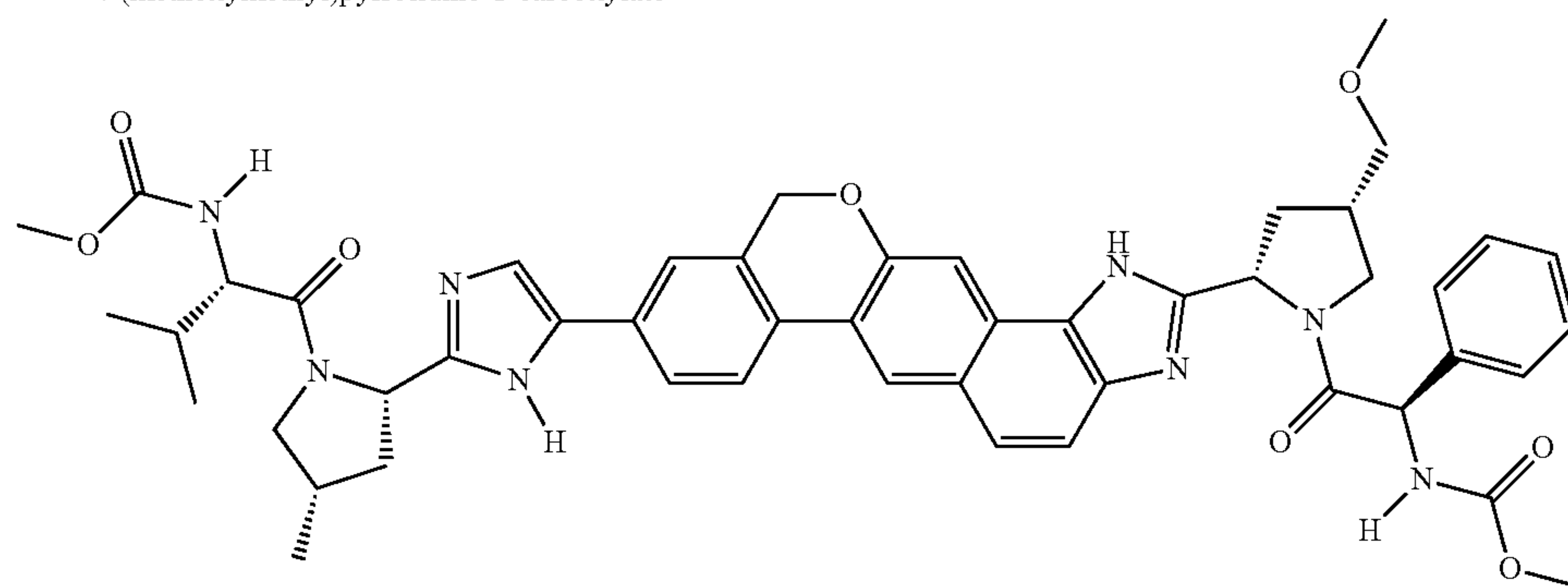
tert-butyl (2S,4S)-2-[9-(2-((2S,4S)-1-[N-(methoxycarbonyl)-L-valyl]-4-methylpyrrolidin-2-yl)-1H-imidazol-5-yl)-3,11-dihydroisochromeno[4',3':6,7]naphtho[1,2-d]imidazol-2-yl]-4-(methoxymethyl)pyrrolidine-1-carboxylate
