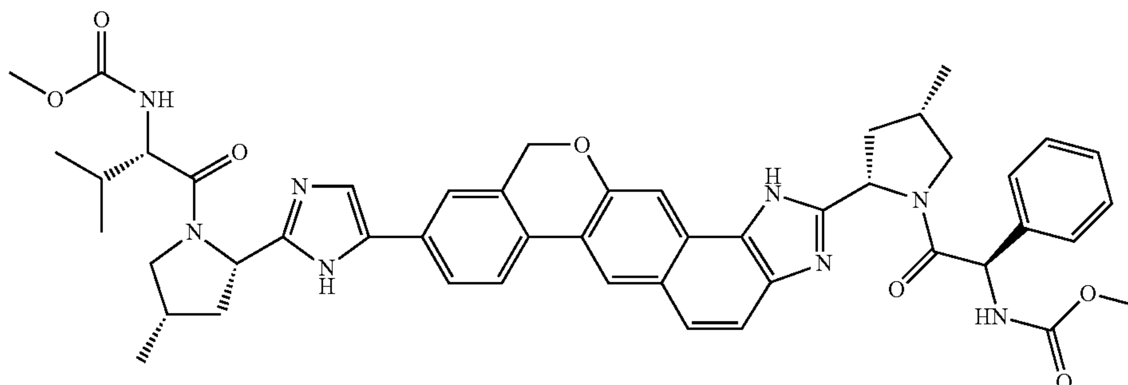
methyl {(2S)-1-[(2S,4S)-2-(5-{2-[(2S,4S)-1-{(2R)-2-[(methoxycarbonyl)amino]-2-phenylacetyl}-4-methylpyrrolidin-2-yl]-1,11-dihydroisochromeno[4',3':6,7]naphtho[1,2-d]imidazol-9-yl}-1H-imidazol-2-yl)-4-methylpyrrolidin-1-yl]-3-methyl-1-oxobutan-2-yl}carbamate
