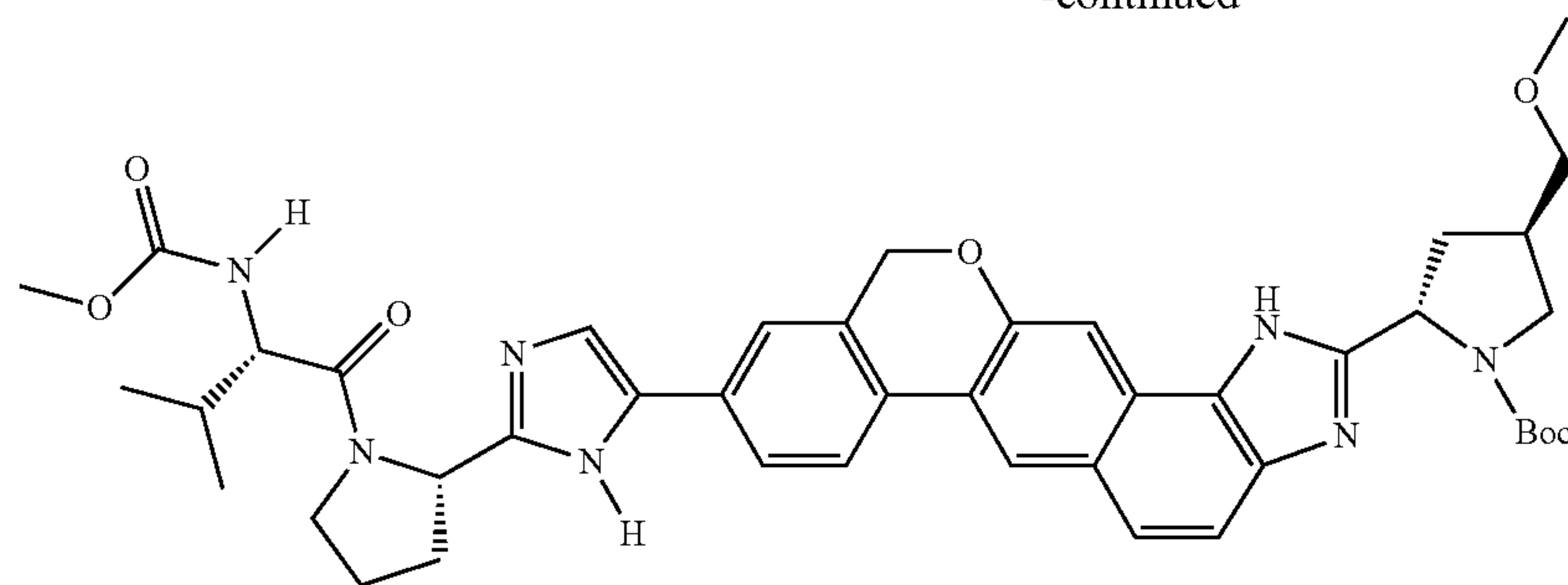
(2S,4R)-tert-butyl 2-(9-(2-((S)-1-((S)-2-(methoxycarbonylamino)-3-methylbutanoyl)pyrrolidin-2-yl)-1H-imidazol-5-yl)-1,11-dihydroisochromeno[4',3':6,7]naphtho[1,2-d]imidazol-2-yl)-4-(methoxymethyl)pyrrolidine-1-carboxylate
