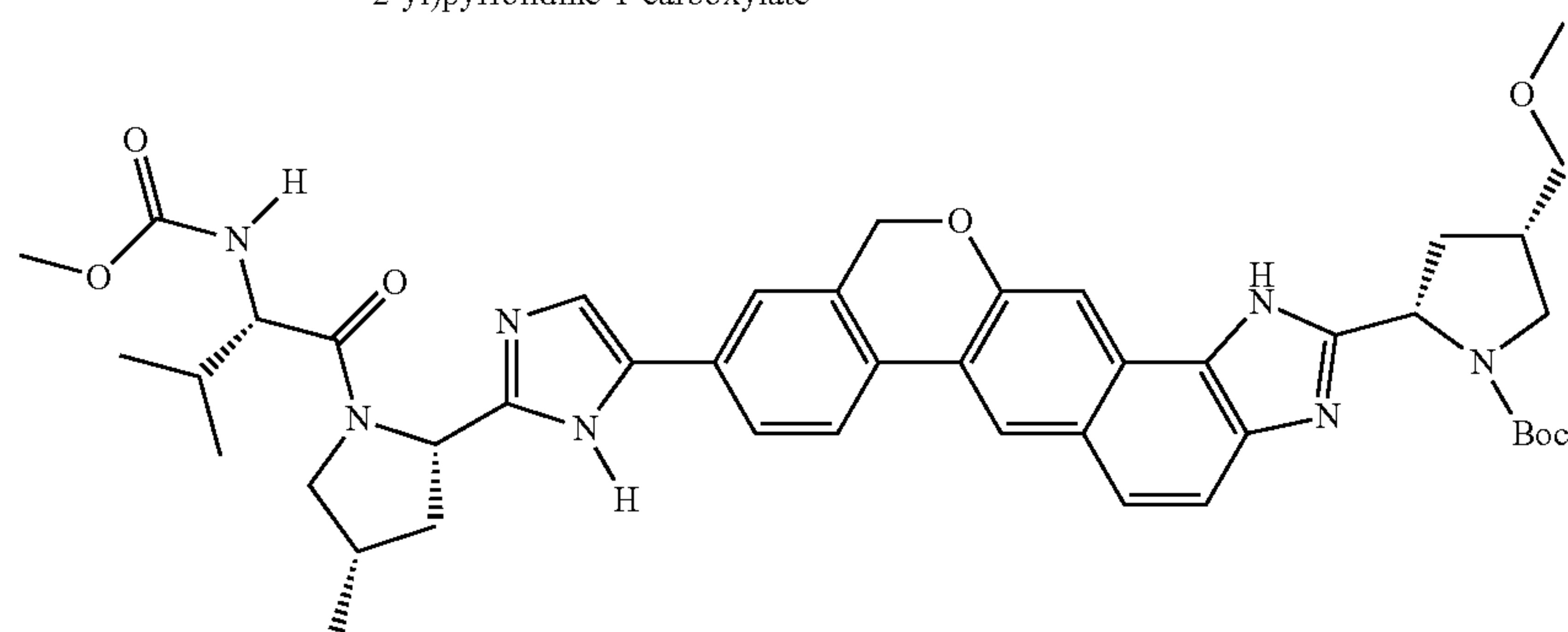
tert-butyl (2S,4S)-2-[9-(2-((2S,4S)-1-[N-(methoxycarbonyl)-L-valyl]-4-methylpyrrolidin-2-yl)-1H-imidazol-5-yl)-3,11-dihydroisochromeno[4',3':6,7]naphtho[1,2-d]imidazol-2-yl]-4-(methoxymethyl)pyrrolidine-1-carboxylate
