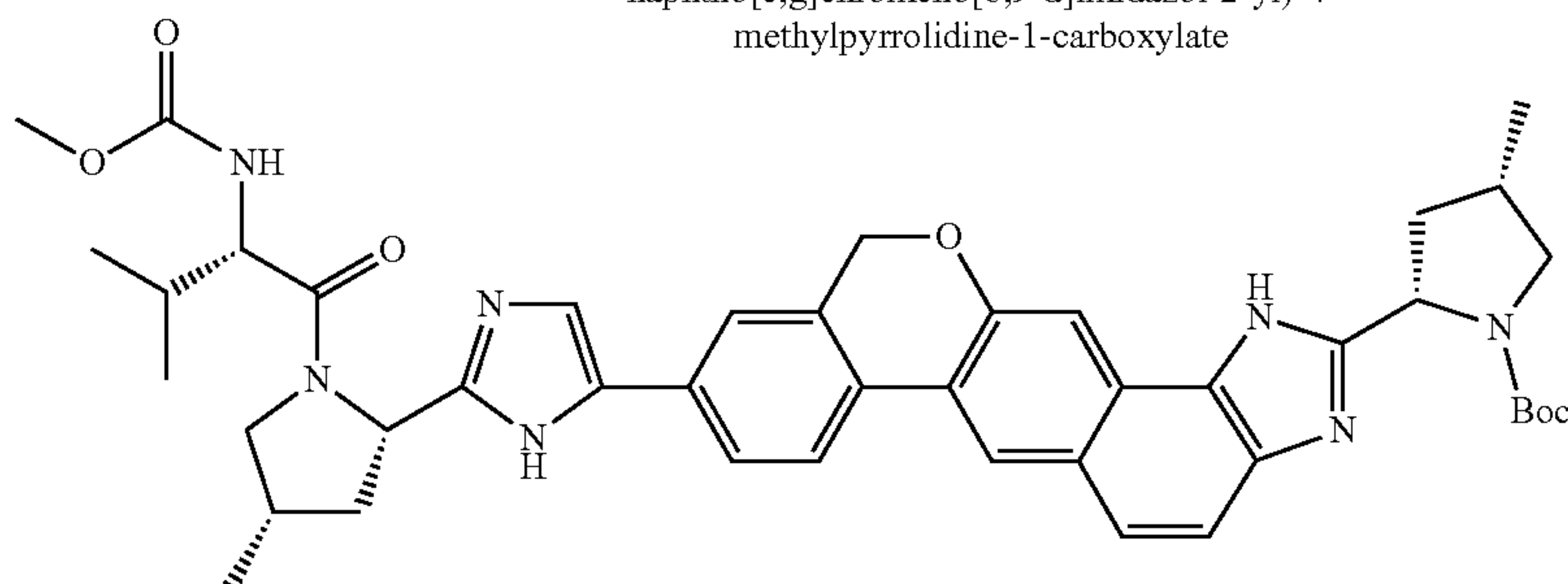
tert-butyl (2S,4S)-2-[9-(2-((2S,4S)-1-[N-(methoxycarbonyl)-L-valyl]-4-methylpyrrolidin-2-yl)-1H-imidazol-5-yl)-1,11-dihydroisochromeno[4',3':6,7]naphtho[1,2-d]imidazol-2-yl)-4-methylpyrrolidine-1-carboxylate
