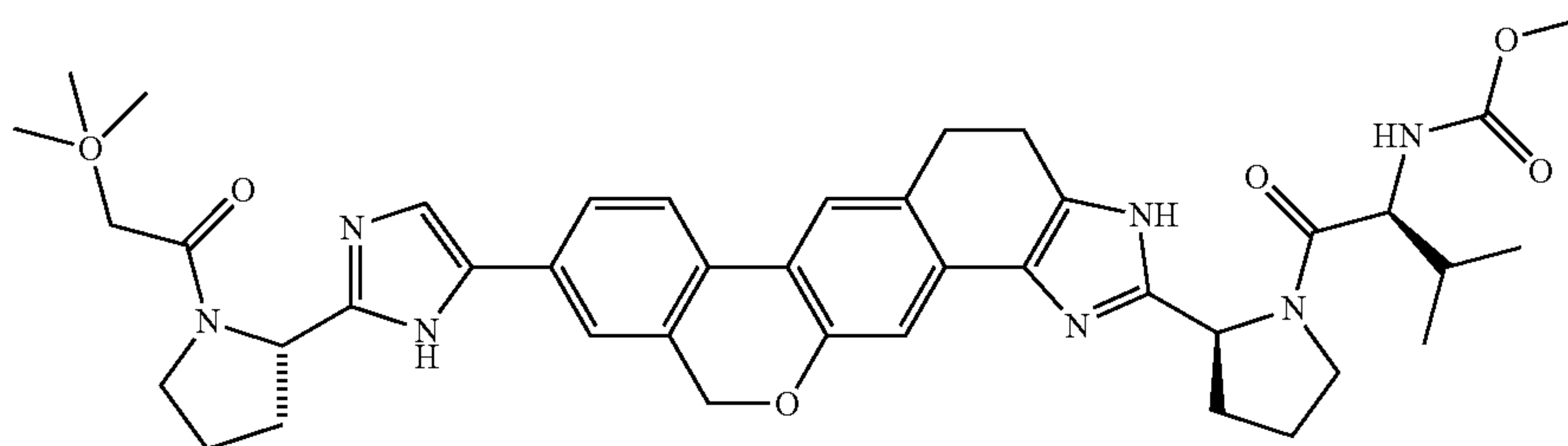
tert-butyl (2R)-2-[5-(2-((2S)-1-[N-(methoxycarbonyl)-L-valyl]pyrrolidin-2-yl)-3,4,5,11-tetrahydroisochromeno[4',3':6,7]naphtho[1,2-d]imidazol-9-yl)-1H-imidazol-2-yl]pyrrolidine-1-carboxylate
