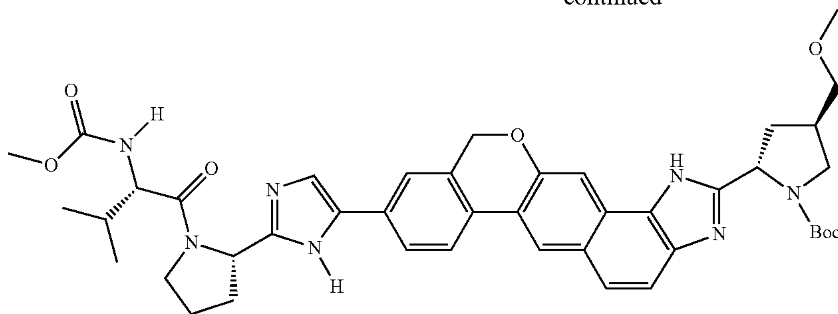
(2S,4R)-tert-butyl 2-(9-(2-((S)-1-((S)-2-(methoxycarbonylamino)-3-methylbutanoyl)pyrrolidin-2-yl)-1H-imidazol-5-yl)-1,11-dihydroisochromeno[4',3':6,7]naphtho[1,2-d]imidazol-2-yl)-4-(methoxymethyl)pyrrolidine-1-carboxylate
