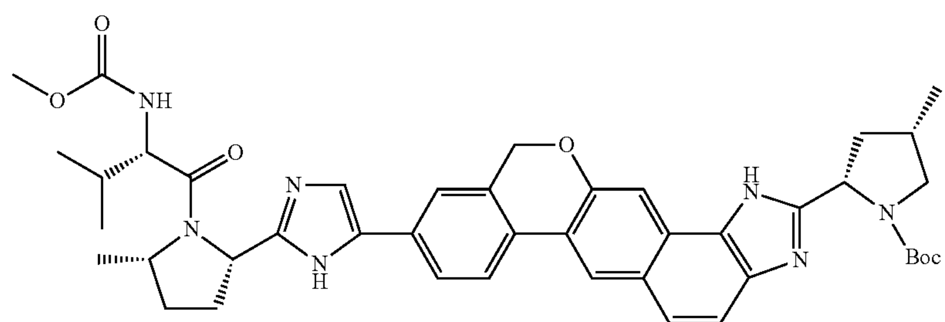
tert-butyl (2S,4S)-2-[9-(2-{(2S,4S)-1-[N-(methoxycarbonyl)-L-valyl]-5-methylpyrrolidin-2-yl}-1H-imidazol-5-yl)-1,11-dihydroisochromeno[4',3':6,7]naphtho[1,2-d]imidazol-2-yl]-4-methylpyrrolidine-1-carboxylate
