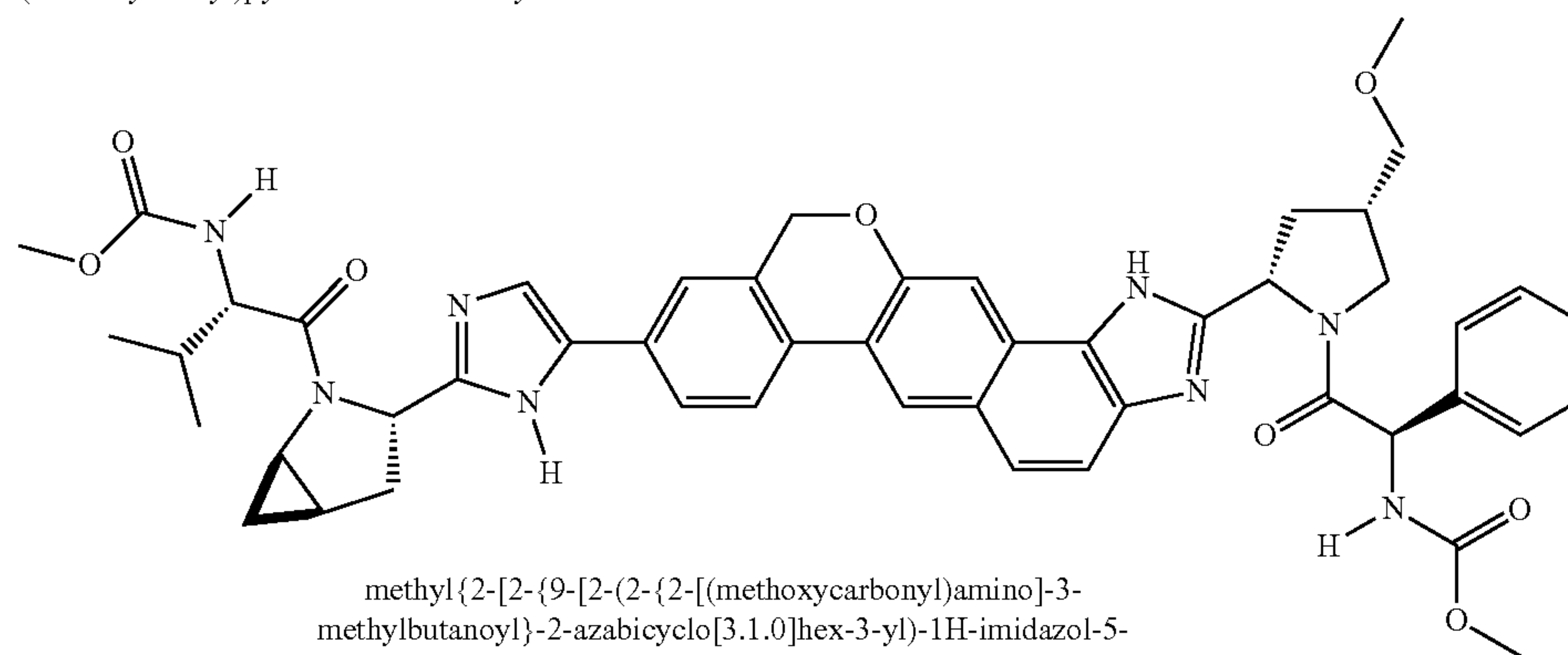
(2S,4S)-tert-butyl 2-(9-(2-((S)-1-((S)-2-(methoxycarbonylamino)-3-methylbutanoyl)azabicyclo[3.1.0]hexan-3-yl)-1H-imidazol-5-yl)-5H-naphtho[c,g]chromeno[8,9-d]imidazol-2-yl)-4-(methoxymethyl)pyrrolidine-1-carboxylate
