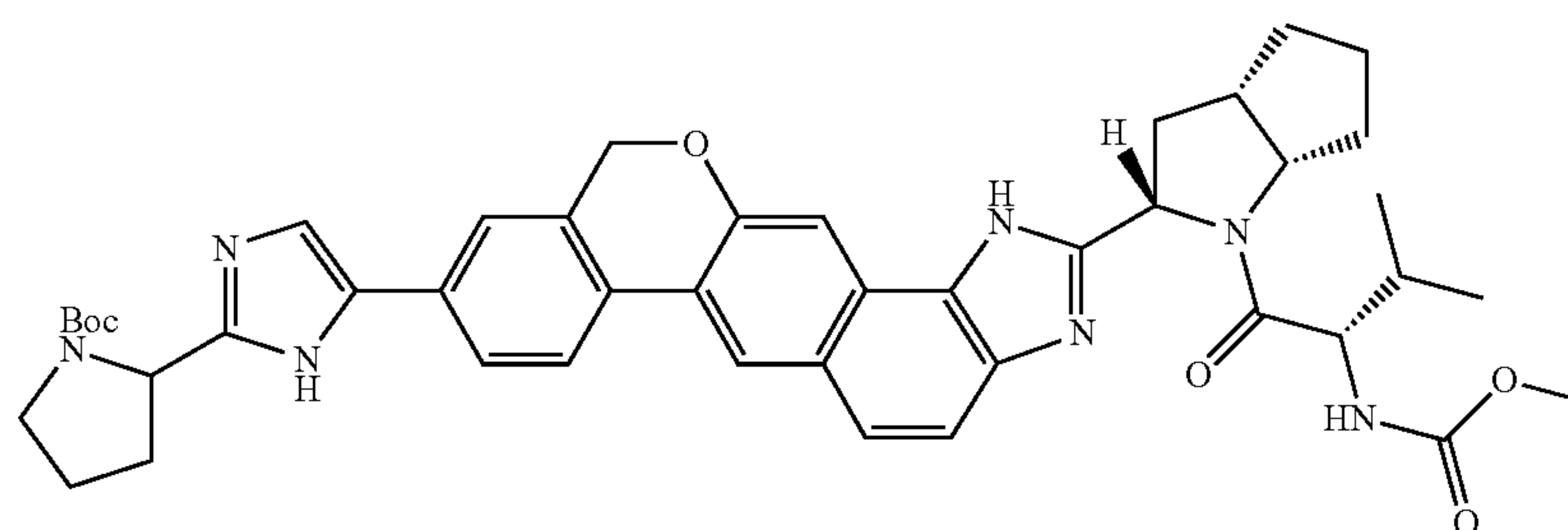
tert-butyl 2-[5-(2-((2S,3aS,6aS)-1-[N-(methoxycarbonyl)-L-valyl]octahydrocyclopenta[b]pyrrol-2-yl)-1,11-dihydroisochromeno[4',3':6,7]naphtho[1,2-d]imidazol-9-yl)-1H-imidazol-2-yl]pyrrolidine-1-carboxylate
