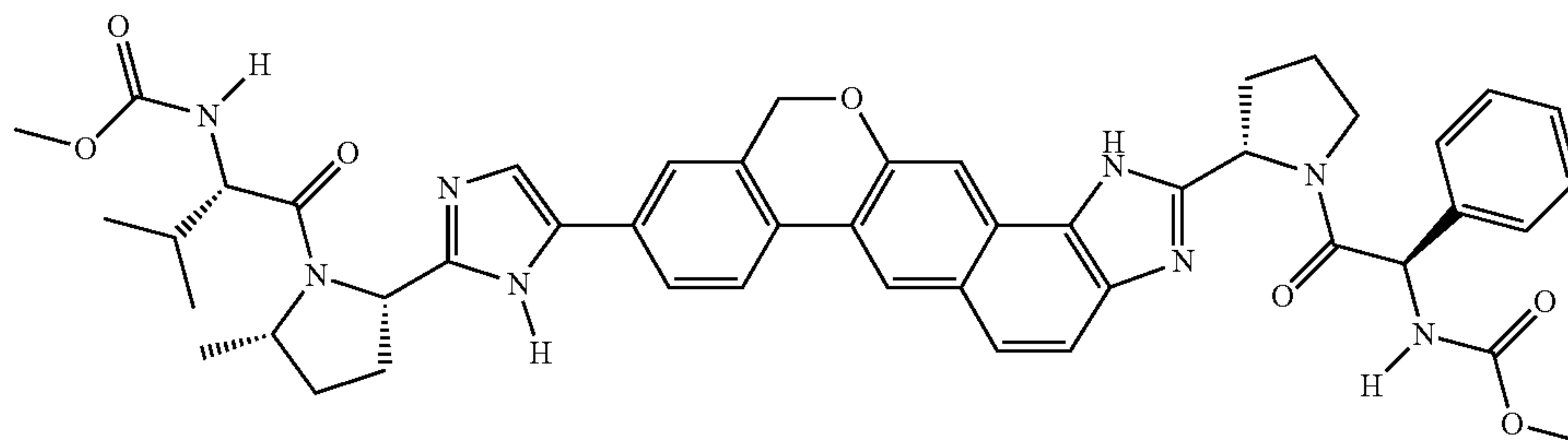
methyl {(2S)-1-[(2S,5S)-2-(5-{2-[(2S)-1-[(2R)-2-[(methoxycarbonyl)amino]-2-phenylacetyl]pyrrolidin-2-yl]-1,11-dihydroisochromeno[4',3':6,7]naphtho[1,2-d]imidazol-9-yl}-1H-imidazol-2-yl)-5-methylpyrrolidin-1-yl]-3-methyl-1-oxobutan-2-yl} carbamate
