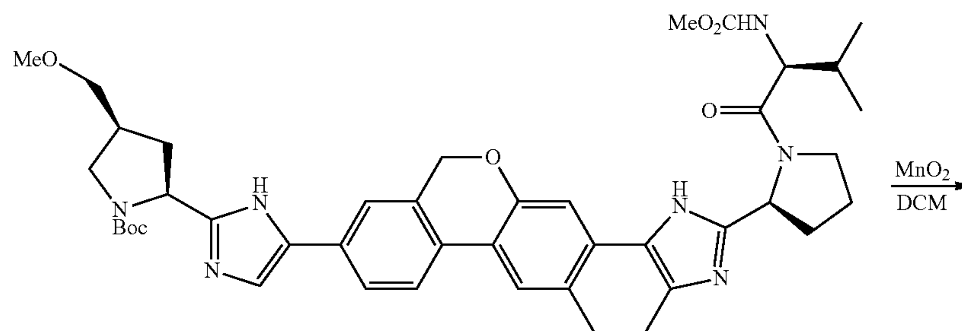
tert-butyl (2S,4S)-2-[5-(2-((2S)-1-[N-(methoxycarbonyl)-L-valyl]pyrrolidin-2-yl)-1,4,5,11-tetrahydroisochromeno[4',3':6,7]naphtho[1,2-d]imidazol-9-yl)-1H-imidazol-2-yl]-4-(methoxymethyl)pyrrolidine-1-carboxylate
