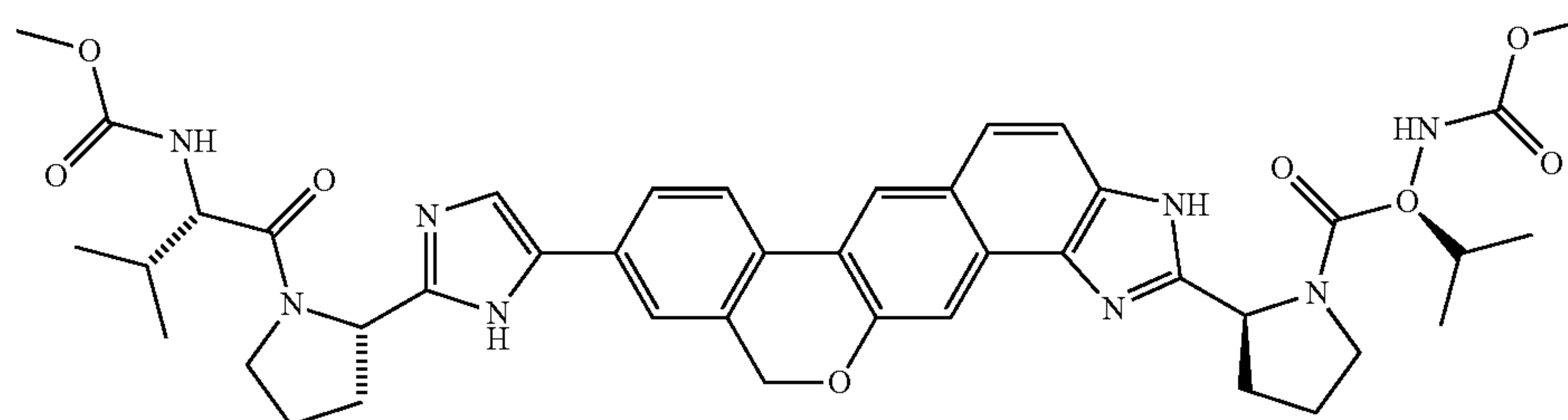
dimethyl (2S,2'S)-1,1'-((2S,2'S)-2,2'l-pyrrolidin-2-yl)-5H-naphtho[c,g]chromeno[8,9-d]imidazol-9-yl)-1H-imidazol-2-yl)pyrrolidin-1-yl))bis(3-methyl-1-oxobutane-2,1-diyl)dicarbamate
