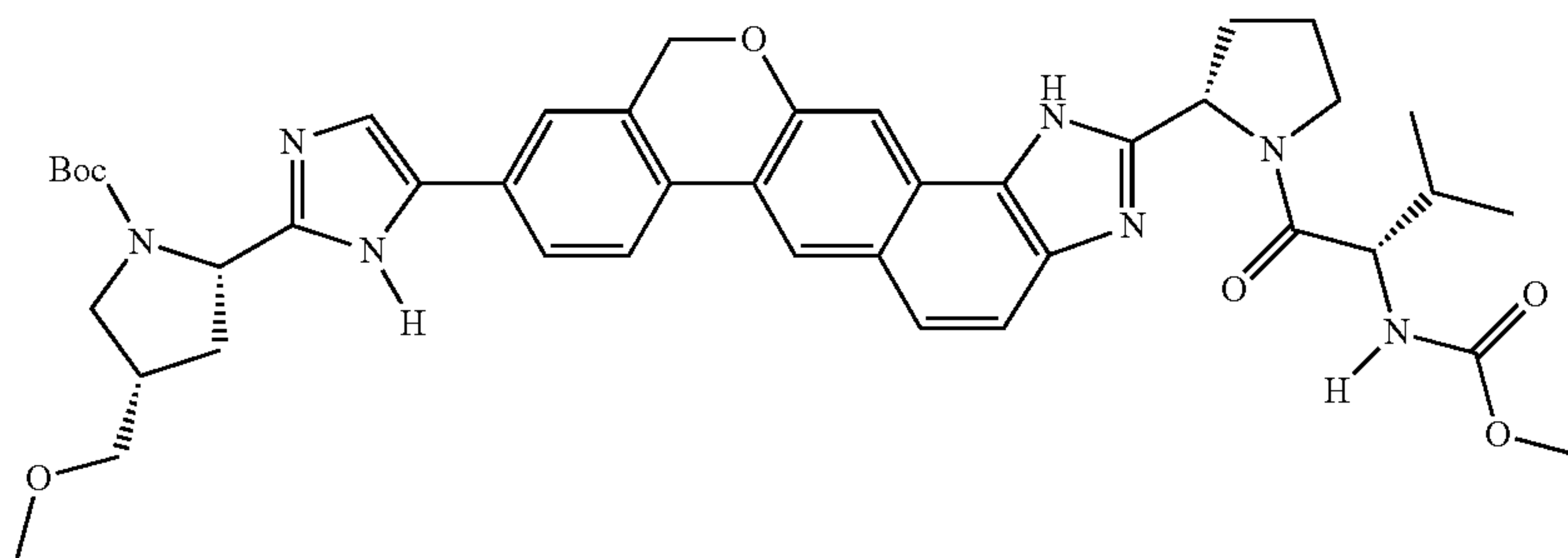
tert-butyl (2S,4S)-2-[5-(2-((2S,4S)-1-[N-(methoxycarbonyl)-L-valyl]-pyrrolidin-2-yl)-1,11-dihydroisochromeno[4',3':6,7]naphtho[1,2-d]imidazol-9-yl)-1H-imidazol-2-yl]-4-(methoxymethyl)pyrrolidine-1-carboxylate
