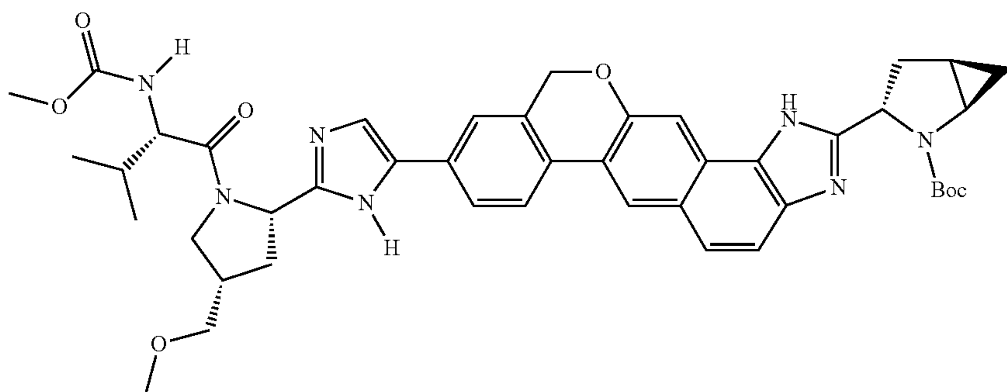
(1R,3S,5R)-tert-butyl 3-(9-(2-((S)-1-((S)-2-(methoxycarbonylamino)-3-methylbutanoyl)-4-methoxymethylpyrrolidin-2-yl)-1H-imidazol-5-yl)-1,11-dihydroisochromeno[4',3':6,7]naphtho[1,2-d]imidazol-2-yl)-2-azabicyclo[3.1.0]hexane-2-carboxylate
