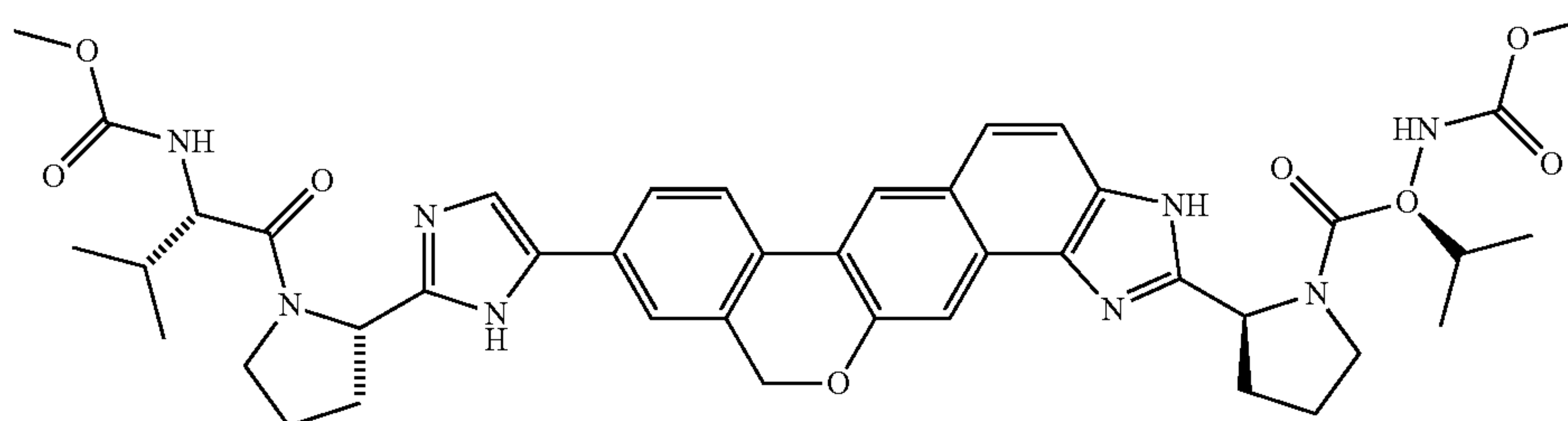
dimethyl (2S,2'S)-1,1'-((2S,2'S)-2,2'1-pyrrolidin-2-yl)-5H-naphtho[c,g]chromeno[8,9-d]imidazol-9-yl)-1H-imidazol-2-yl)pyrrolidin-1-yl))bis(3-methyl-1-oxobutane-2,1-diyl)dicarbamate
