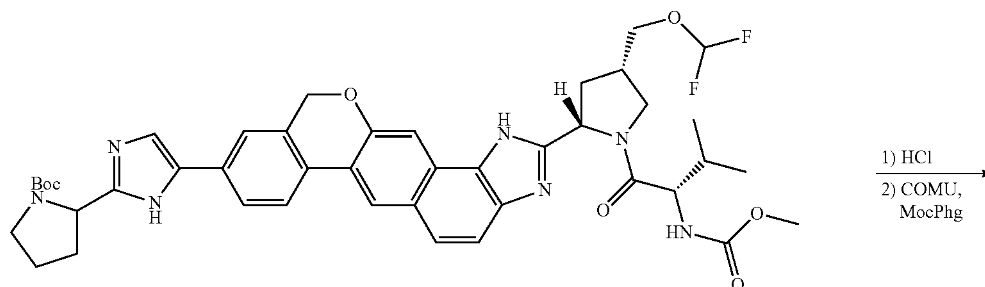
tert-butyl 2-[5-(2-((2S,4S)-4-((difluoromethoxy)methyl)-1-[N-(methoxycarbonyl)-L-valyl]pyrrolidin-2-yl)-1,11-dihydroisochromeno[4',3':6,7]naphtho[1,2-d]imidazol-9-yl)-1H-imidazol-2-yl]pyrrolidine-1-carboxylate
