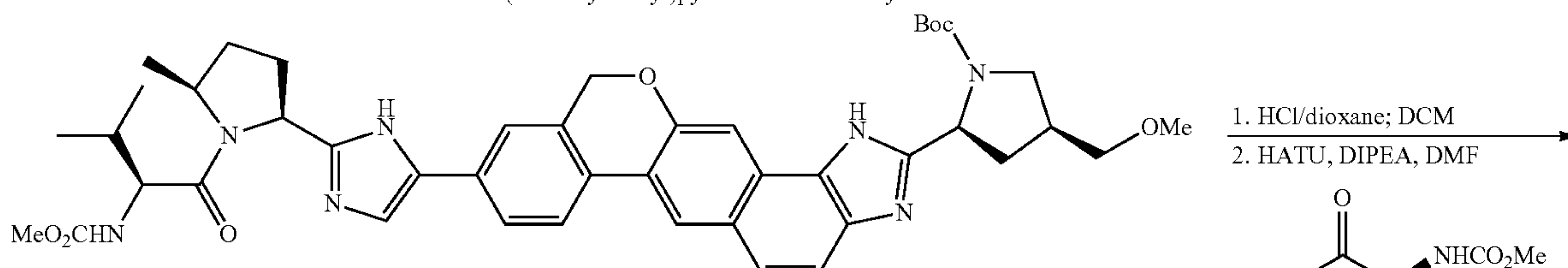
tert-butyl (2S,4S)-2-[9-(2-((2S,5S)-1-[N-(methoxycarbonyl)-L-valyl]-5-methylpyrrolidin-2-yl)-1H-imidazol-5-yl)-1,11-dihydroisochromeno[4',3':6,7]naphtho[1,2-d]imidazol-2-yl]-4-(methoxymethyl)pyrrolidine-1-carboxylate
