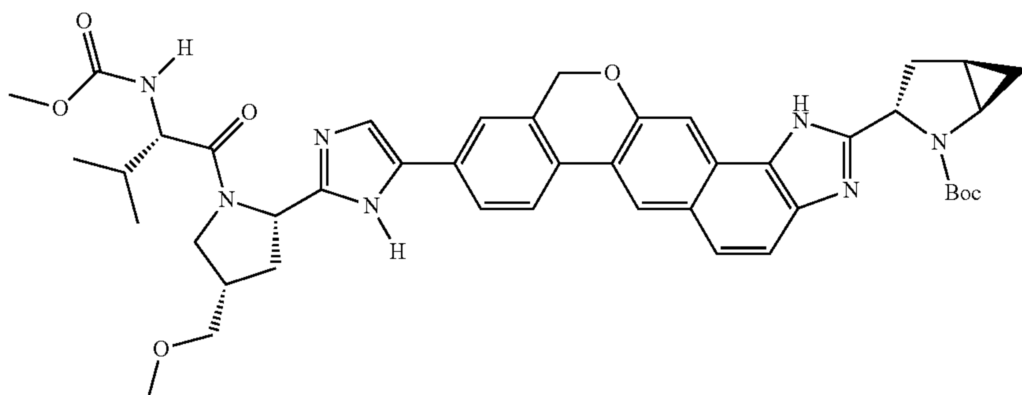
(1R,3S,5R)-tert-butyl 3-(9-(2-((S)-1-((S)-2-(methoxycarbonylamino)-3-methylbutanoyl)-4-methoxymethylpyrrolidin-2-yl))-1H-imidazol-5-yl))-1,11-dihydroisochromeno[4',3':6,7]naphtho[1,2-d]imidazol-2-yl)-2-azabicyclo[3.1.0]hexane-2-carboxylate
