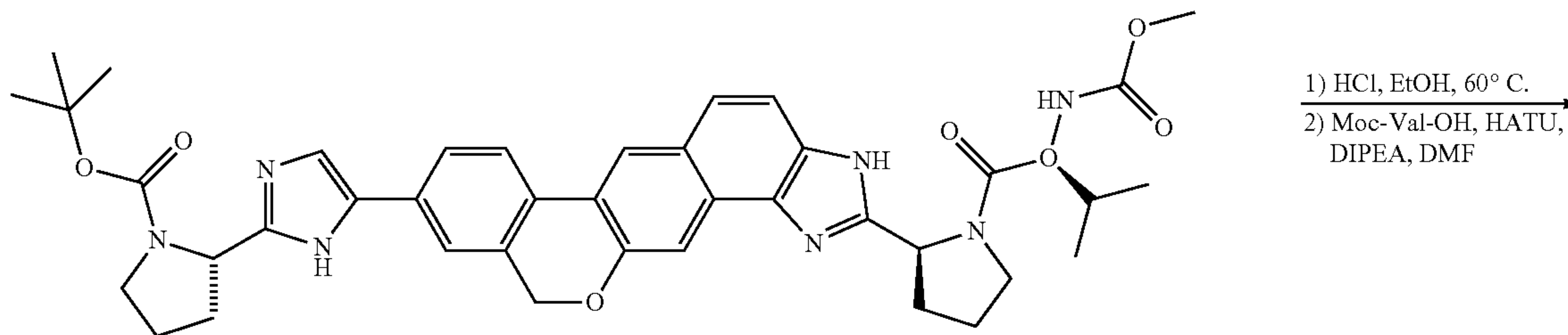
tert-butyl (2R)-2-[5-(2-((2S)-1-[N-(methoxycarbonyl)-L-valyl]pyrrolidin-2-yl)-3,11-dihydroisochromeno[4',3':6,7]naphtho[1,2-d]imidazol-9-yl)-1H-imidazol-2-yl]pyrrolidine-1-carboxylate
