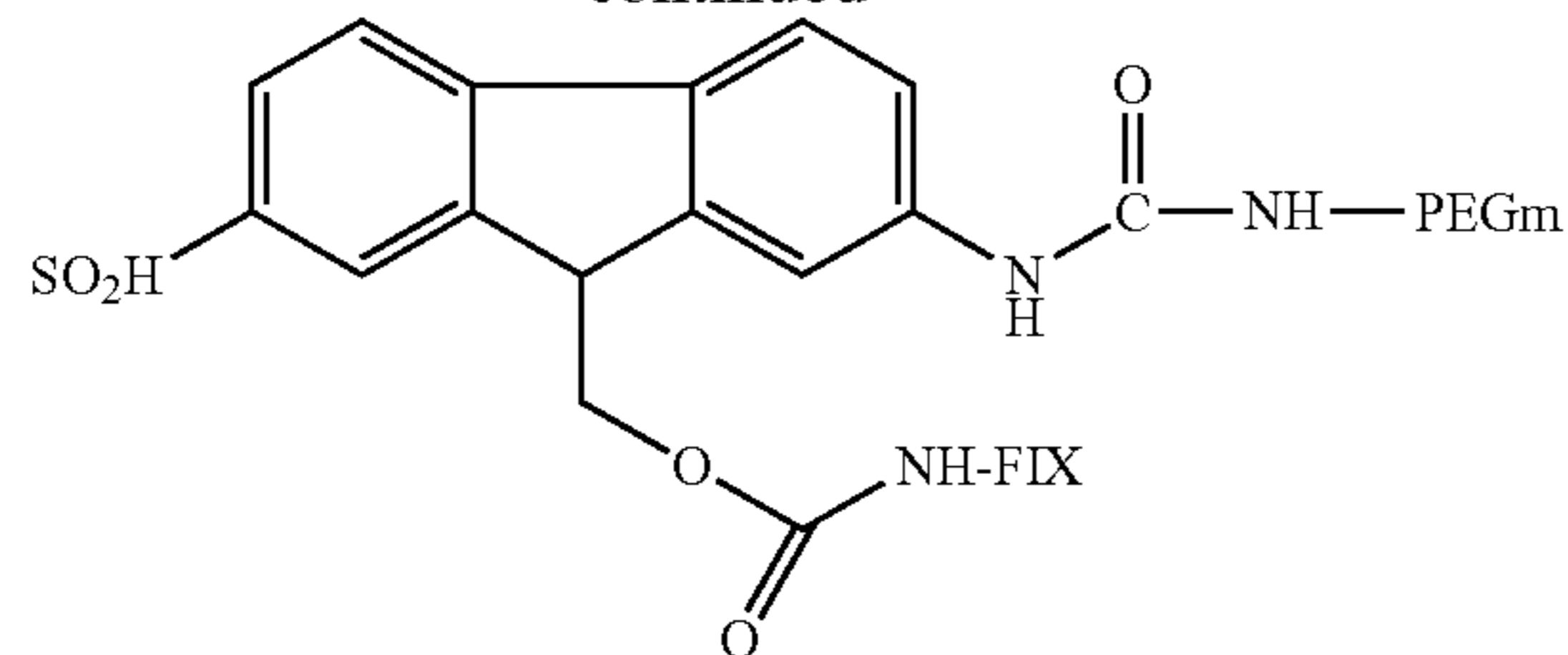
FIX Conjugate #4A
