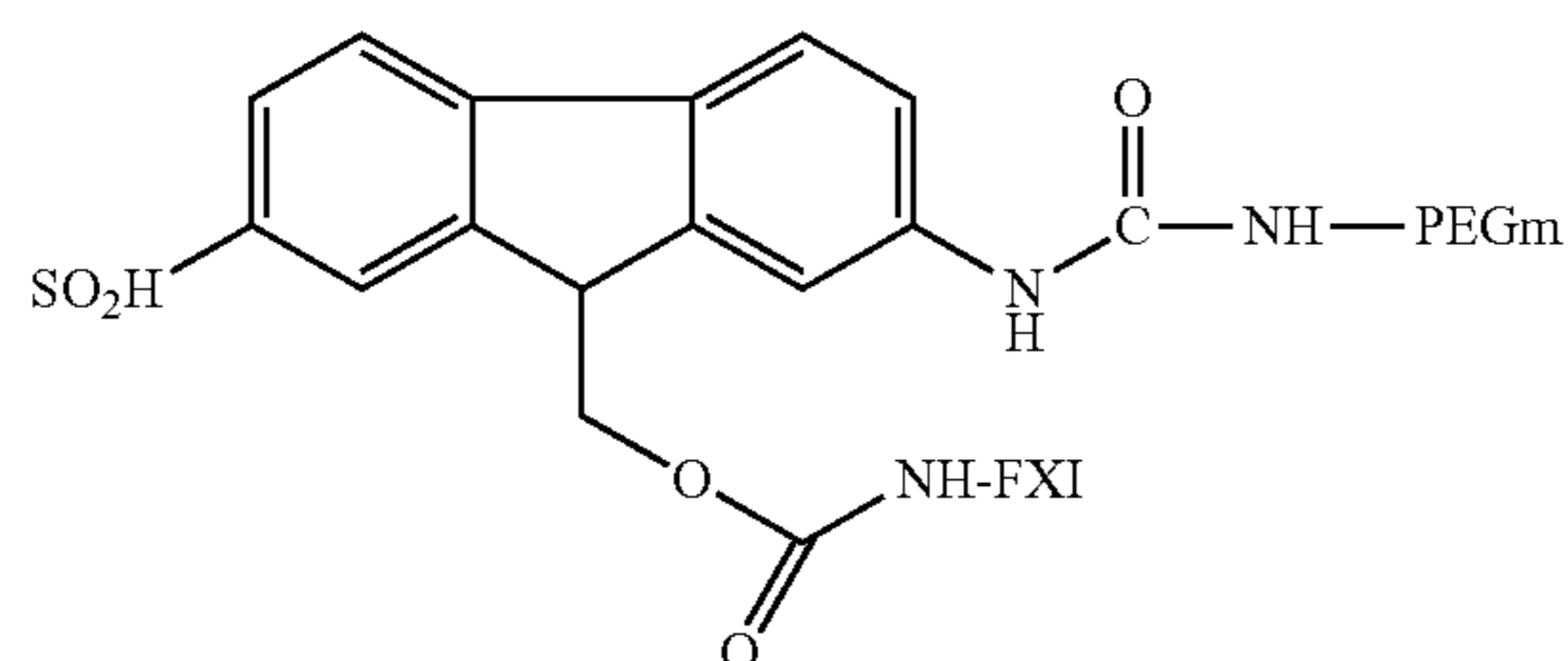
FXI Conjugate #4A
